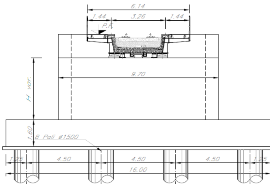
Figura 2 - Sezione trasversale spalla H=5.00 m
