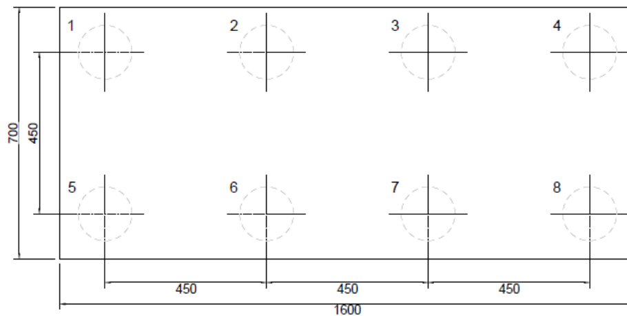
Figura 3 – Disposizione dei pali di fondazione
