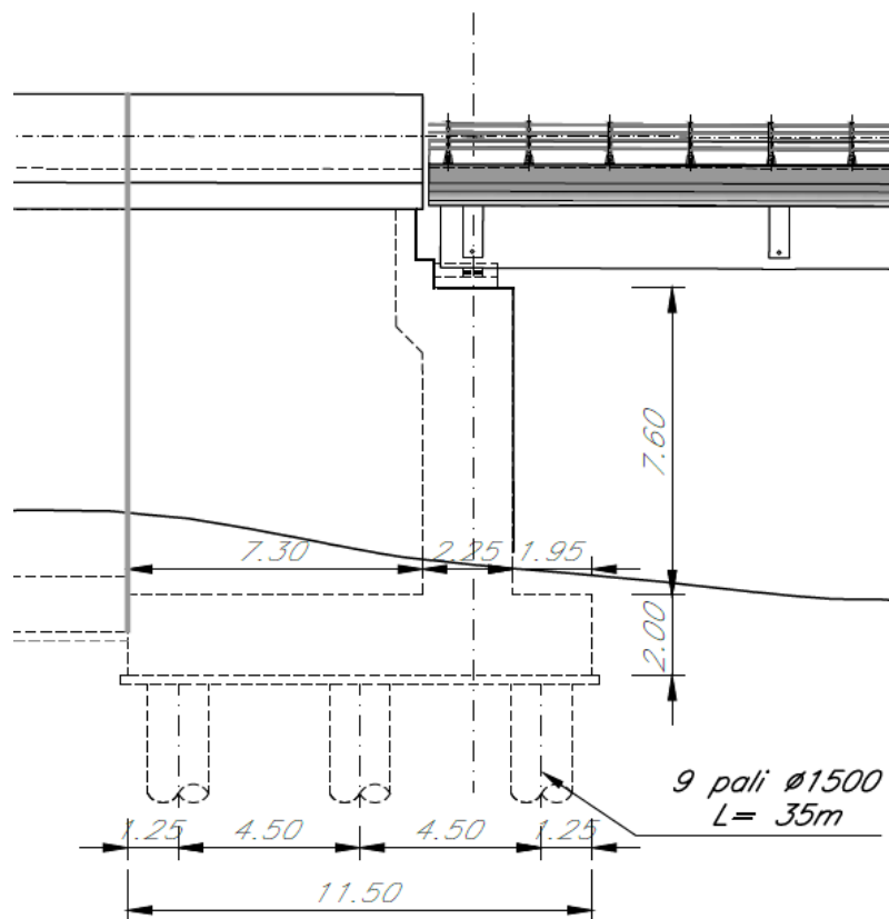
Figura 1 – Prospetto longitudinale spalla
