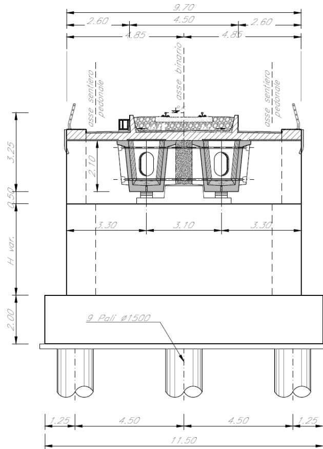
Figura 2 – Sezione trasversale spalla H=7.60 m
