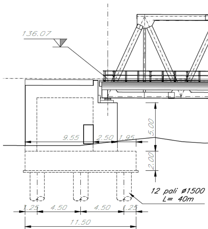
Figura 1 – Prospetto longitudinale spalla
