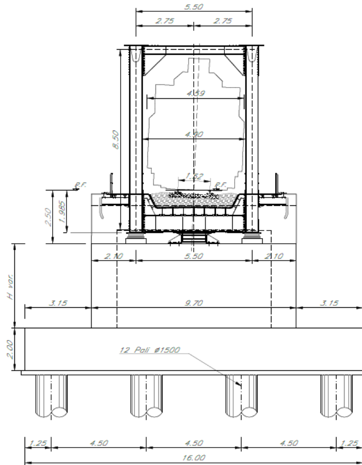
Figura 2 – Sezione trasversale spalla H=5.00 m
