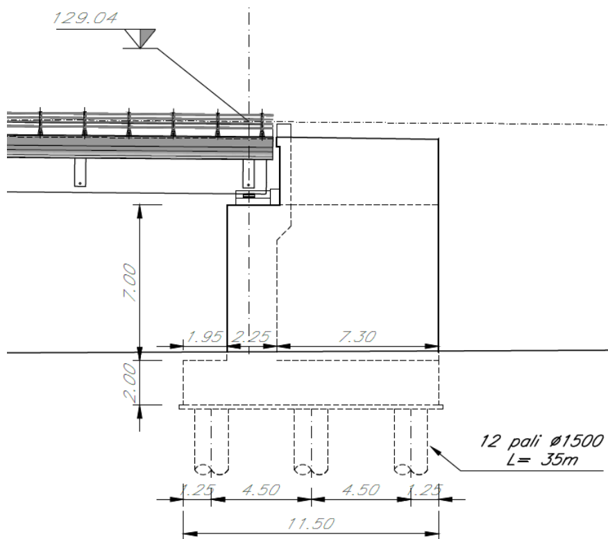
Figura 1 – Prospetto longitudinale spalla
