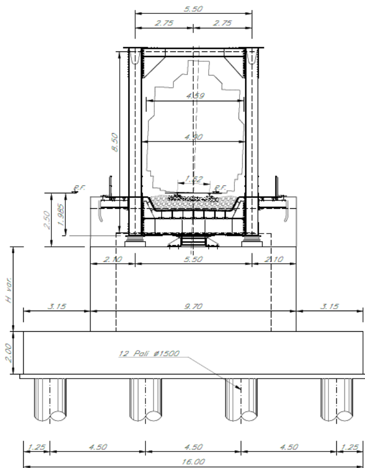
Figura 2 – Sezione trasversale spalla H=5.50 m
