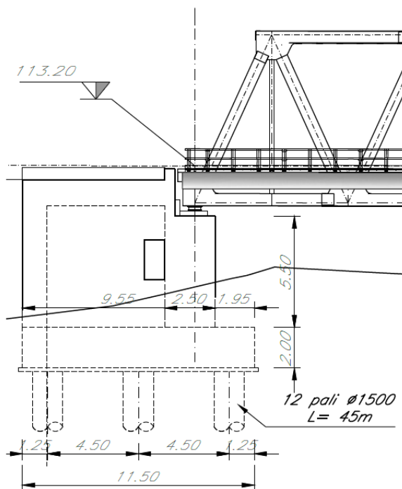
Figura 1 – Prospetto longitudinale spalla
