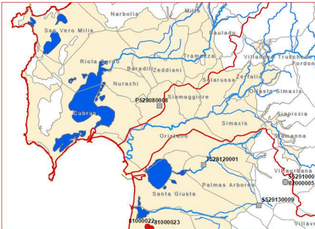
corpi idrici sotterranei degli acquiferi sedimentari plio-quadernari (fonte RAS PGDI)
