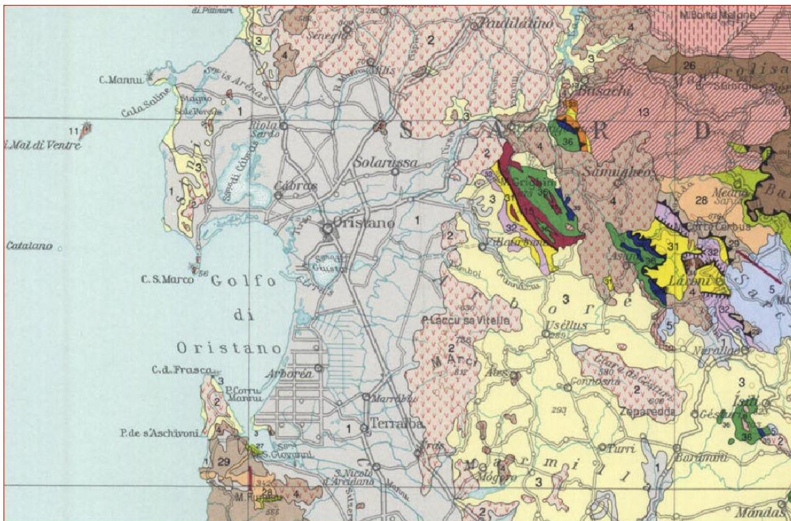
Stralcio Carta Tettonica d'Italia
