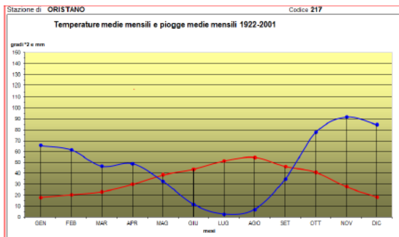
Fig. 4.4.7.1 - Grafico - Diagramma ombro termico per l'area di Oristano
