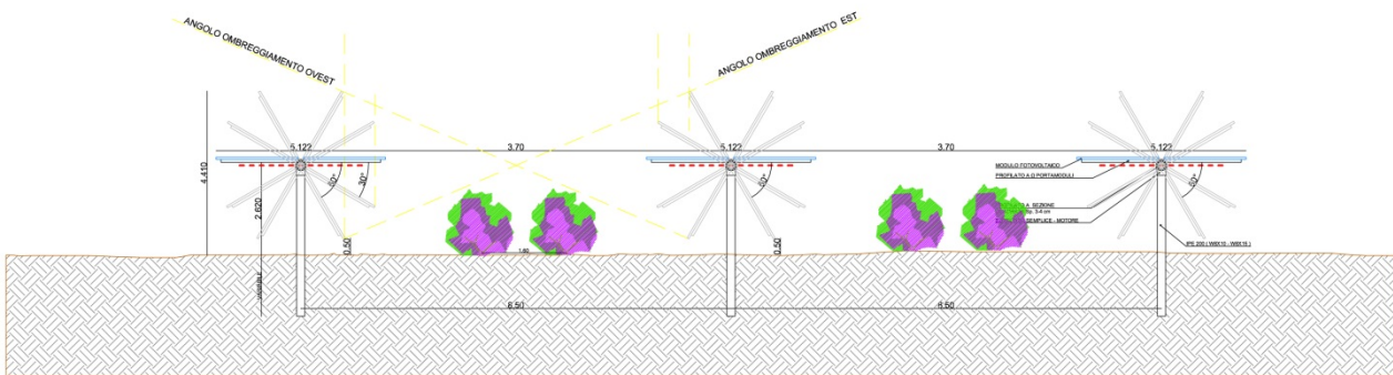
Struttura di sostegno tipo
