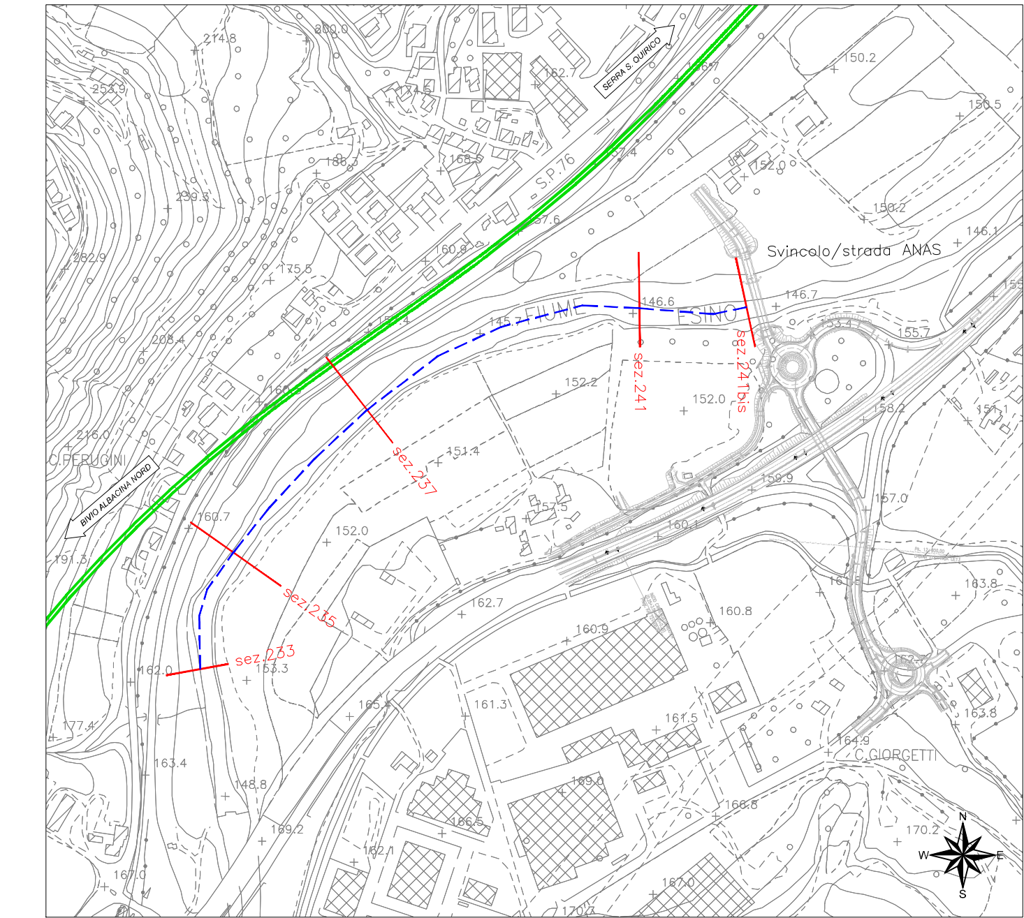
Planimetria (scala 1:5000) Tratto di parallelismo con il Fiume Esino (progr. 7+300 ÷ 7+700)
