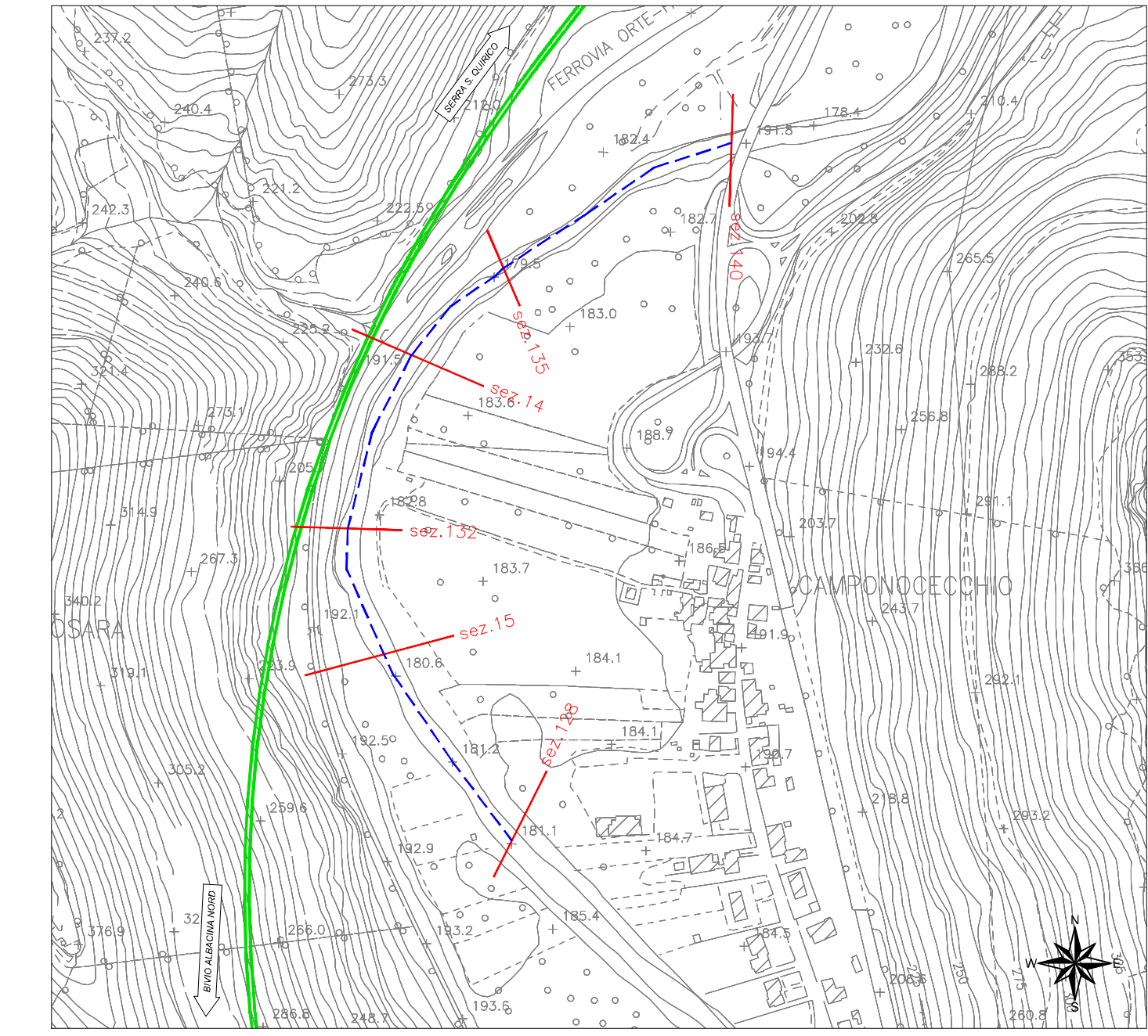
Planimetria (scala 1:5000) Tratto di parallelismo con il Fiume Esino (progr. 2+300 ÷ 2+600)
