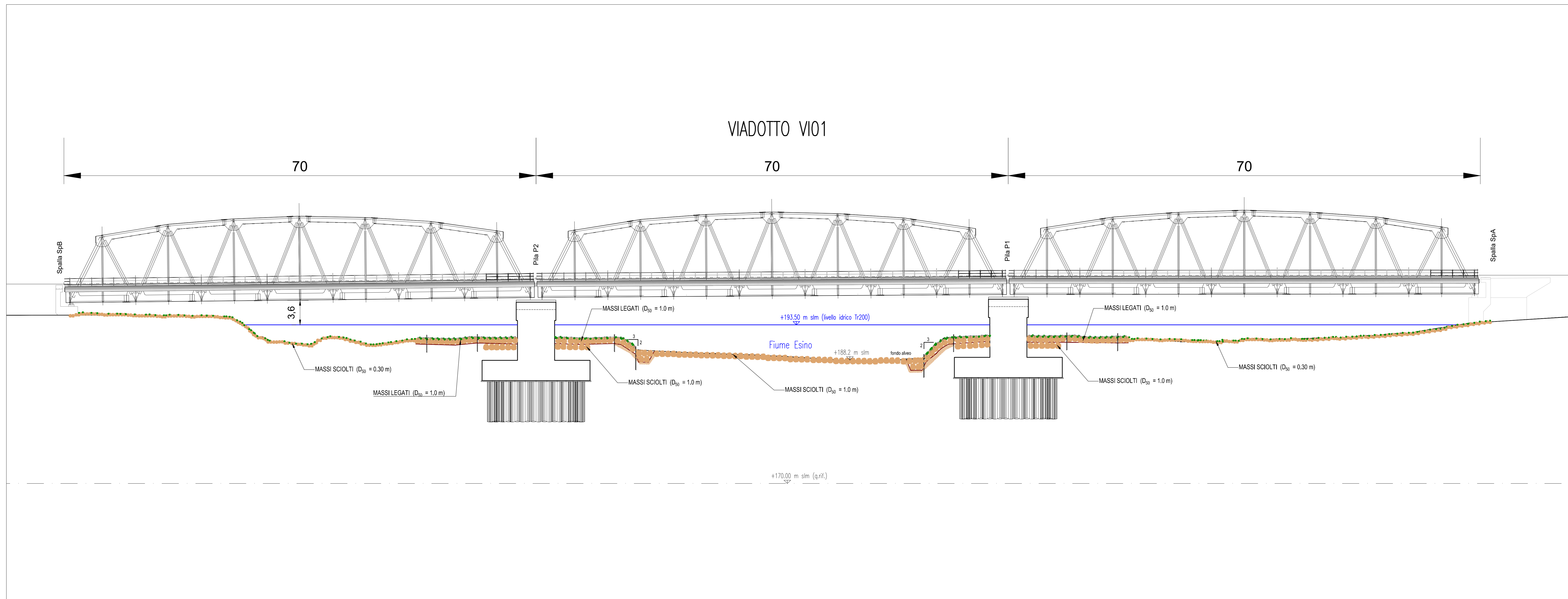
SEZIONE SISTEMAZIONE IDRAULICA - FIUME ESINO - VI01 - Scala 1:250
