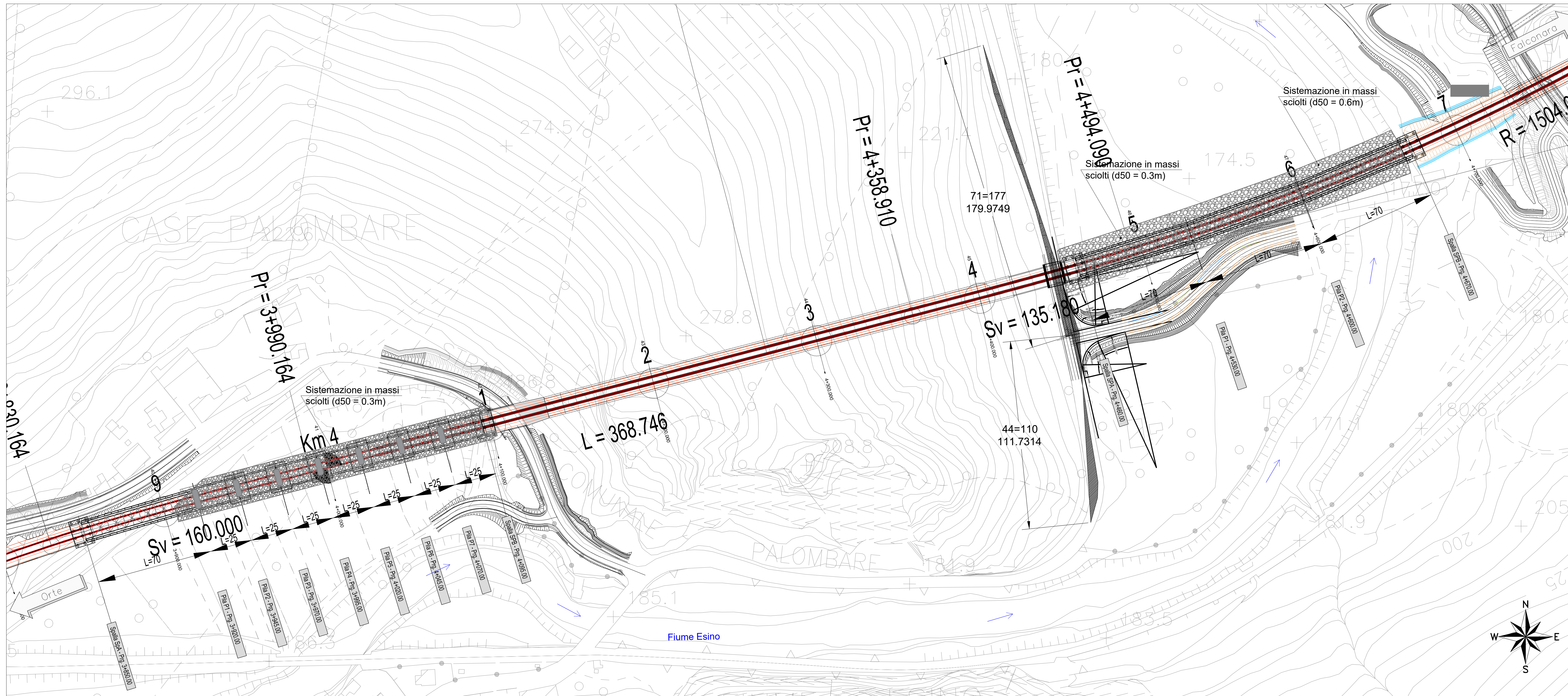
SEZIONE SISTEMAZIONE IDRAULICA - FIUME ESINO - VI02 - Scala 1:250
