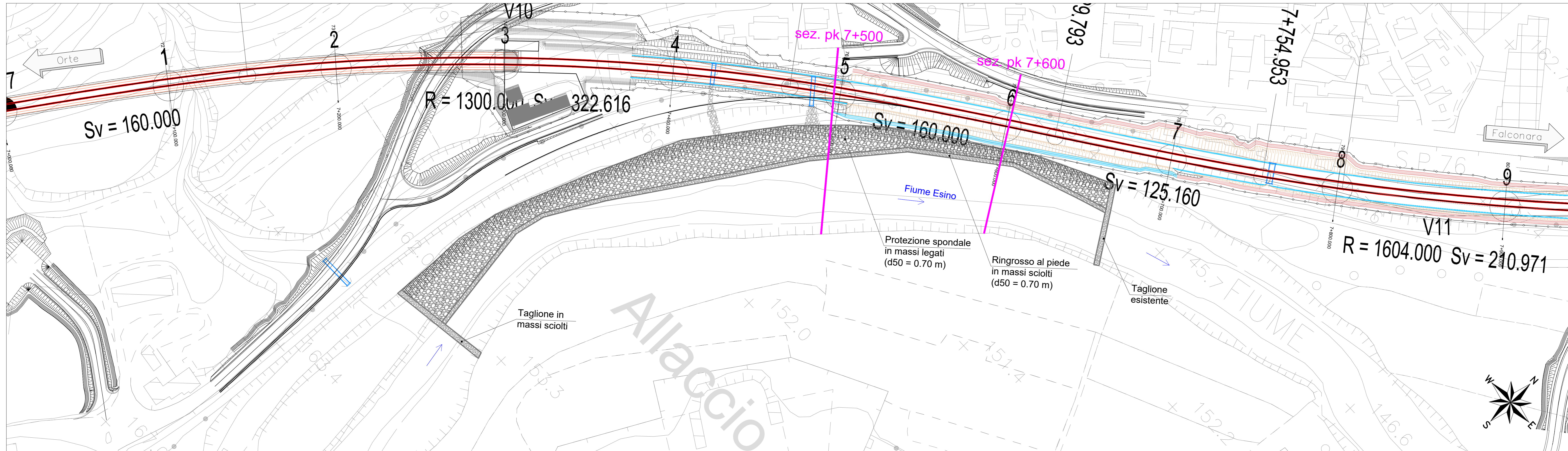
PLANIMETRIA SISTEMAZIONE IDRAULICA - AFFIANCAMENTO AL FIUME ESINO - TRATTO PROGR. 7+300 E 7+700 - Scala 1:1000
