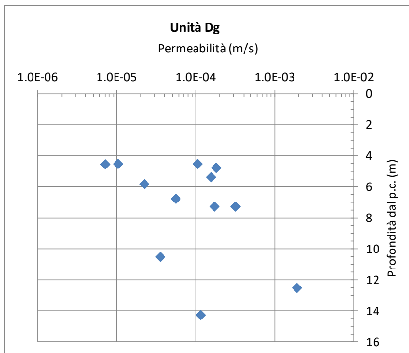
figura 10.17: Risultati prove di permeabilità
