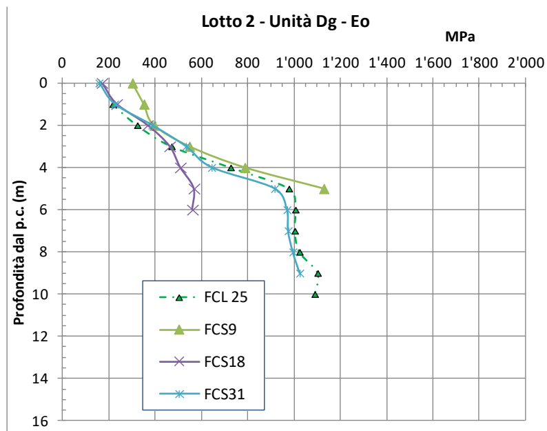
figura 10.23: Lotto 2 – Prove DH - Andamento di E_0 con la profondità
