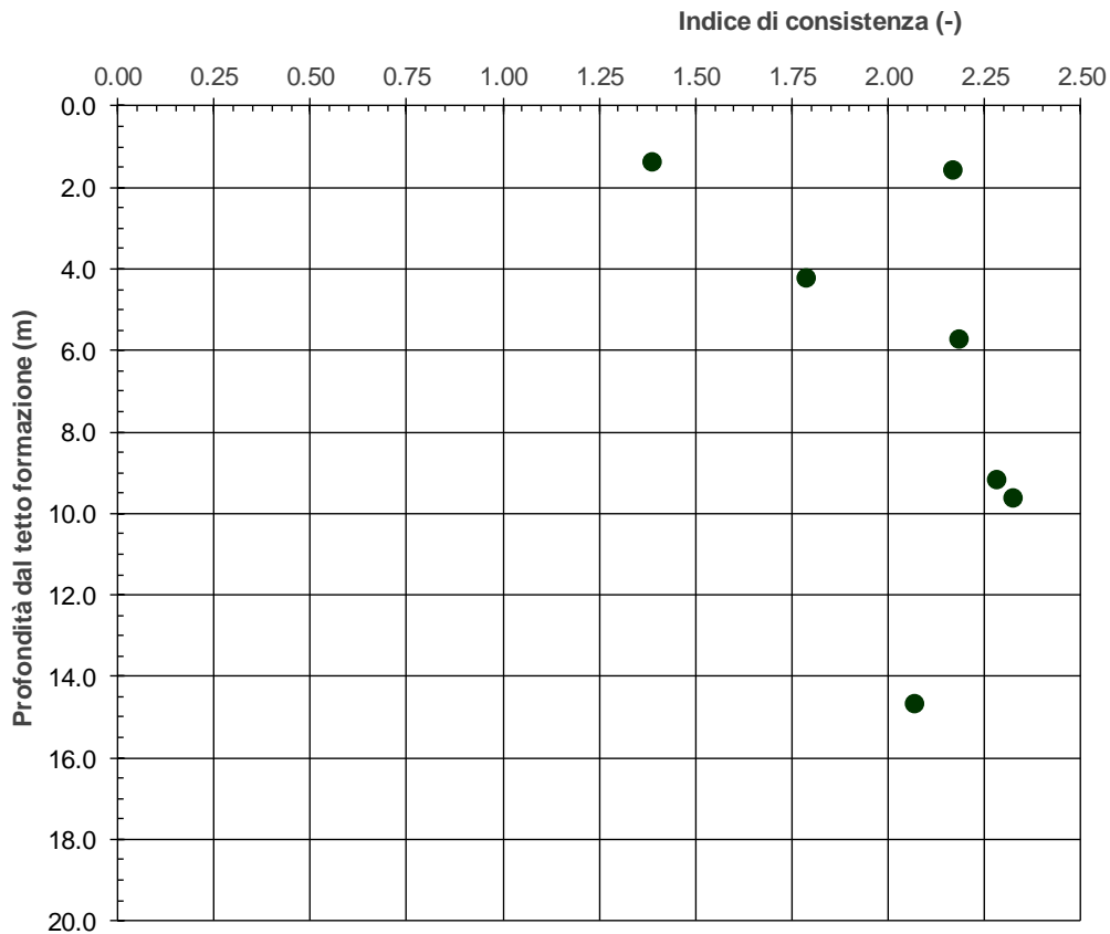
figura 13.4: Indice di consistenza in funzione della profondità
