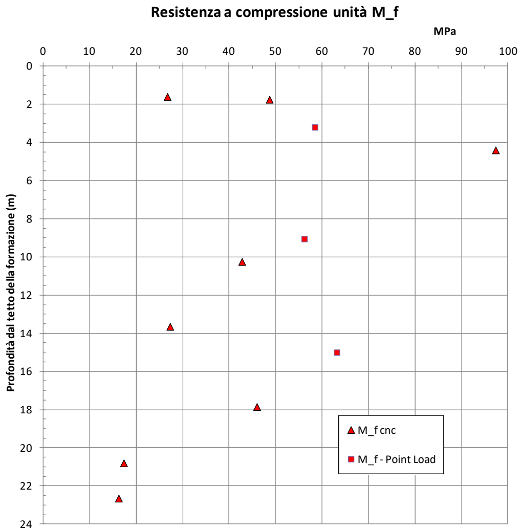
figura 12.4: Resistenza a compressione unità M_f
