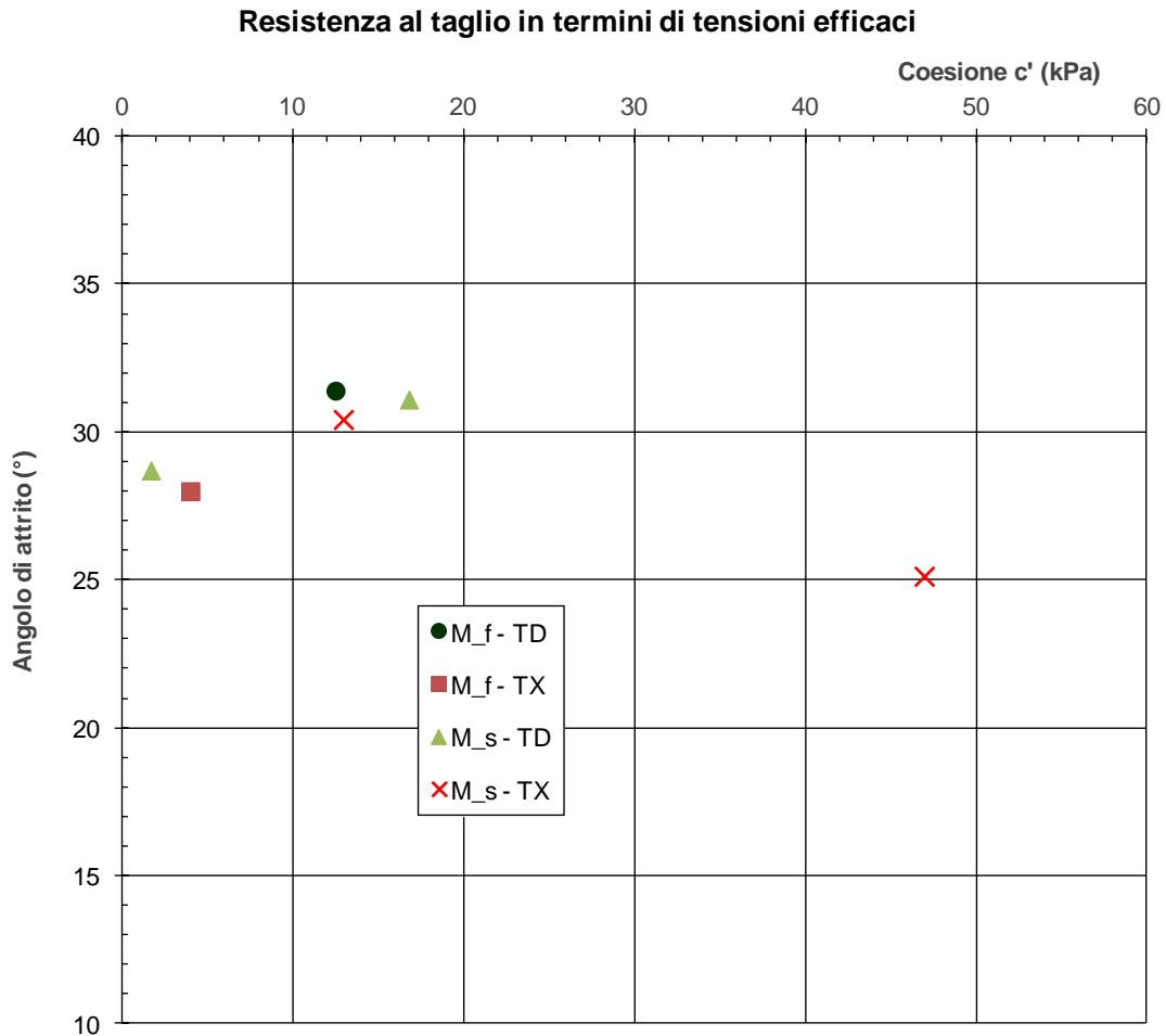
figura 13.8: Resistenza al taglio in termini di sforzi efficaci \phi' e c'
