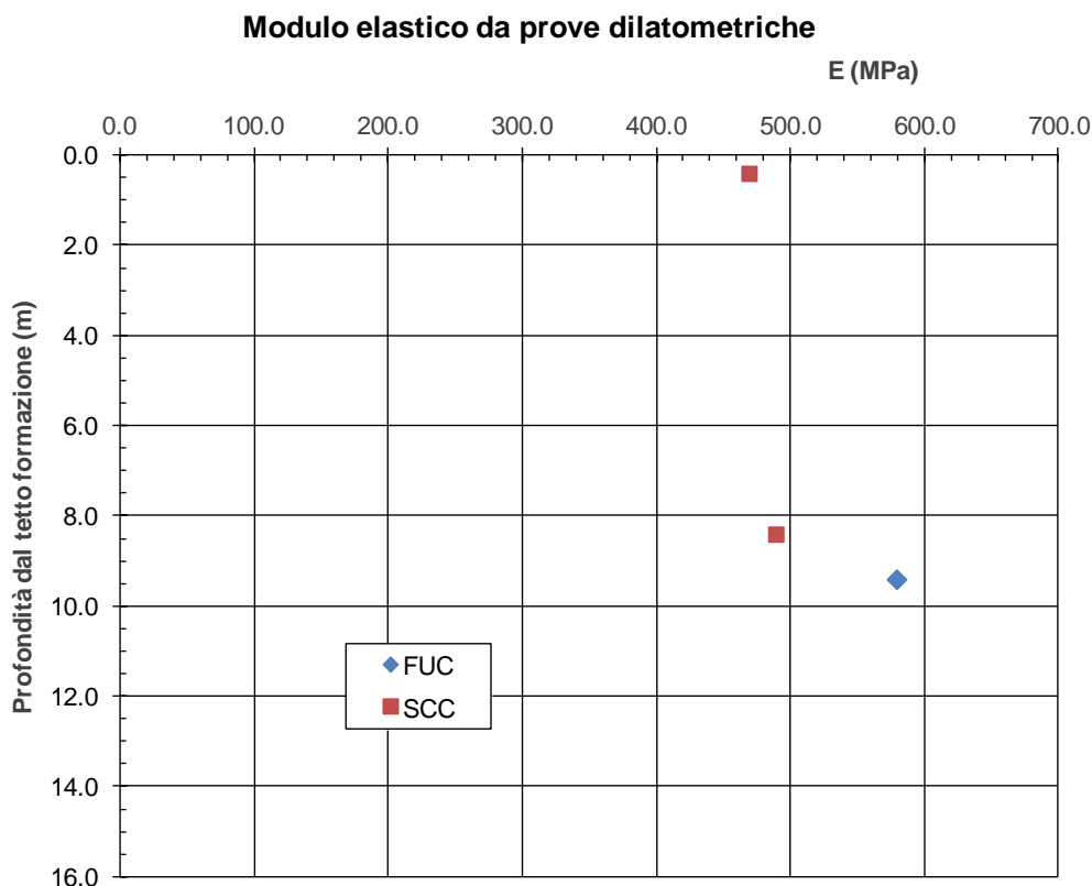
figura 13.10: Modulo elastico da prova dilatometrica
