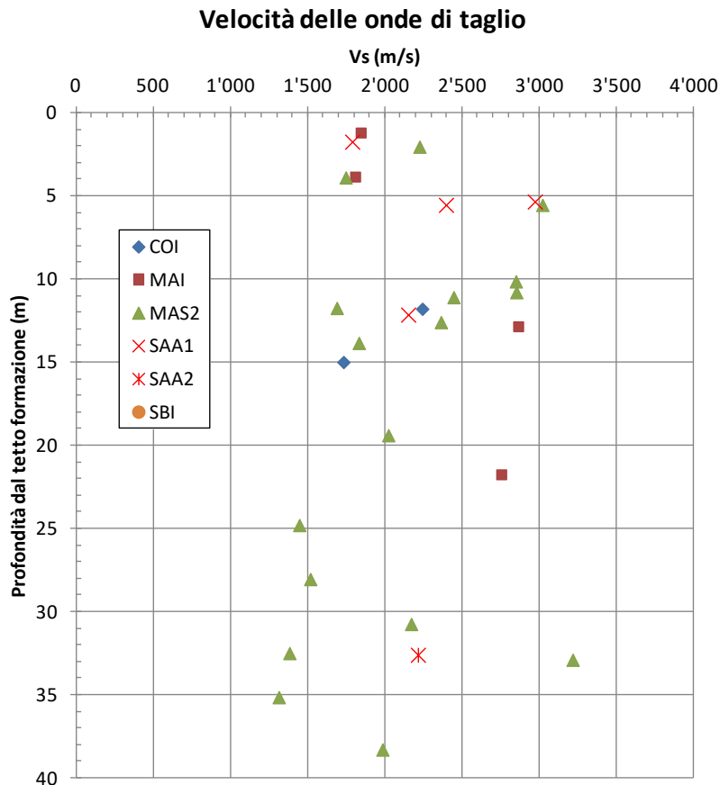
figura 11.9: Velocità delle onde V_s suddivise per formazione geologica
