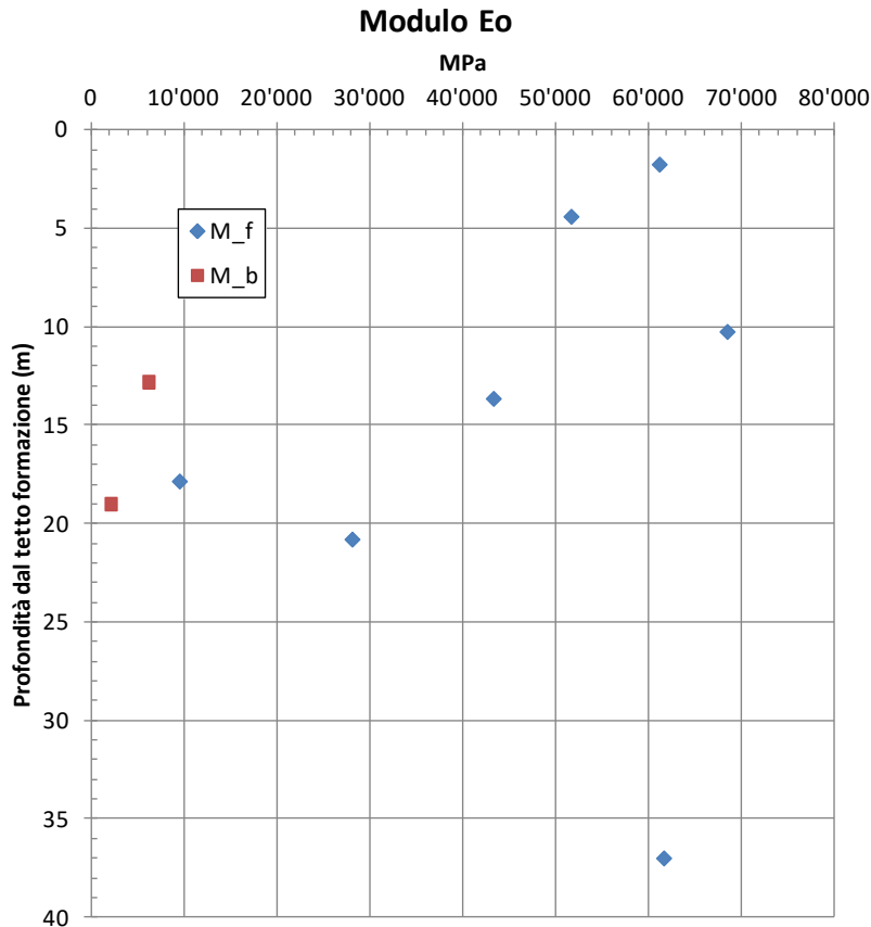
figura 12.12: Modulo elastico E 0 - unità geotecnica M f
