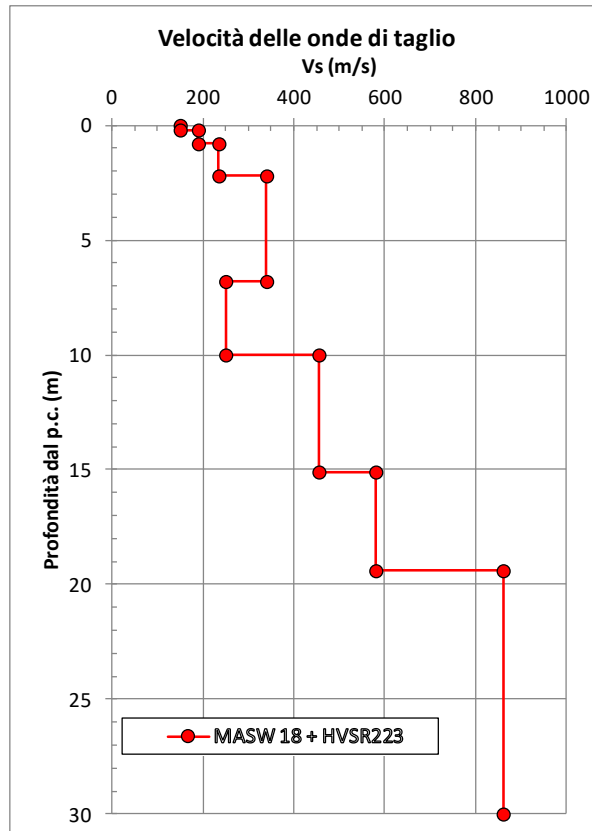
figura 15.6: MASW18 - Velocità delle onde di taglio con la profondità
