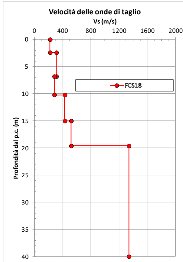
figura 15.7: DH FCS18 - Velocità delle onde di taglio con la profondità
