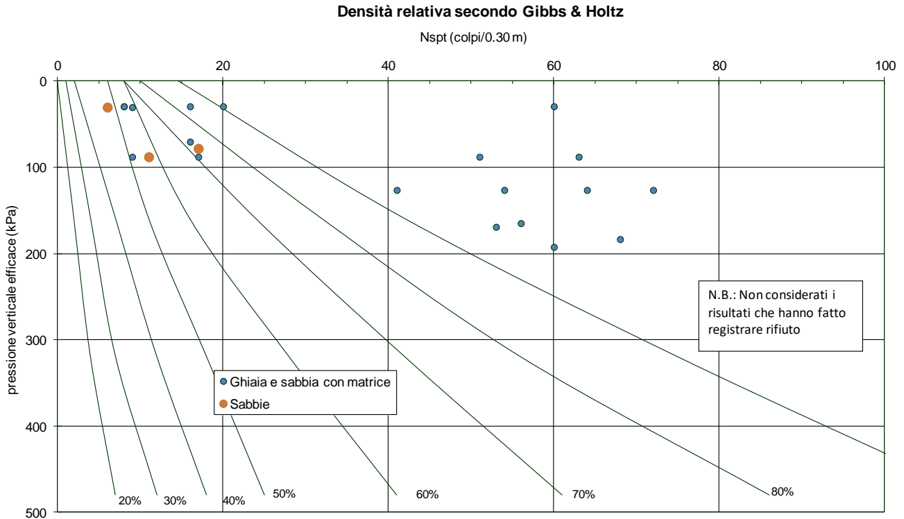
figura 10.21: Relazione N_{SPT} - Densità relativa (Gibbs&Holtz 1959)
