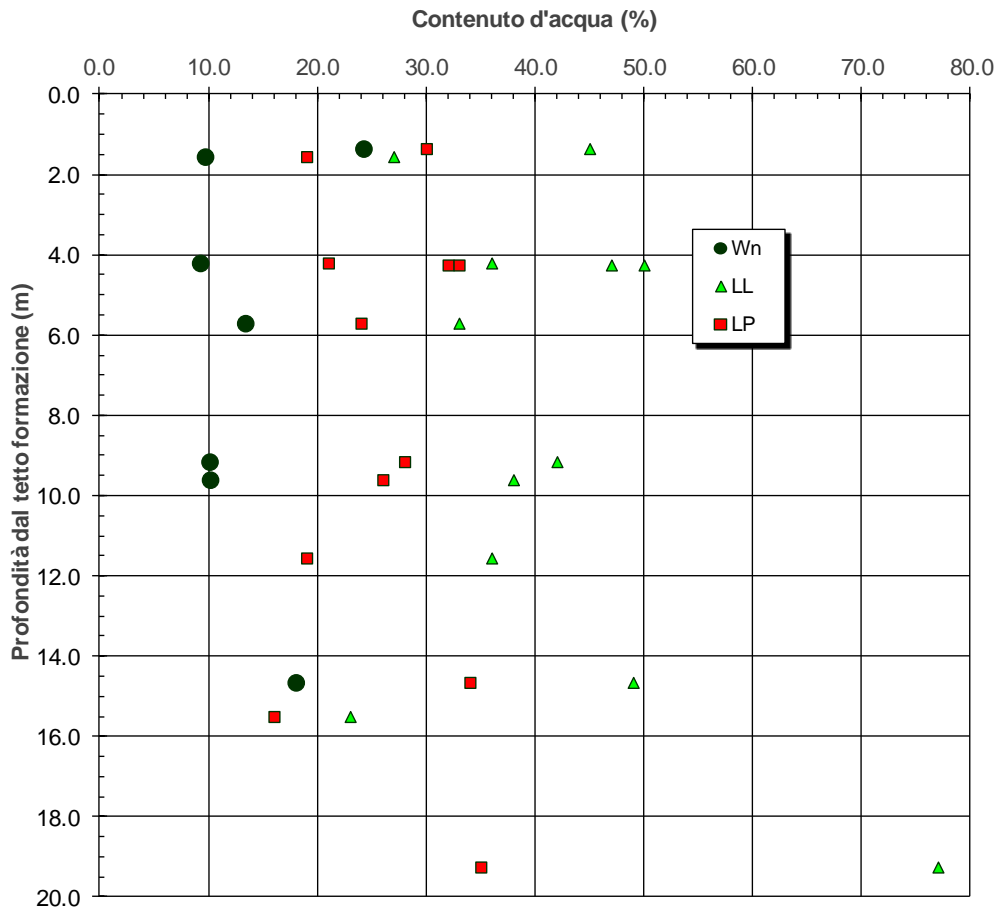
figura 13.3: Limiti di Atterberg e umidità naturale in funzione della profondità
