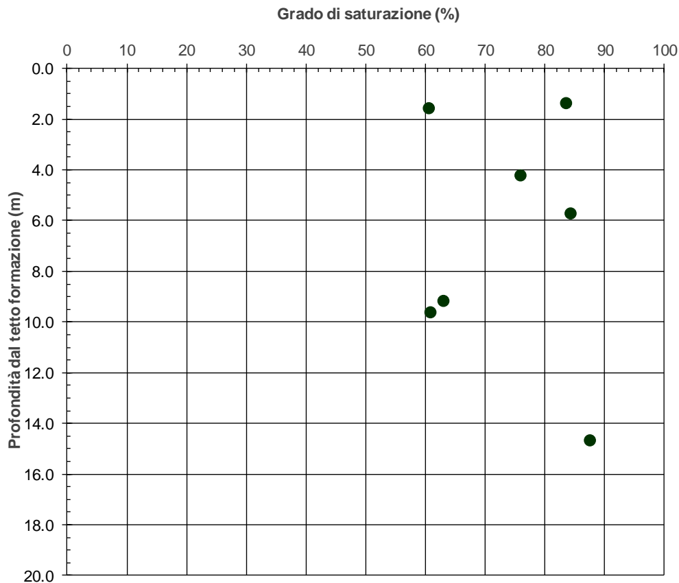
figura 13.5: Grado di saturazione in funzione della profondità
