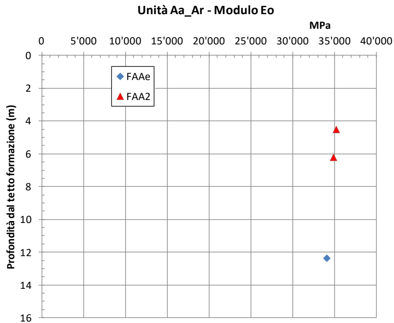
figura 14.19: Modulo E_0
