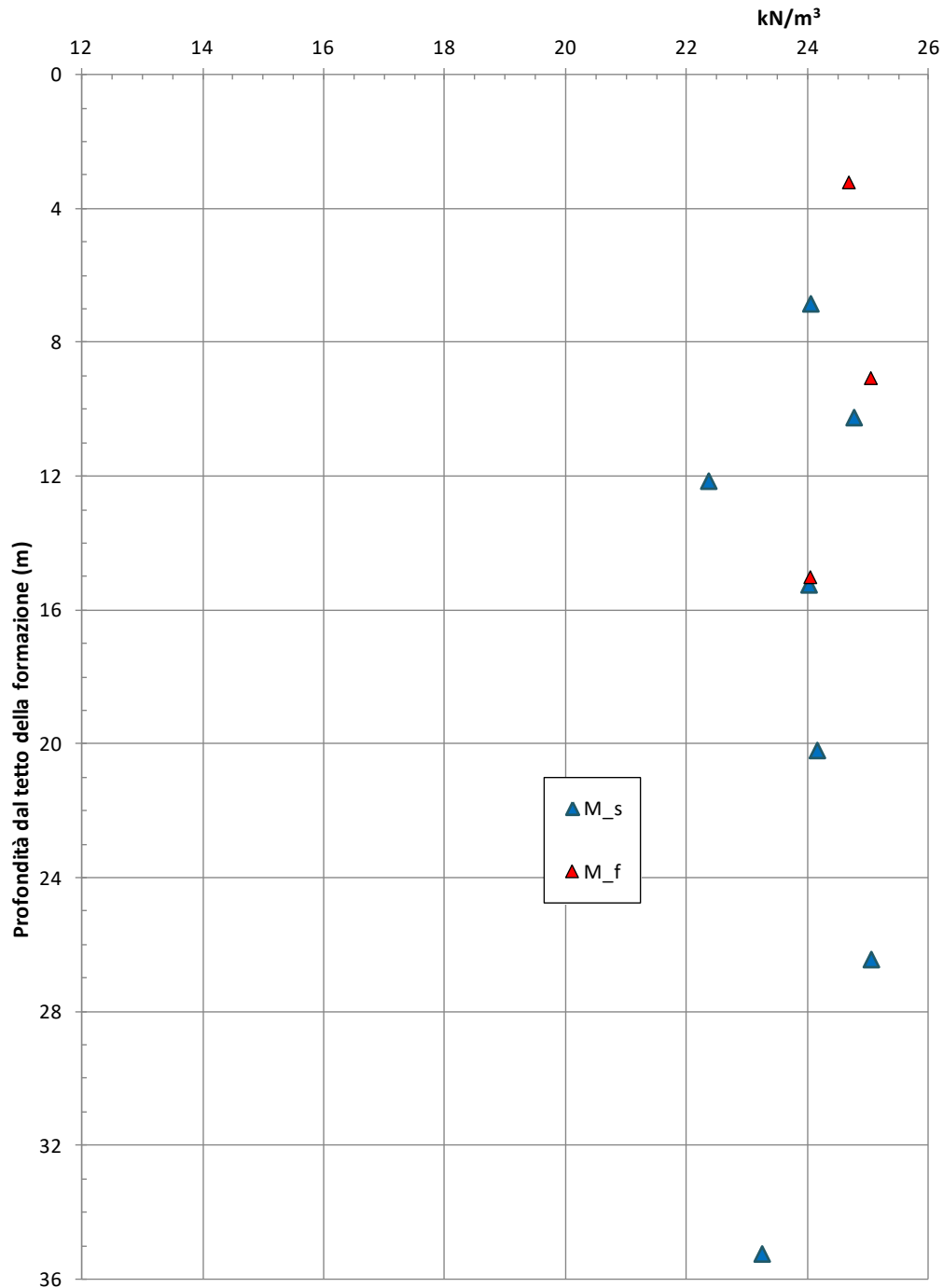
figura 12.1: Peso di volume per le diverse unità geotecniche
