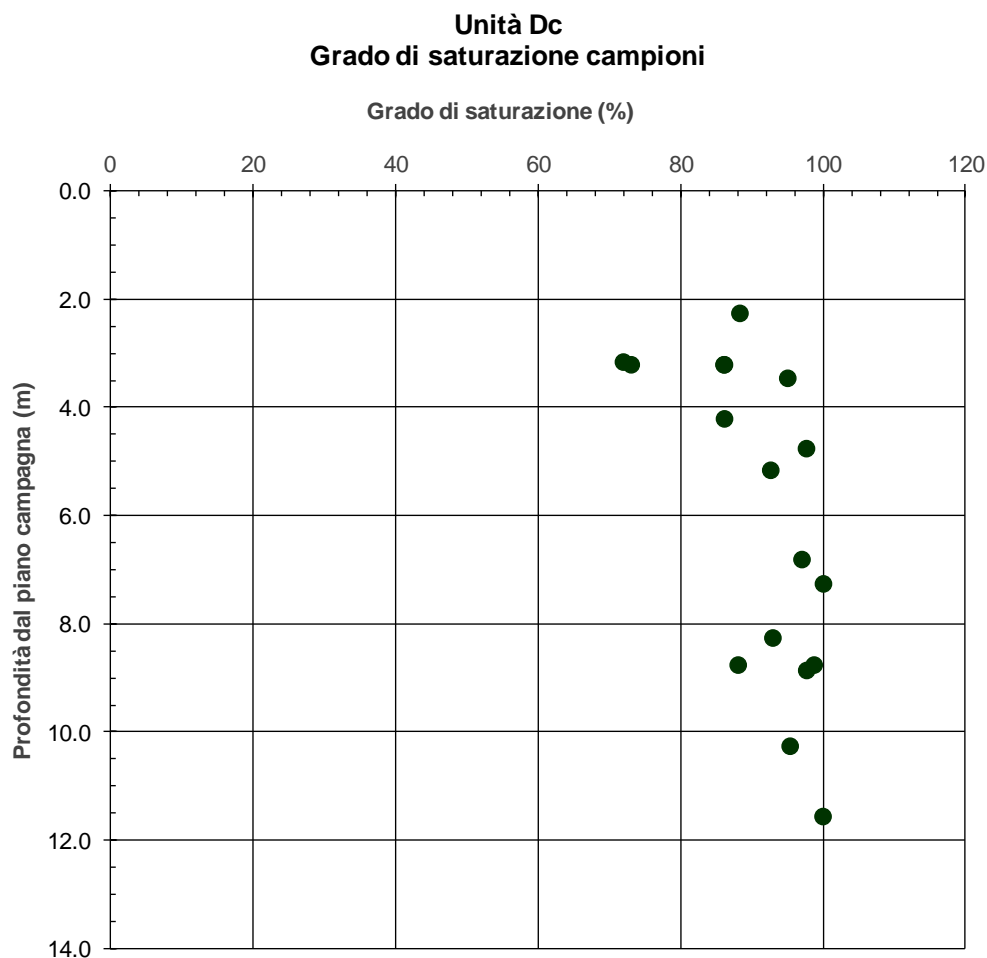
figura 10.6: Grado di saturazione in funzione della profondità
