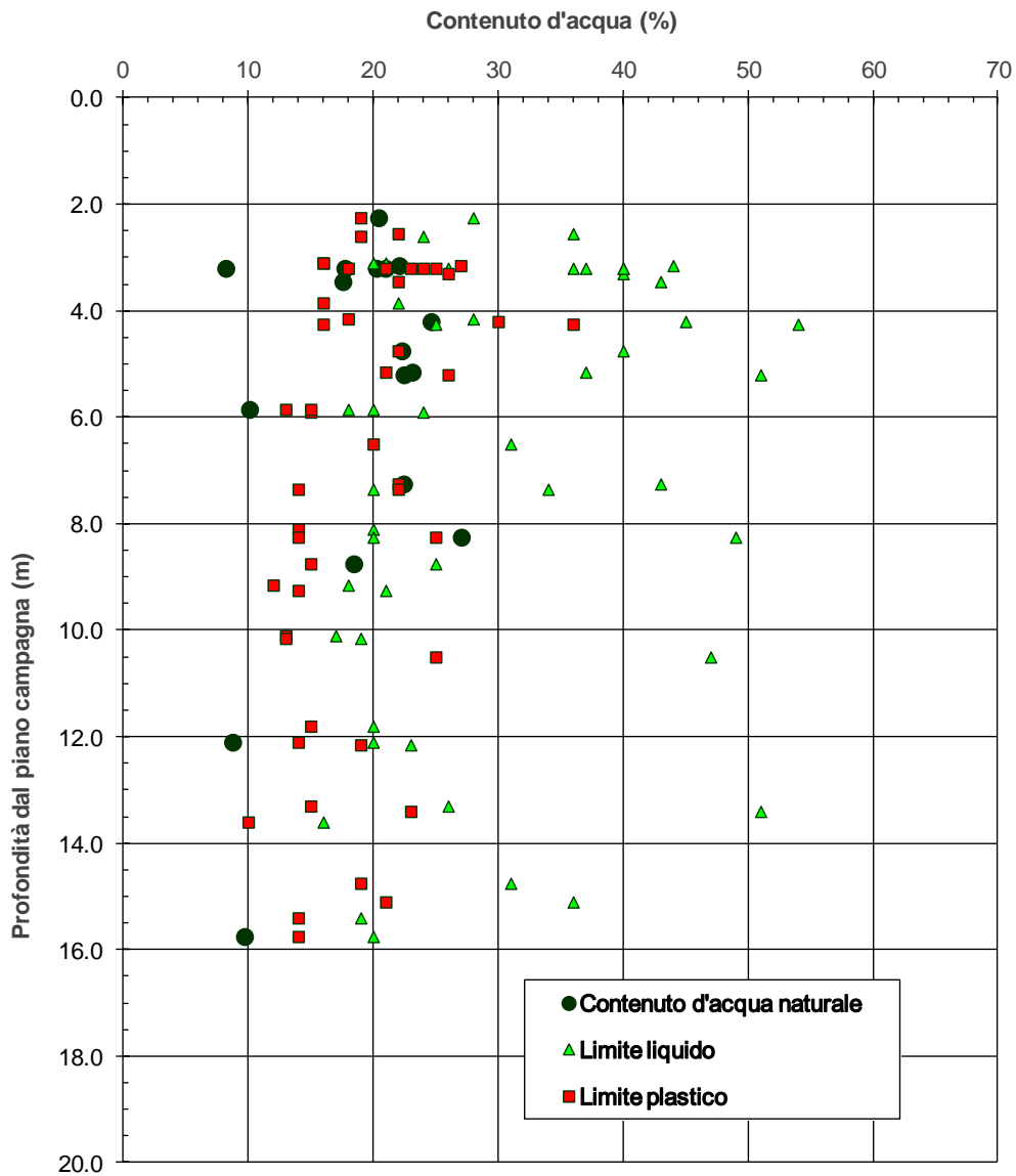
figura 10.2: Limiti di Atterberg e umidità naturale in funzione della profondità
