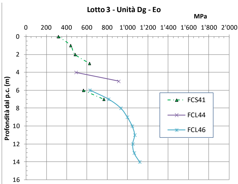
figura 10.24: Lotto 3 – Prove DH - Andamento di E_0 con la profondità
