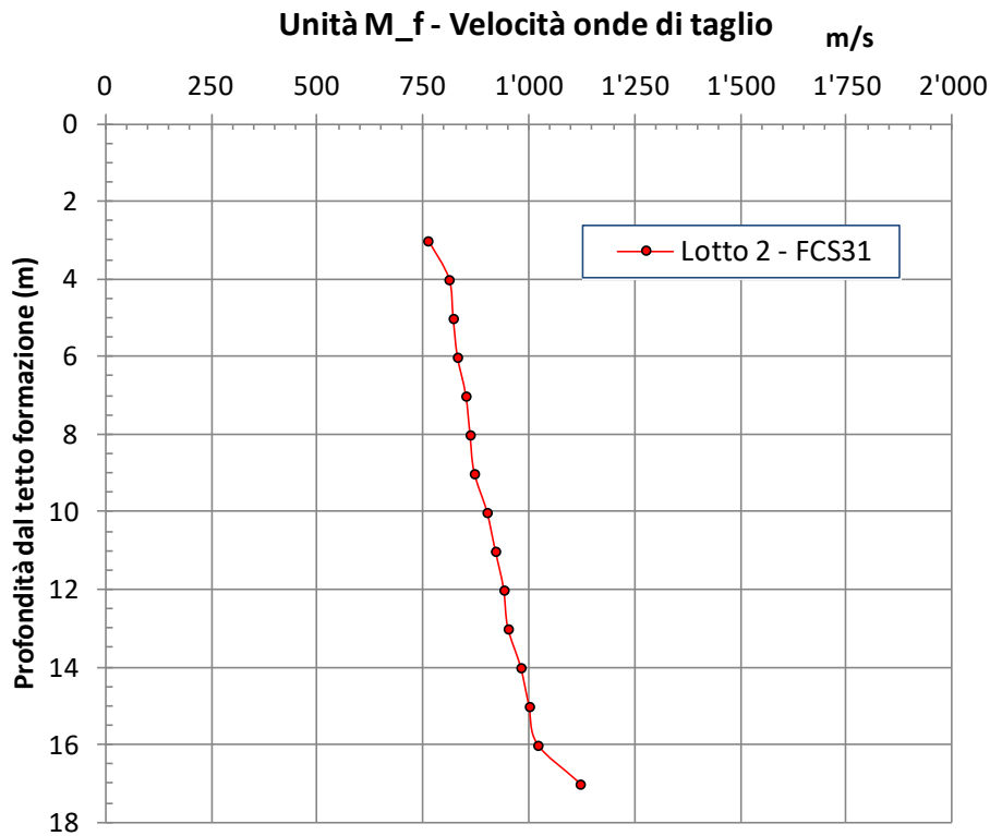
figura 12.13: Velocità delle onde di taglio - unità geotecnica M f
