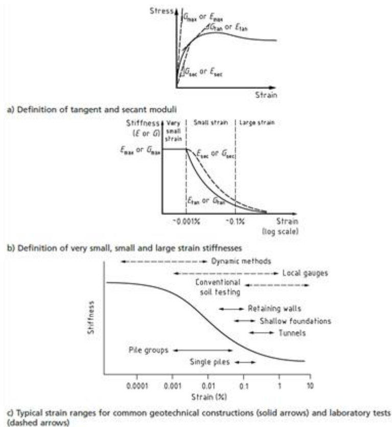
Figura 6-1 – Parametri di rigidezza per il terreno in dipendenza del livello deformativo
