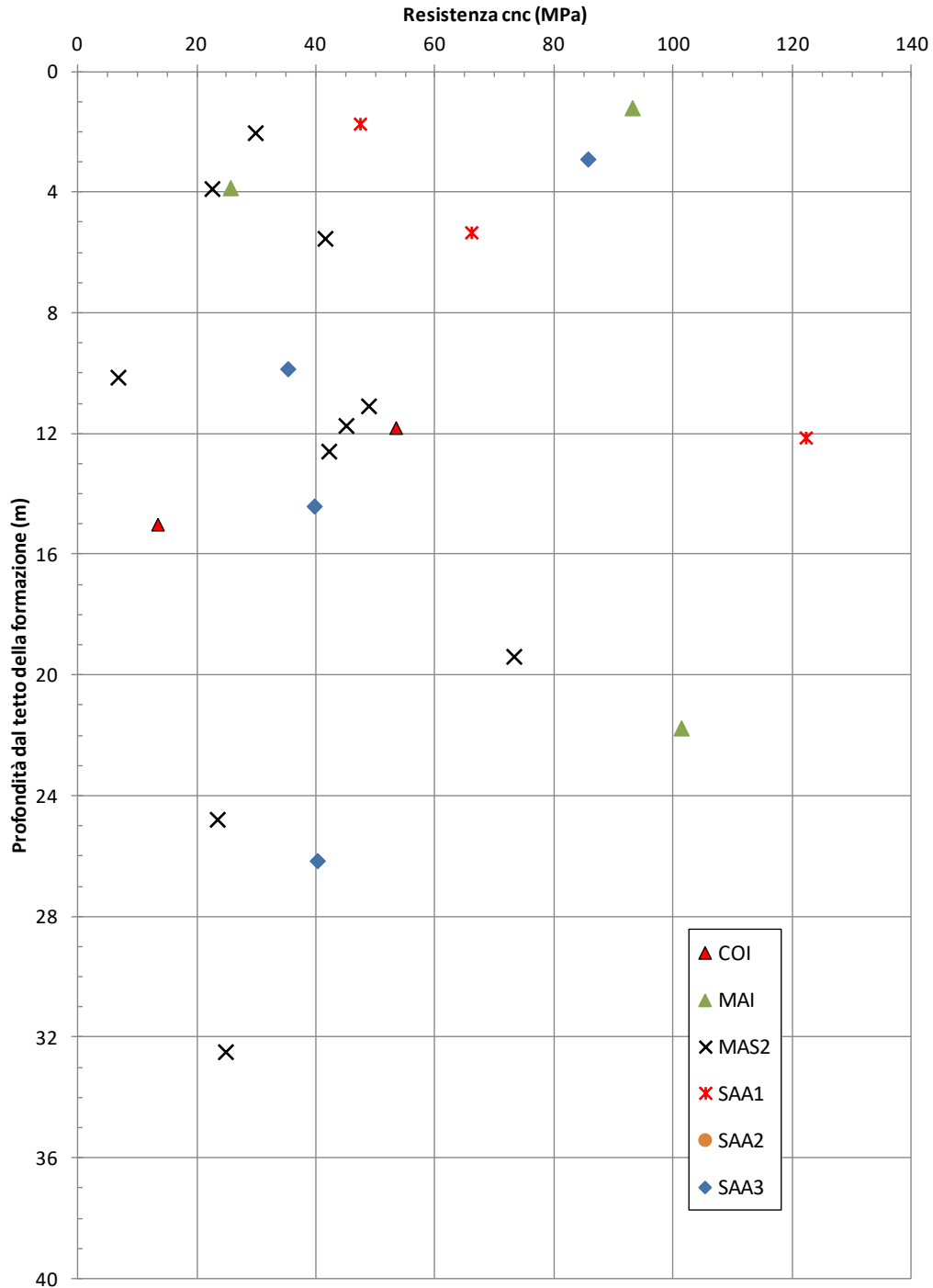
figura 11.3: Resistenza a compressione materiali calcarei per formazione
