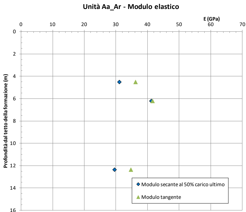
figura 14.15: Modulo elastico E_i livelli arenacei
