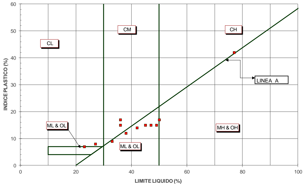
figura 13.1: Carta di plasticità marne alterate
