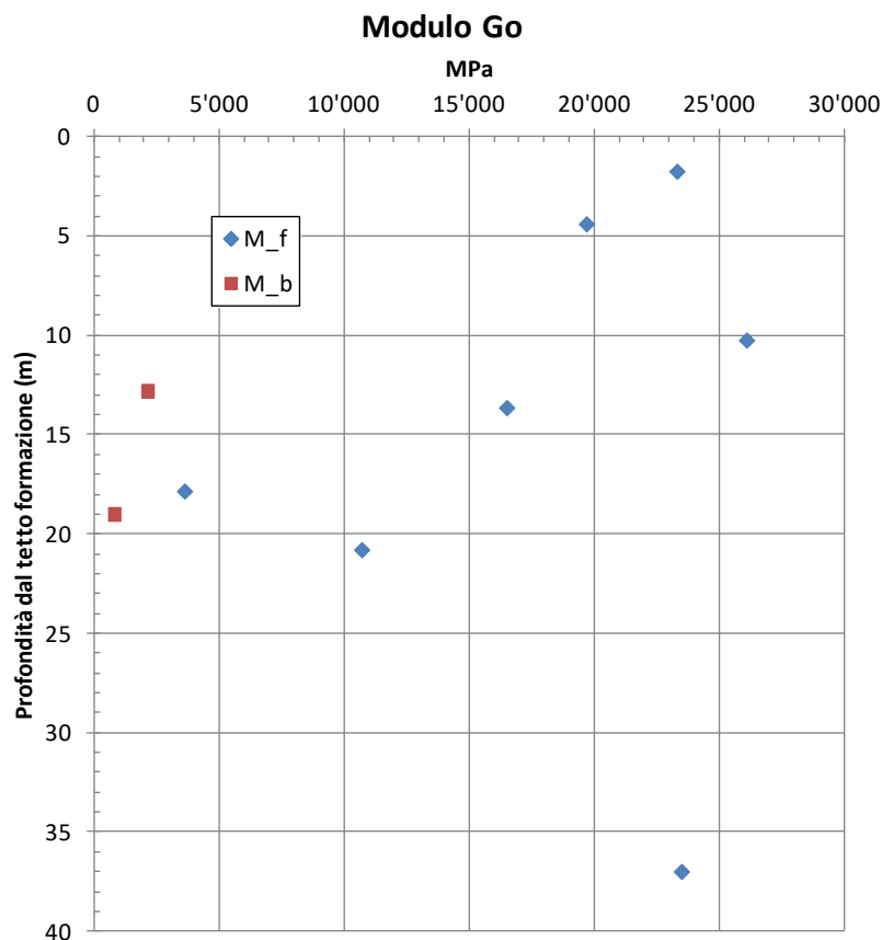
figura 12.11: Modulo di taglio G_0 - unità geotecnica M_f
