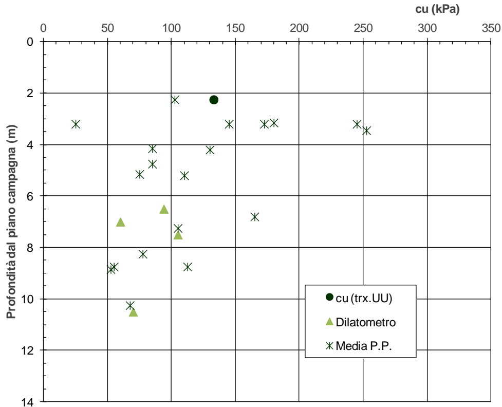
figura 10.11: Resistenza al taglio in condizioni non drenate
