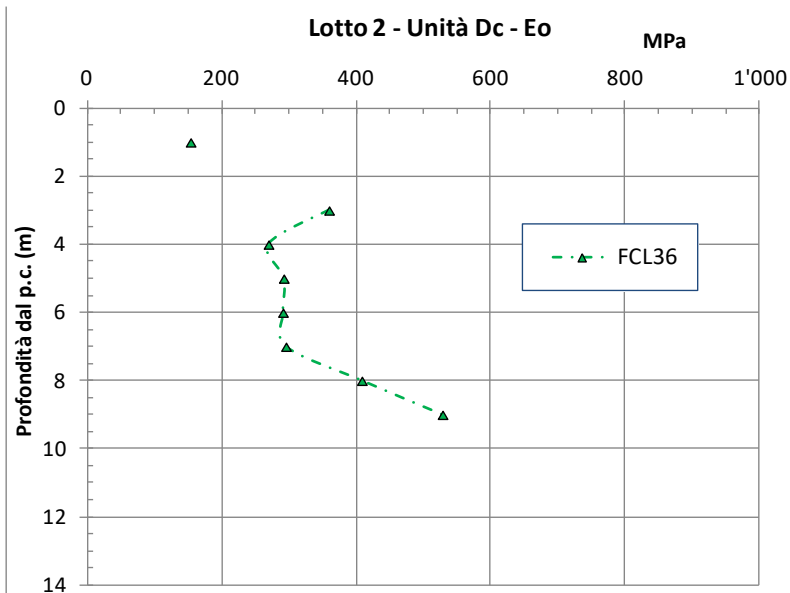
figura 10.14: Modulo Eo a piccole deformazioni – Lotto 2
