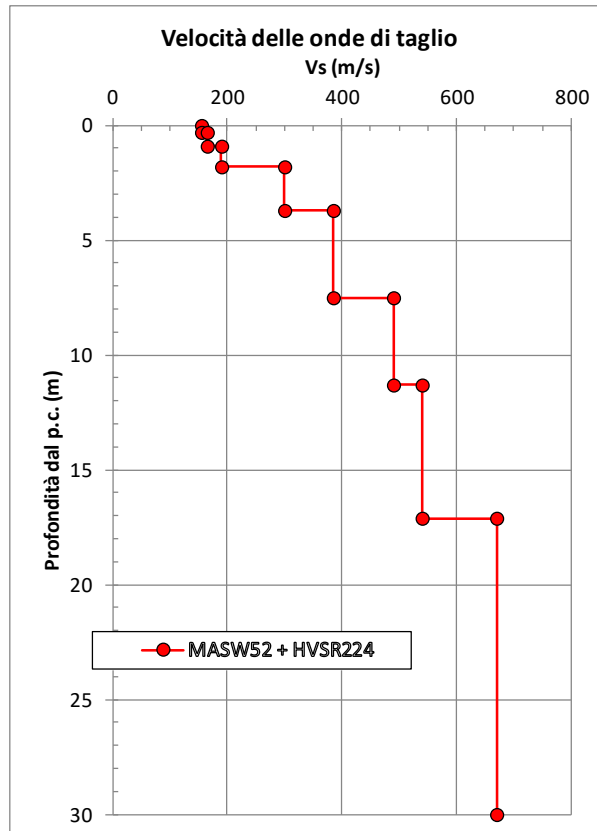
figura 15.5: MASW52 - Velocità delle onde di taglio con la profondità
