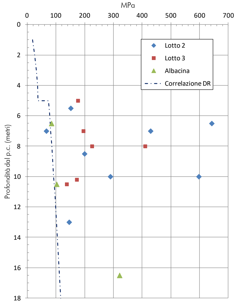
figura 10.28: Modulo elastico da prove dilatometriche
