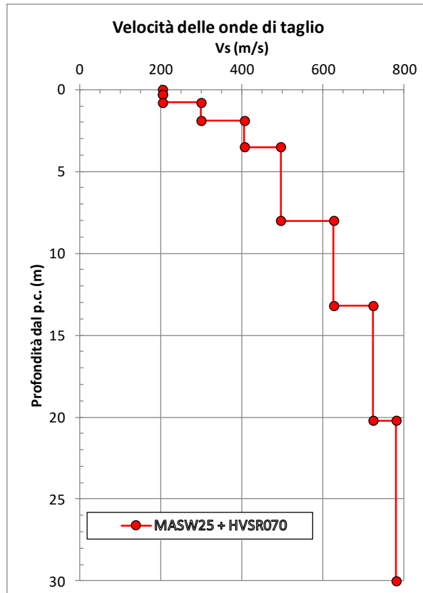
figura 15.8: MASW25 - Velocità delle onde di taglio con la profondità
