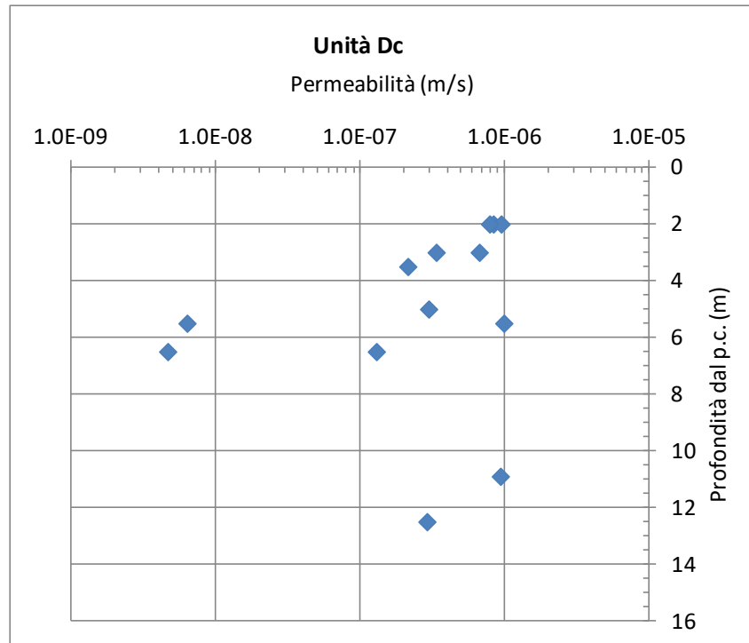
figura 10.7: Risultati prove di permeabilità
