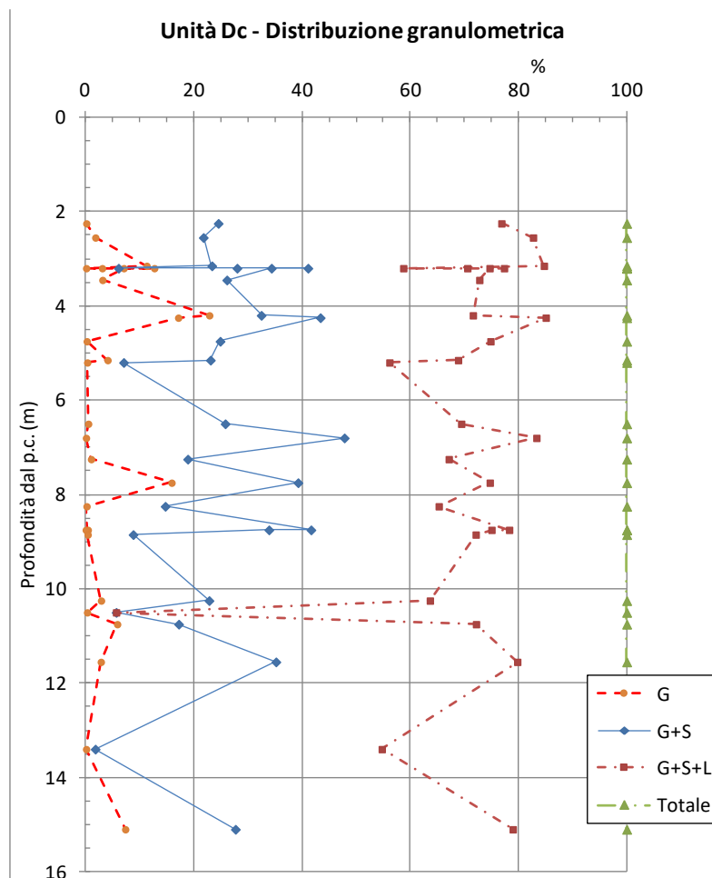
figura 10.3: Distribuzione granulometrica in funzione della profondità
