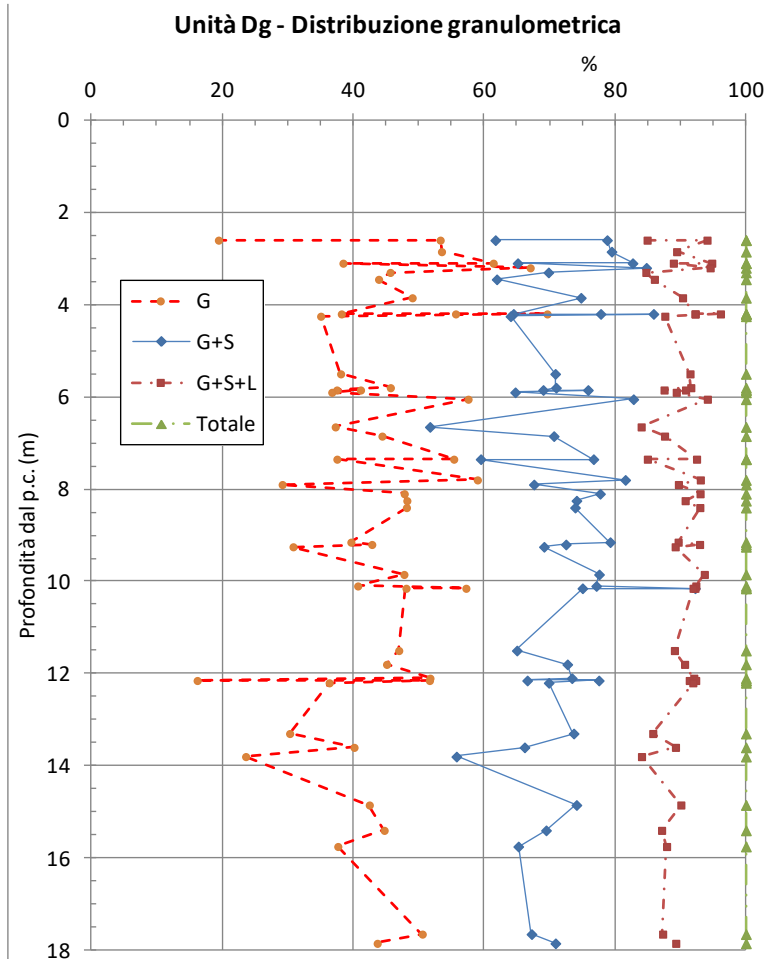
figura 10.16: Distribuzione granulometrica in funzione della profondità
