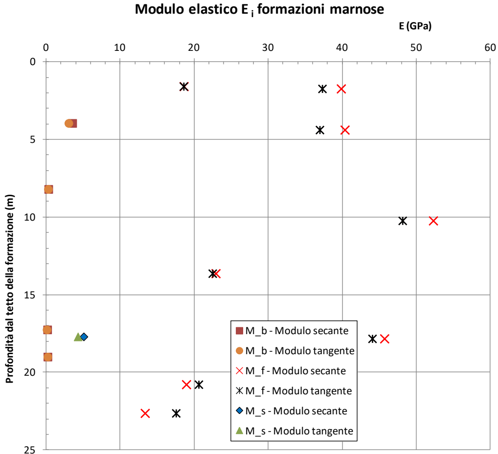
figura 12.8: Modulo elastico E_i formazioni marnose
