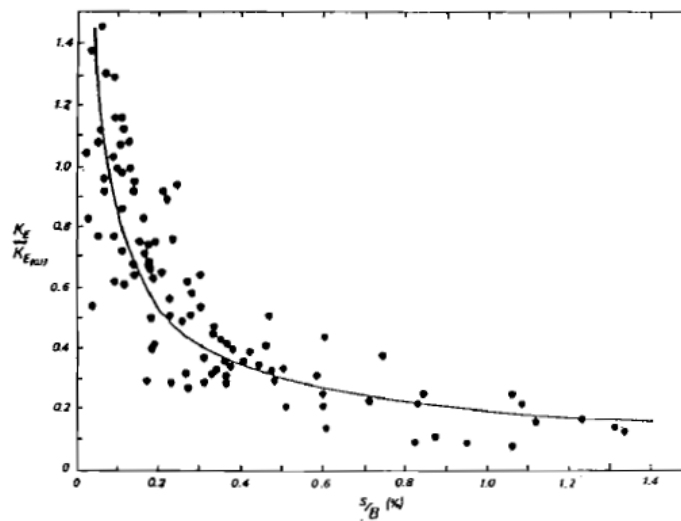
figura 7.3: Decadimento del numero del modulo normalizzato
