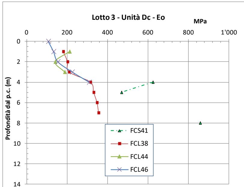
figura 10.15: Modulo Eo a piccole deformazioni – Lotto 3
