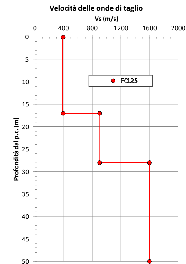
figura 15.9: DH FCL25 - Velocità delle onde di taglio con la profondità
