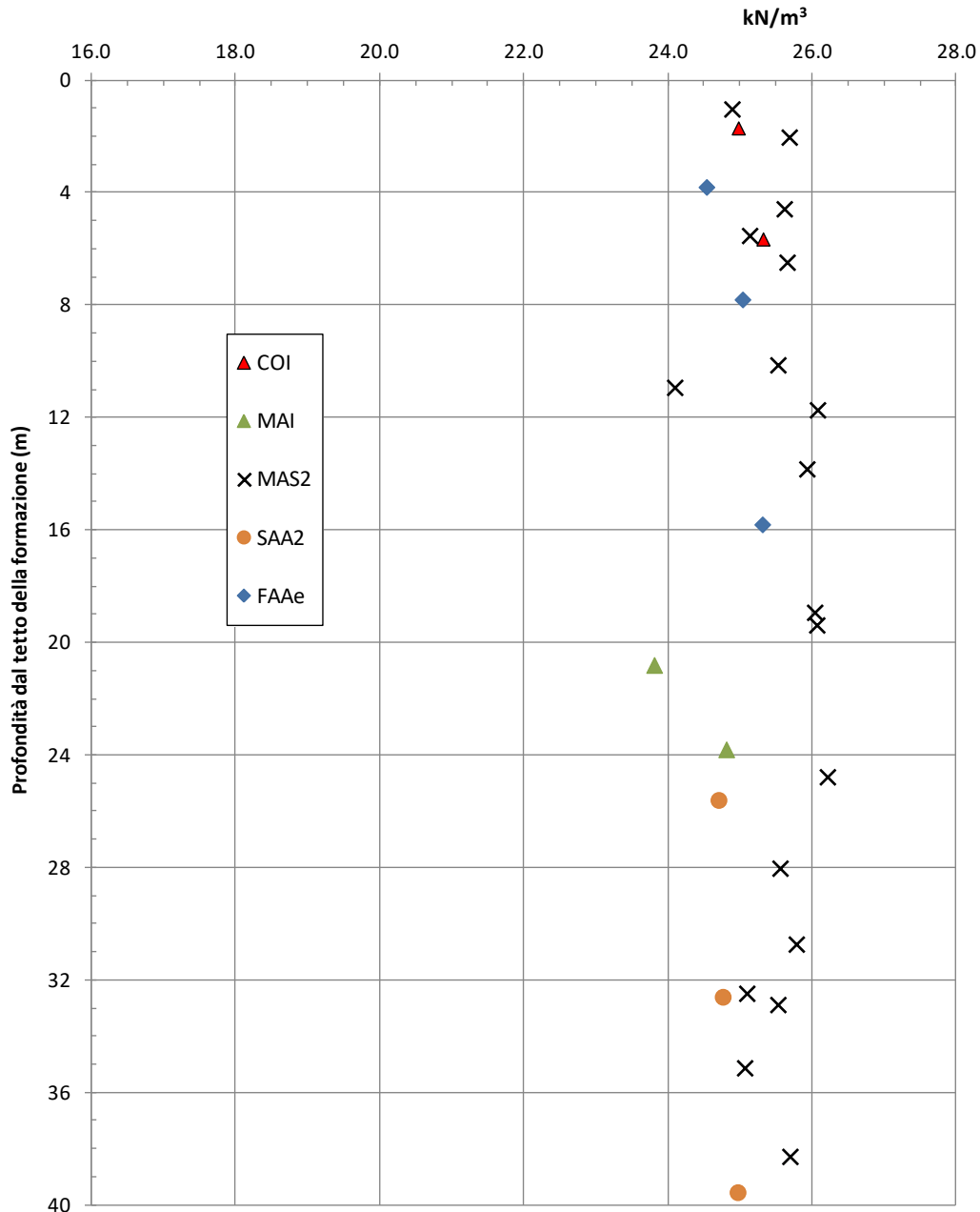
figura 11.1: Peso di volume per le diverse formazioni geologiche dell'unità CL
