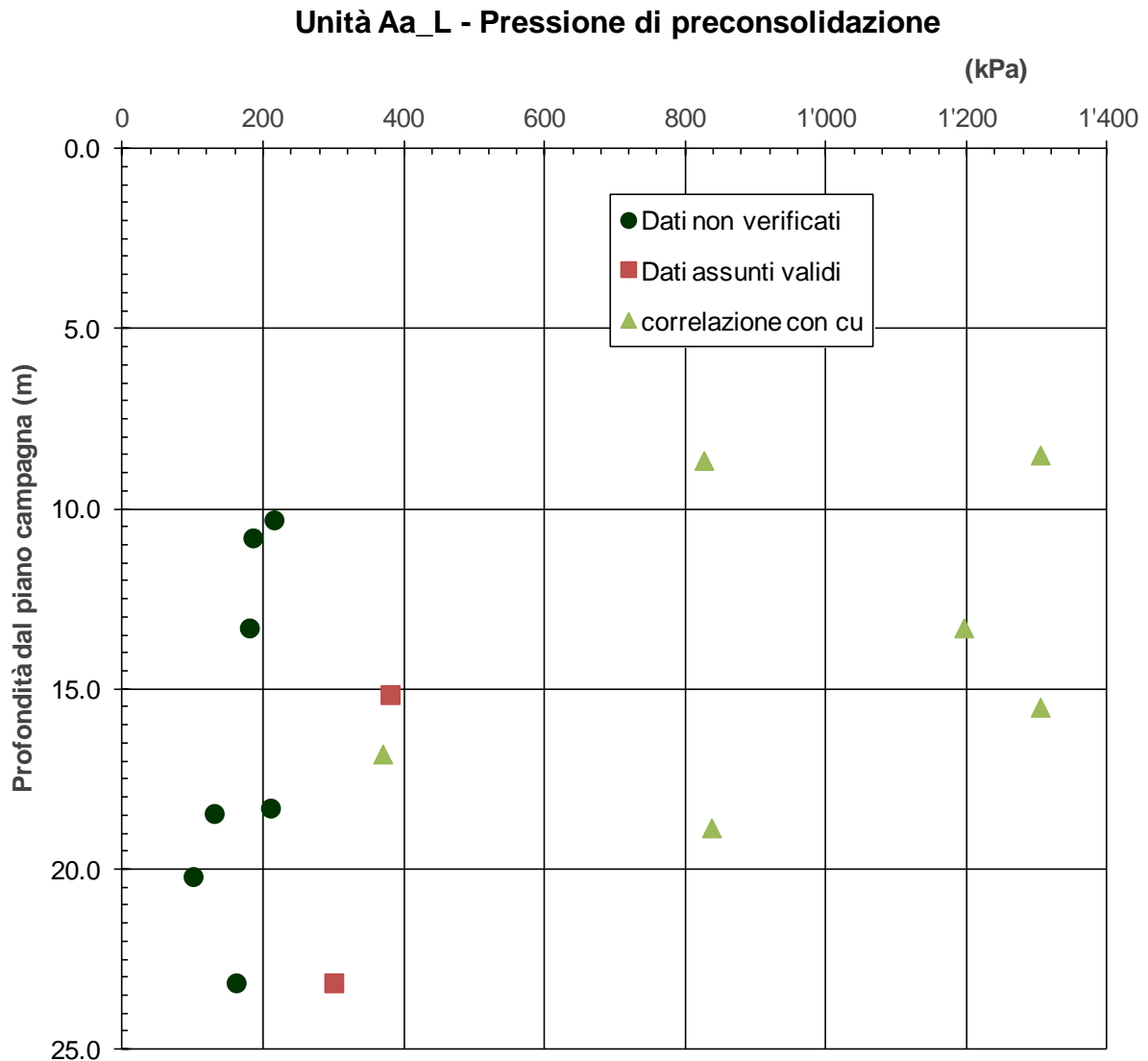
figura 14.8: Pressione di preconsolidazione in funzione della profondità dal p.c.
