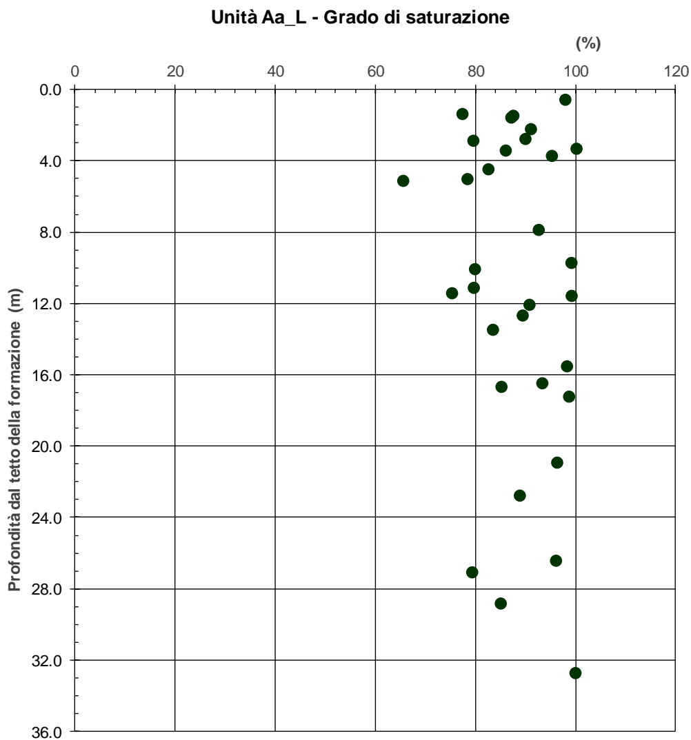
figura 14.6: Grado di saturazione in funzione della profondità
