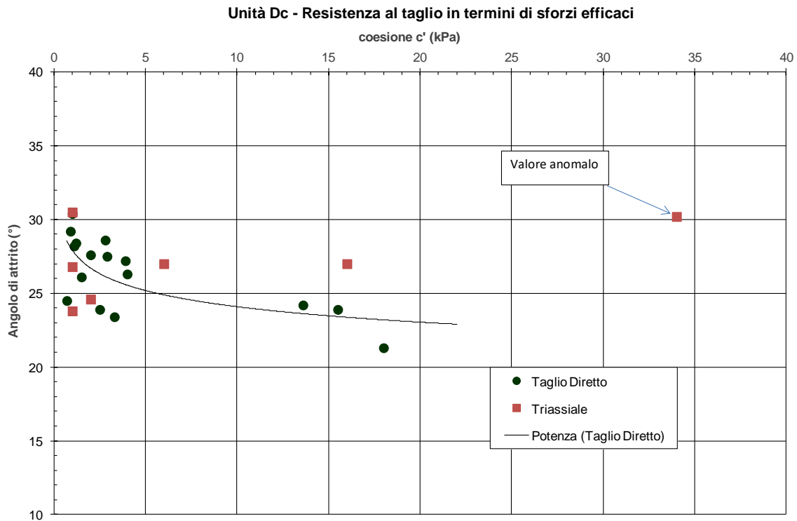
figura 10.10: Relazione c' - \phi' da prove triassiali e di taglio diretto
