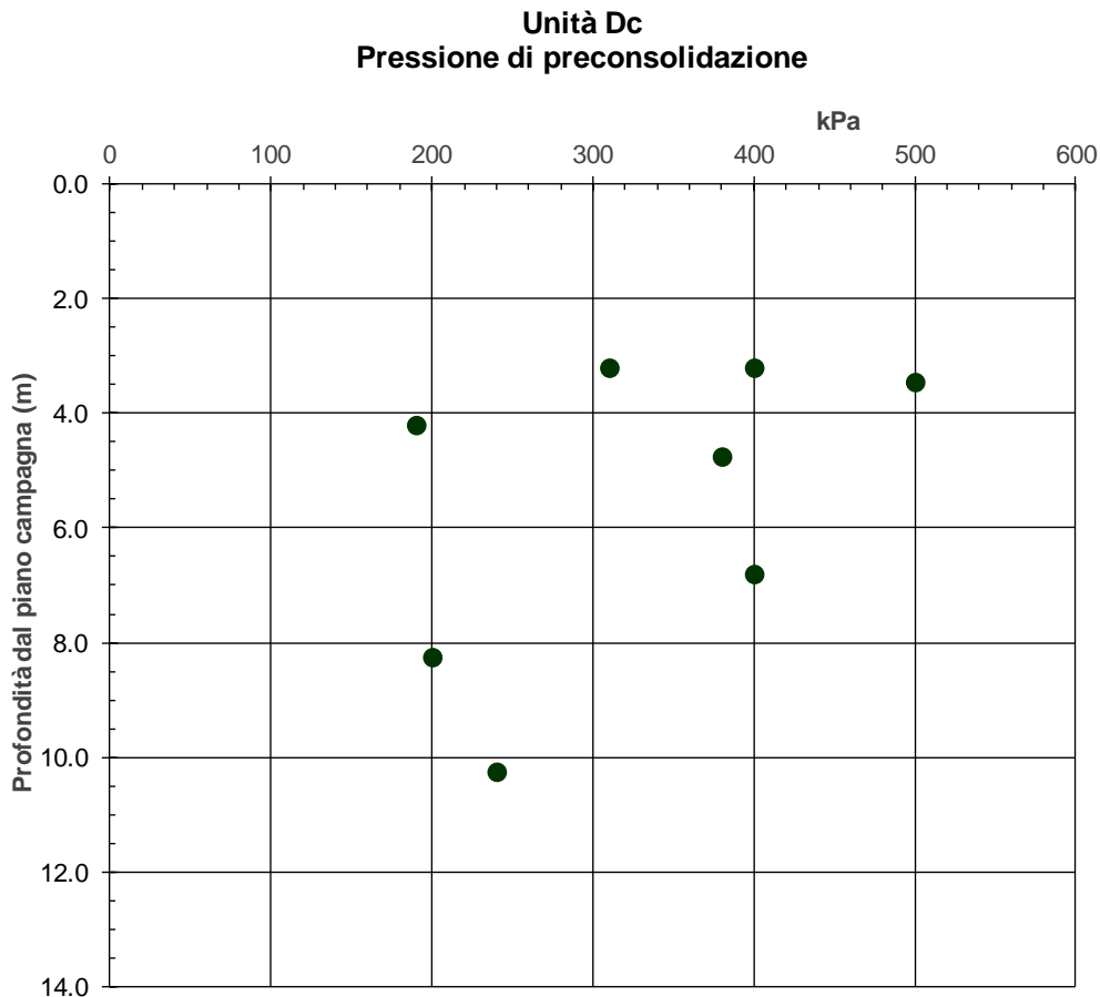
figura 10.8: pressione di preconsolidazione in funzione della profondità
