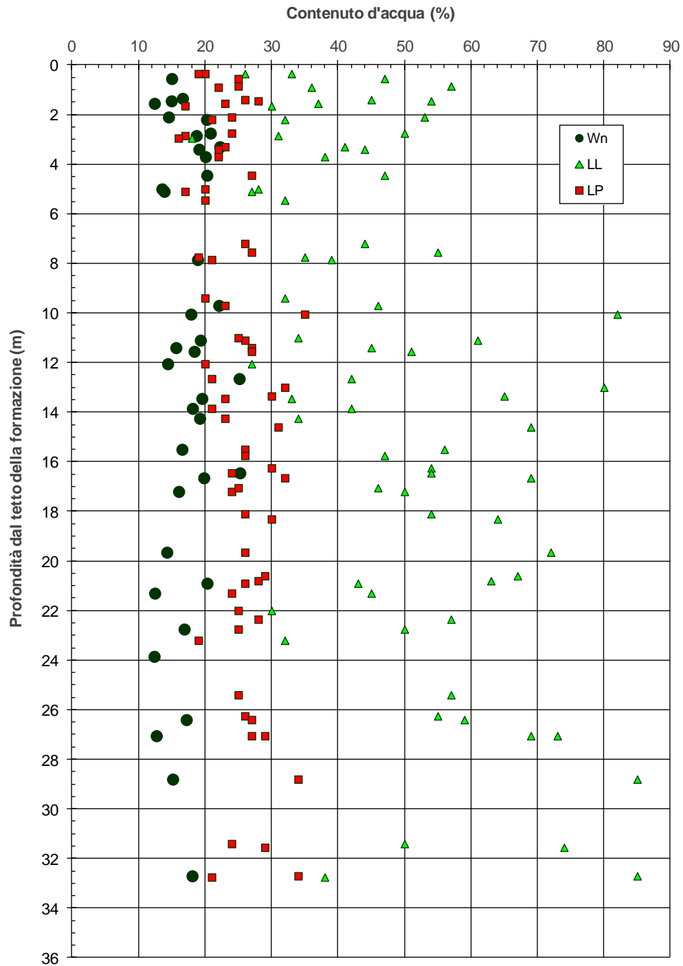
figura 14.4: Limiti di Atterberg e umidità naturale in funzione della profondità
