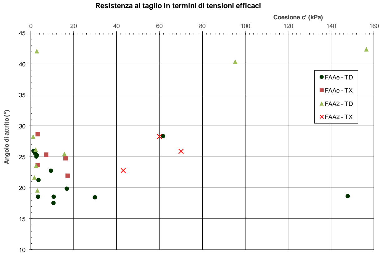
figura 14.10: Resistenza al taglio in termini di sforzi efficaci
