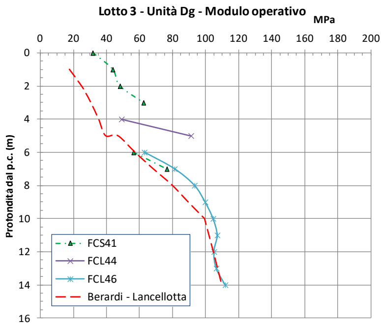
figura 10.30: Confronto con correlazione Berardi Lancellotta (Rif. [32])
