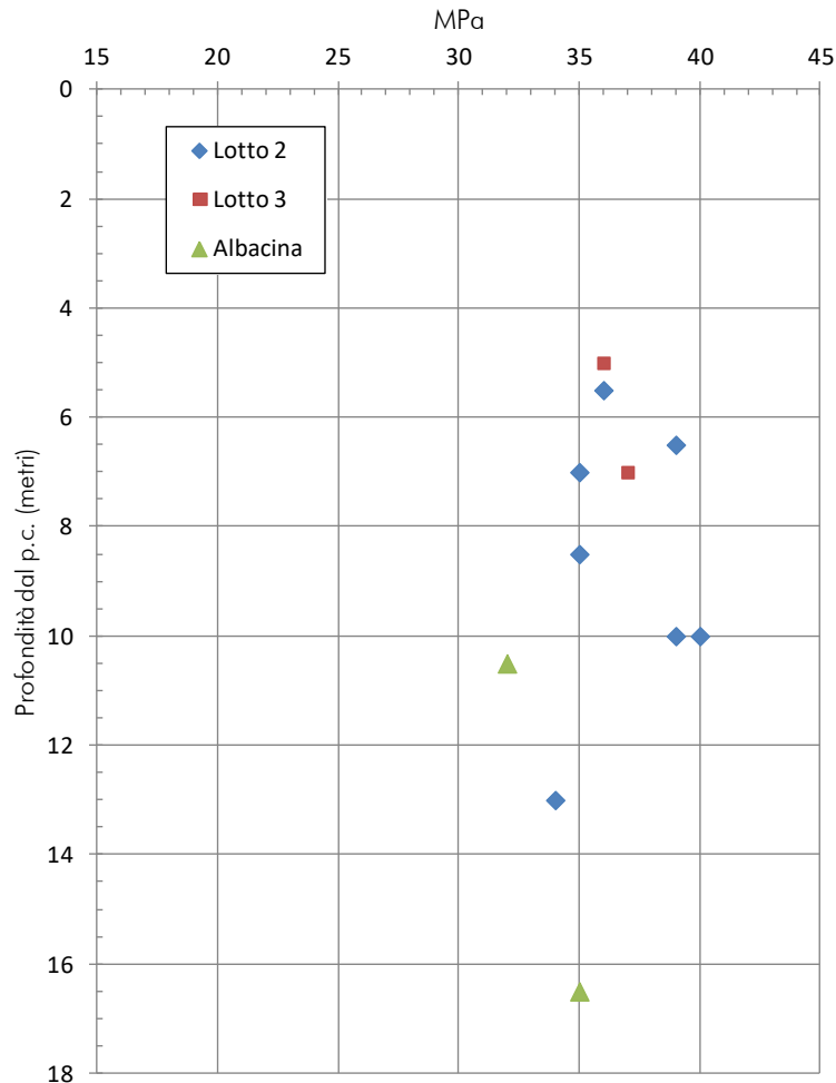
figura 10.22: Angolo di attrito da prove dilatometriche
