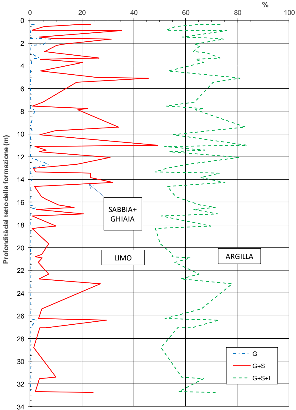
figura 14.2: Andamento granulometrico
