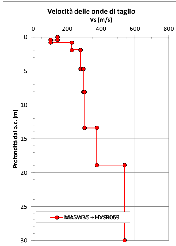
figura 15.11: MASW35 - Velocità delle onde di taglio con la profondità
