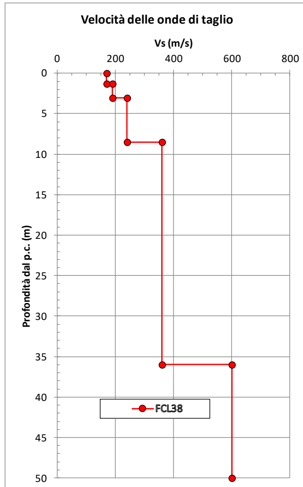
figura 15.14: DH FCL38 - Velocità delle onde di taglio con la profondità
