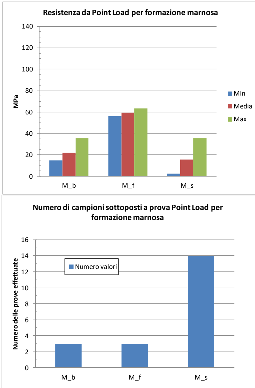
figura 12.7: Resistenza Point Load e numero di prove per formazione
