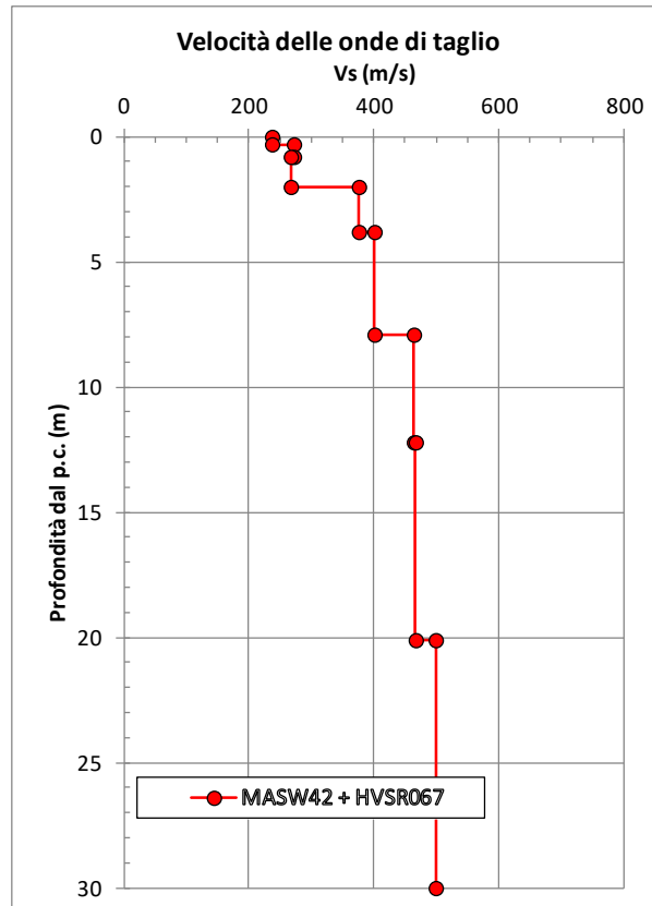
figura 15.16: MASW42 - Velocità delle onde di taglio con la profondità
