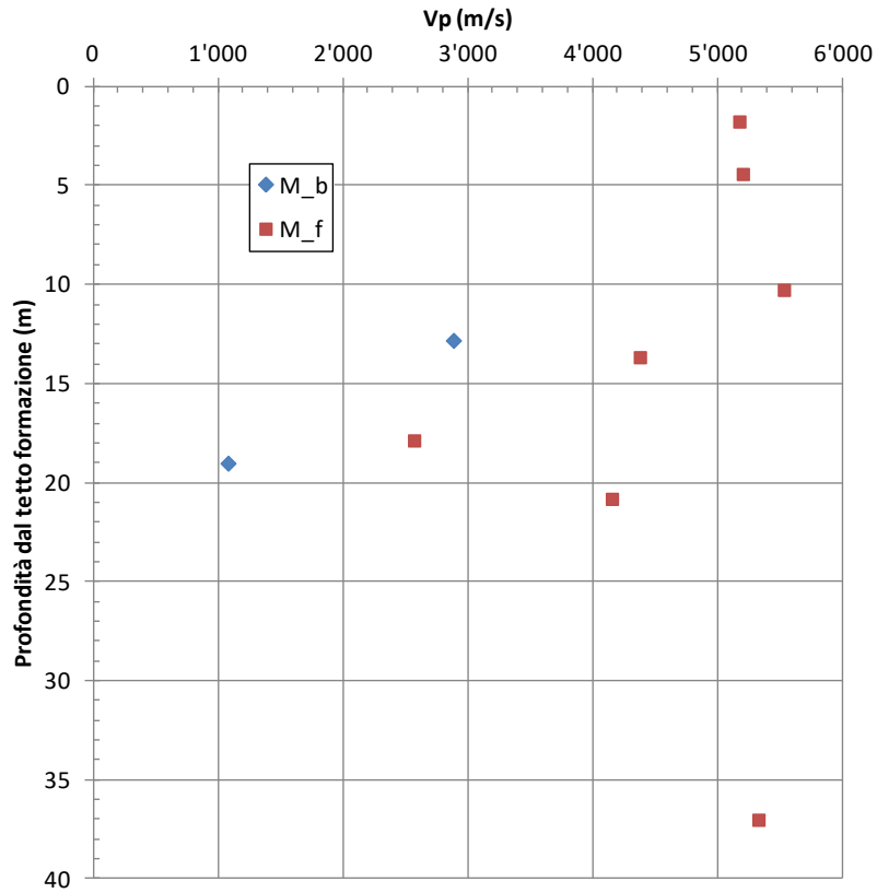
figura 12.9: Velocità delle onde V_p suddivise per unità geotecnica
