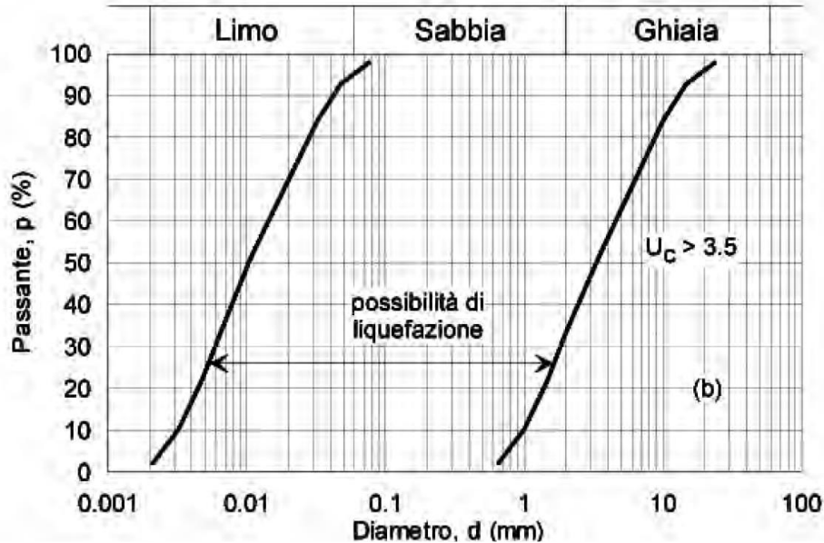
figura 15.21: Fuso granulometrico dei materiali suscettibili di liquefazione (Rif. [1])
