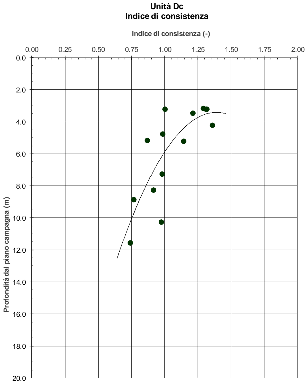
figura 10.5: Indice di consistenza in funzione della profondità
