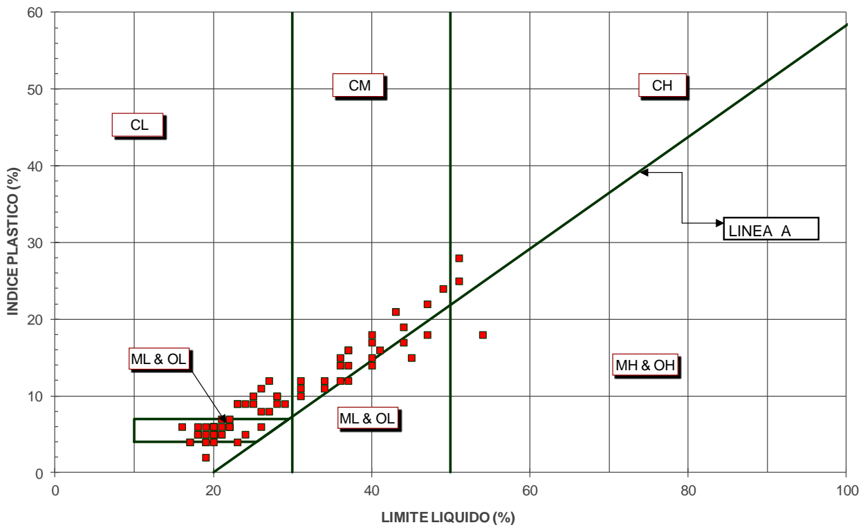
figura 10.1: Carta di Plasticità alluvioni terrazzate
