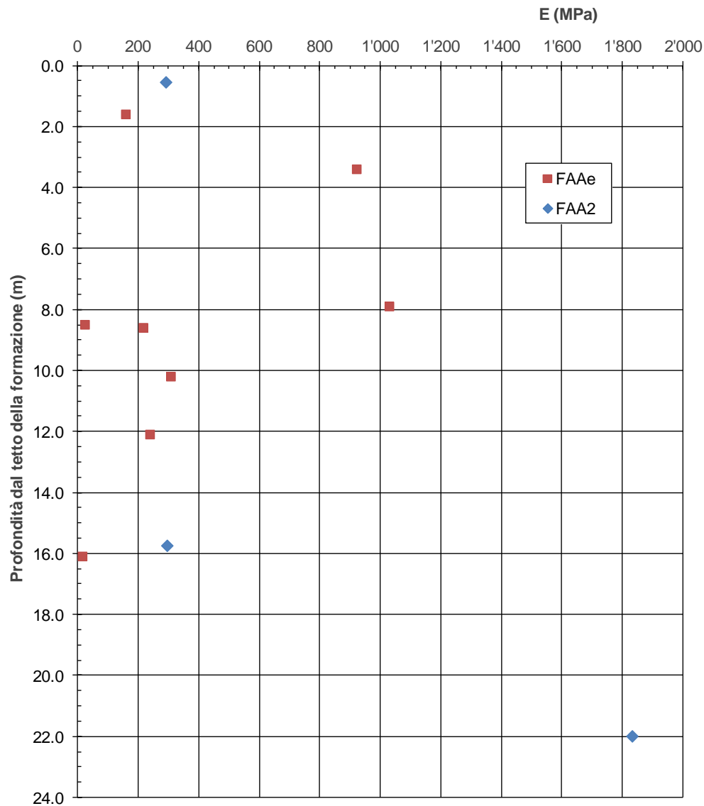
figura 14.13: Modulo elastico E_u desunto da prove dilatometriche
