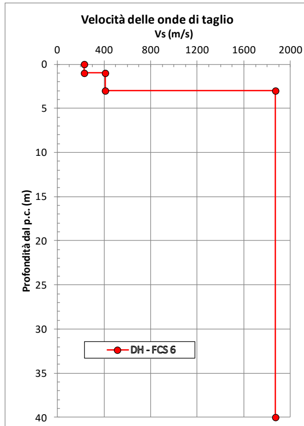
figura 15.3: DH FCS6 - Velocità delle onde di taglio con la profondità
