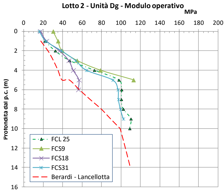
figura 10.29: Confronto con correlazione Berardi Lancellotta (Rif. [32])
