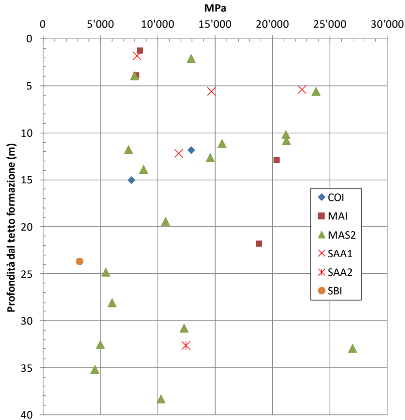
figura 11.10: Moduli di taglio G_0 suddivisi per formazione geologica
