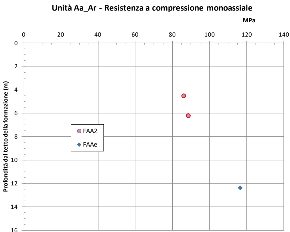
figura 14.14: Resistenza a compressione
