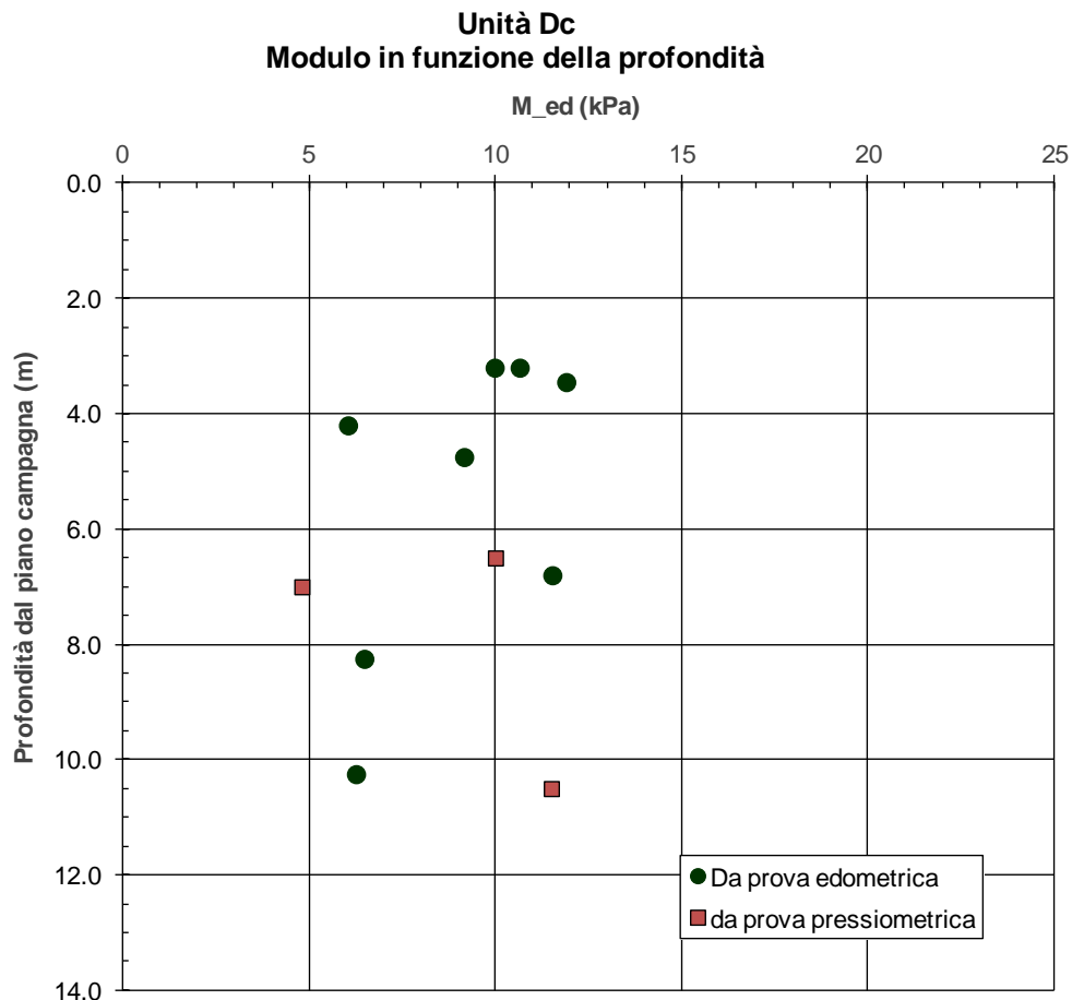
figura 10.9: Modulo edometrico in funzione della profondità
