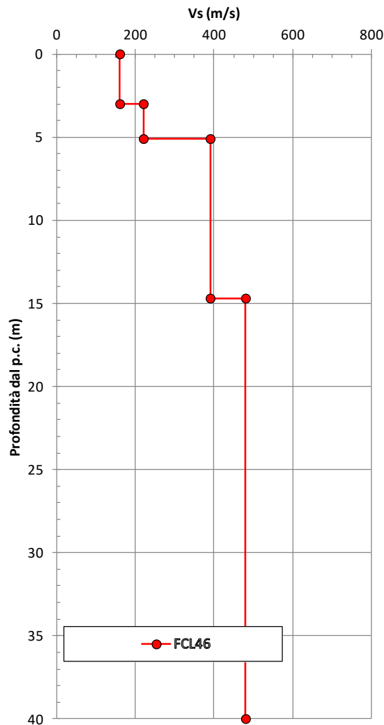
figura 15.19: DH FCL46 - Velocità delle onde di taglio con la profondità
