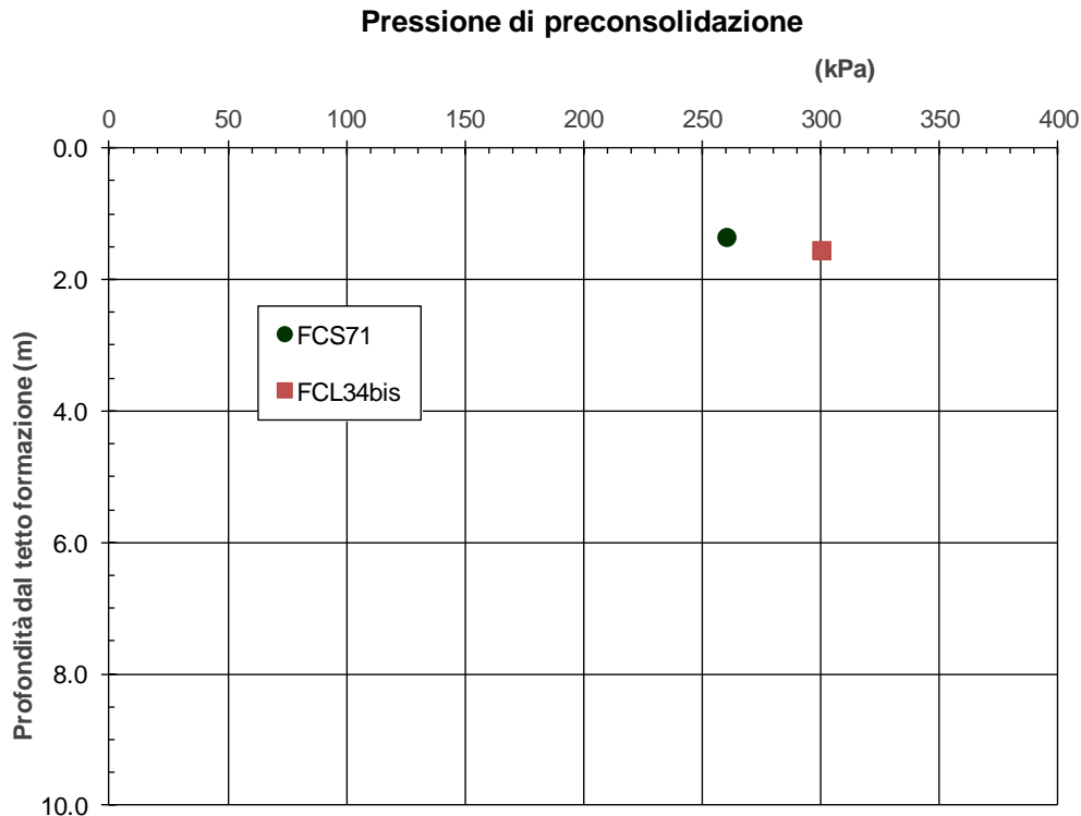
figura 13.6: Pressione di consolidazione in funzione della profondità
