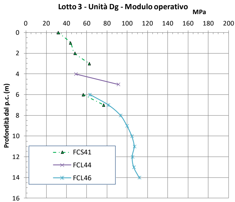
figura 10.26: Lotto 3 –Andamento di E_{op,2} con la profondità
