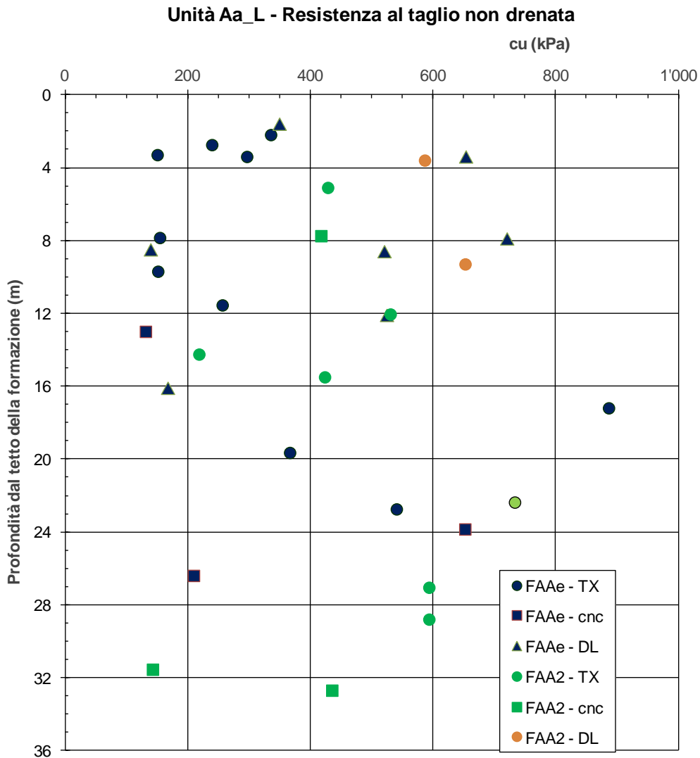
figura 14.12: Resistenza al taglio in condizioni non drenata in funzione della profondità
