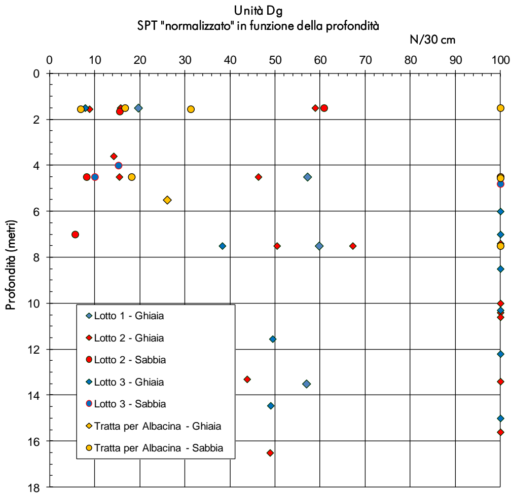
figura 10.19: SPT “normalizzato” in funzione della profondità
