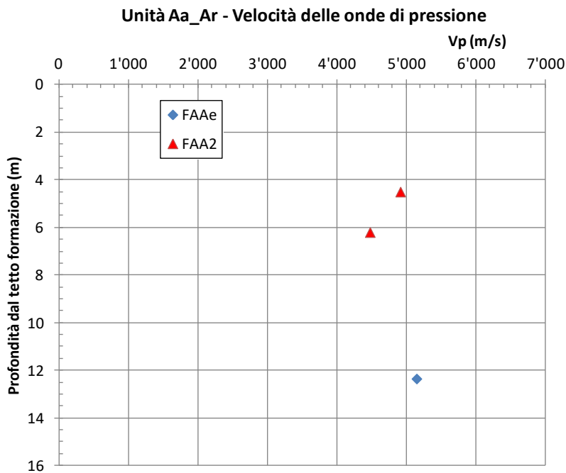
figura 14.16: Velocità delle onde V_p
