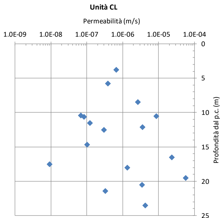
figura 11.14: Risultati prove di permeabilità
