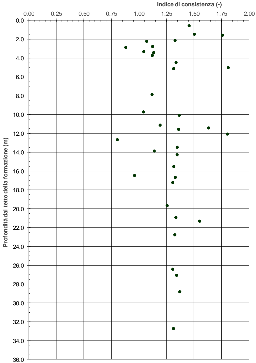
figura 14.5: Indice di consistenza in funzione della profondità
