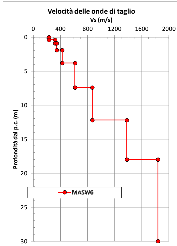
figura 15.2: MASW6 - Velocità delle onde di taglio con la profondità
