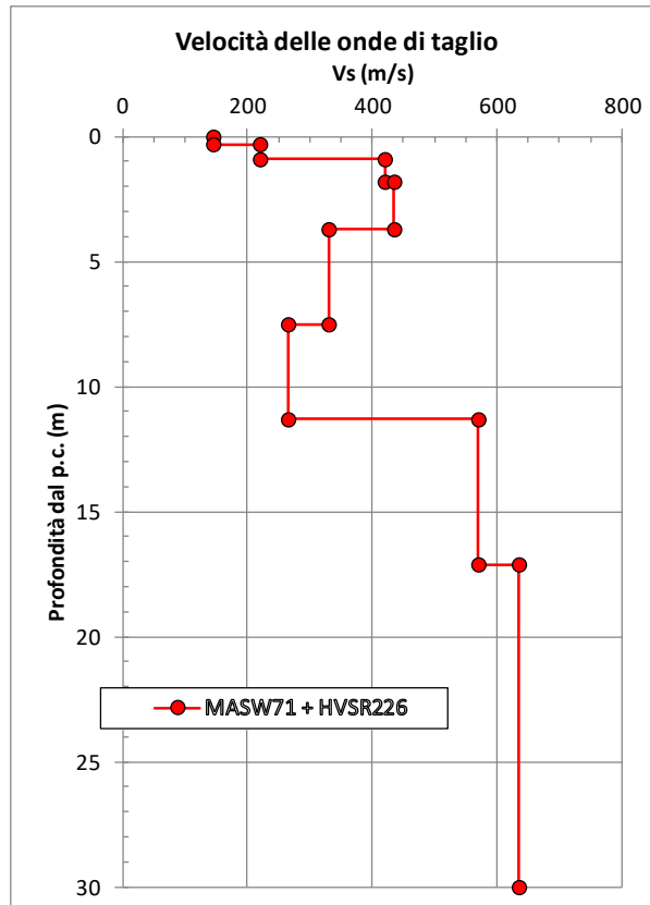
figura 15.1: MASW71 - Velocità delle onde di taglio con la profondità
