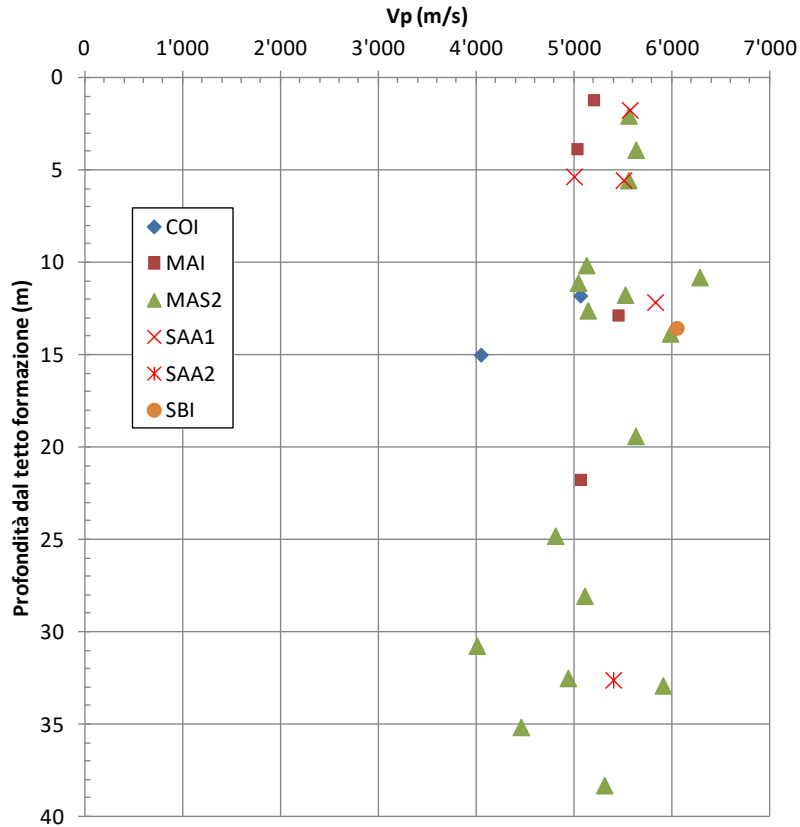
figura 11.8: Velocità delle onde V_p suddivise per formazione geologica
