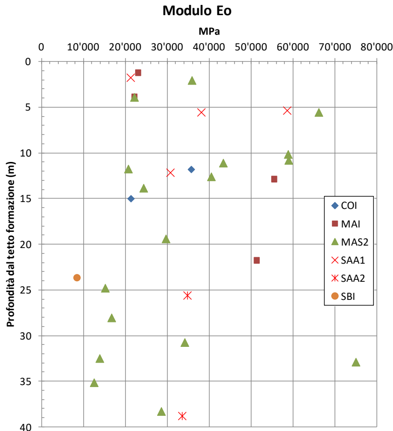
figura 11.11: Moduli elastici E 0 suddivisi per formazione geologica
