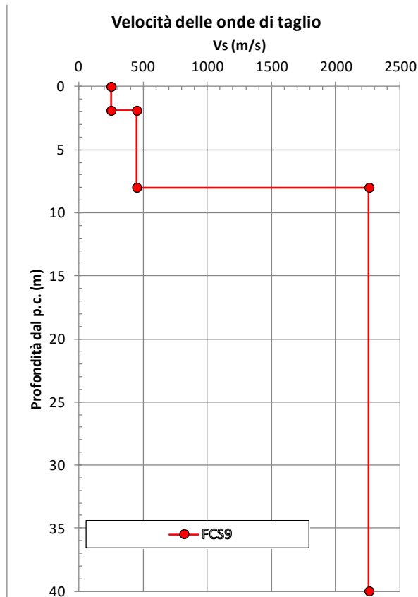
figura 15.4: DH FCS9 - Velocità delle onde di taglio con la profondità
