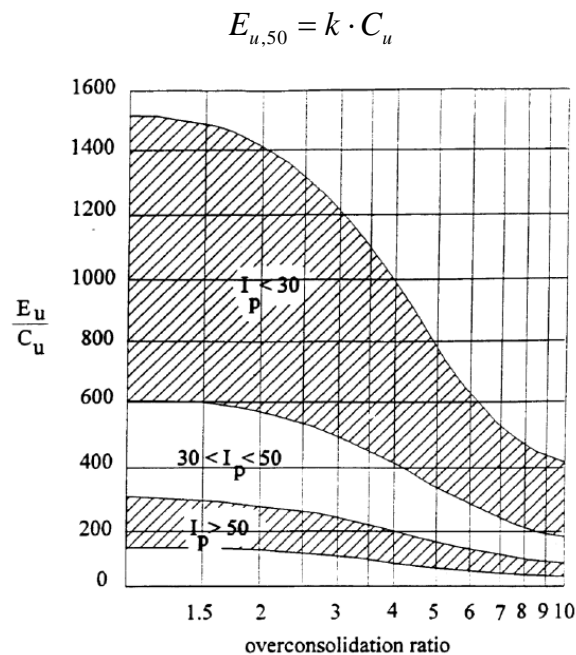
figura 8.2: Correlazione di Duncan e Buchignani (1976)
