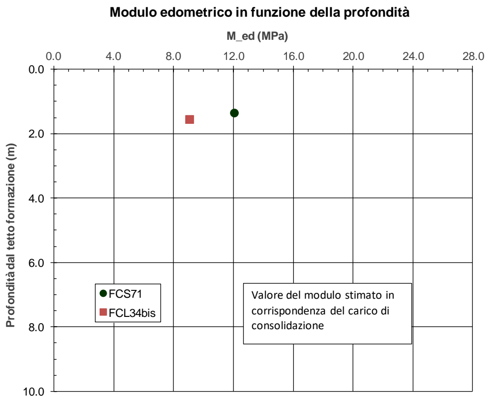
figura 13.7: Modulo edometrico in funzione della profondità
