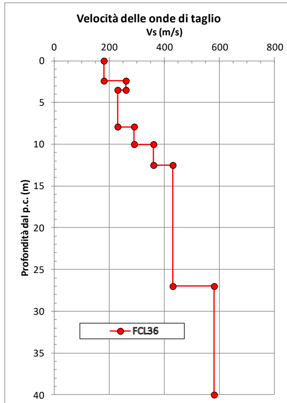
figura 15.13: DH FCL36 - Velocità delle onde di taglio con la profondità
