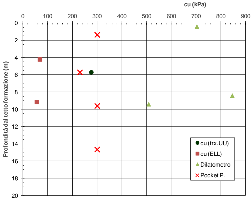
figura 13.9: Resistenza al taglio in condizioni non drenate
