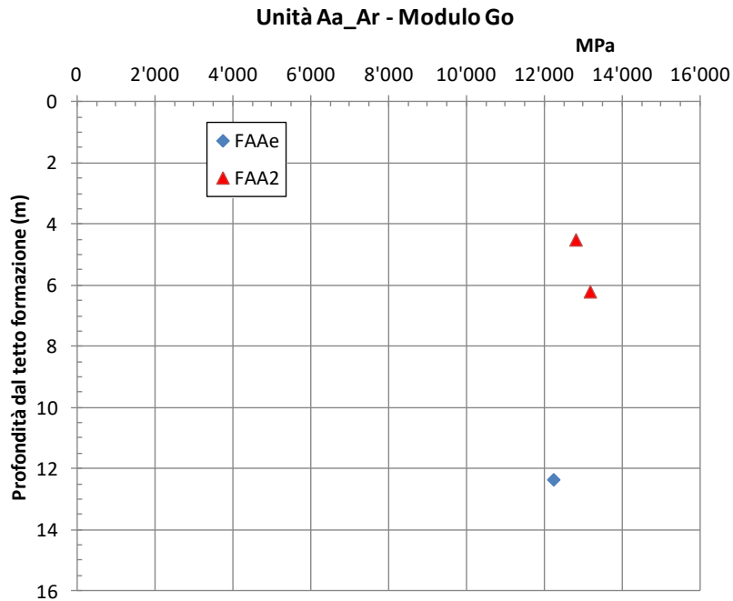
figura 14.18: Modulo G_0
