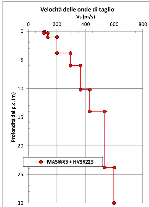
figura 15.17: MASW43 - Velocità delle onde di taglio con la profondità
