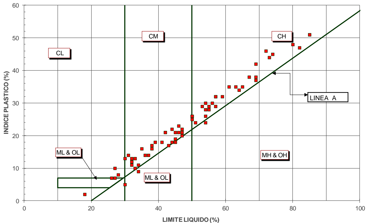
figura 14.1: Carta di Plasticità componente pelitica Argille Azzurre
