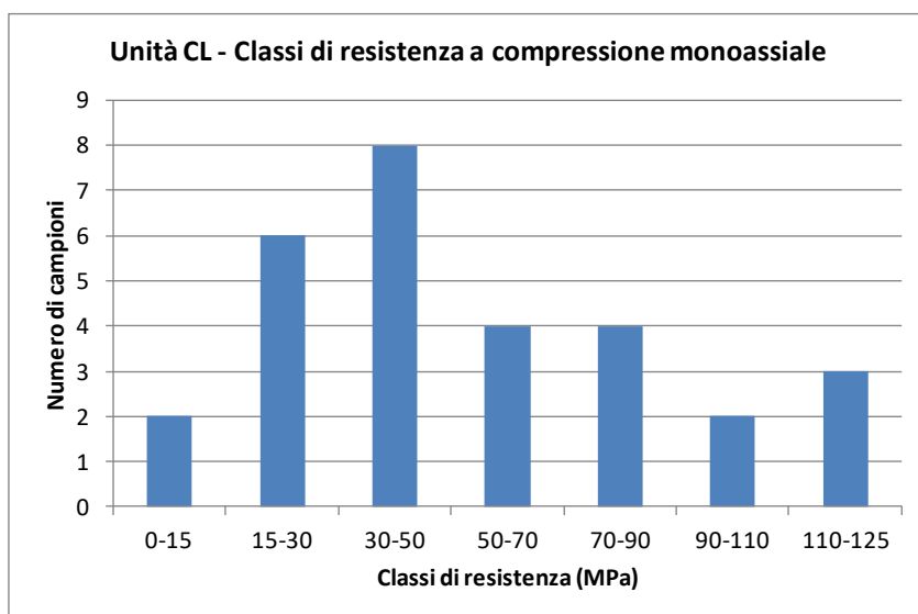
figura 11.5: Compressione monoassiale – Numero di risultati per classe di resistenza
