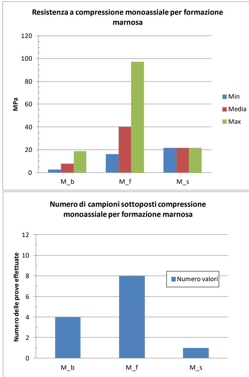
figura 12.6: Resistenza a compressione e numero di prove per formazione
