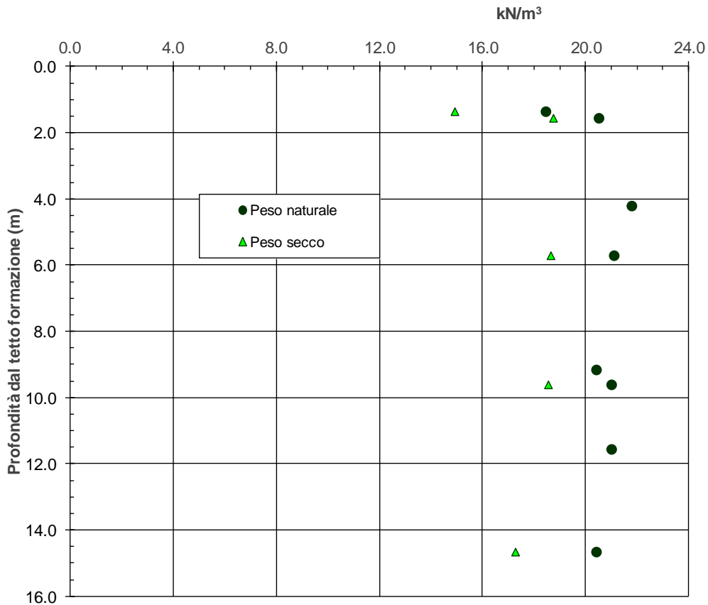
figura 13.2: Peso di volume in funzione della profondità
