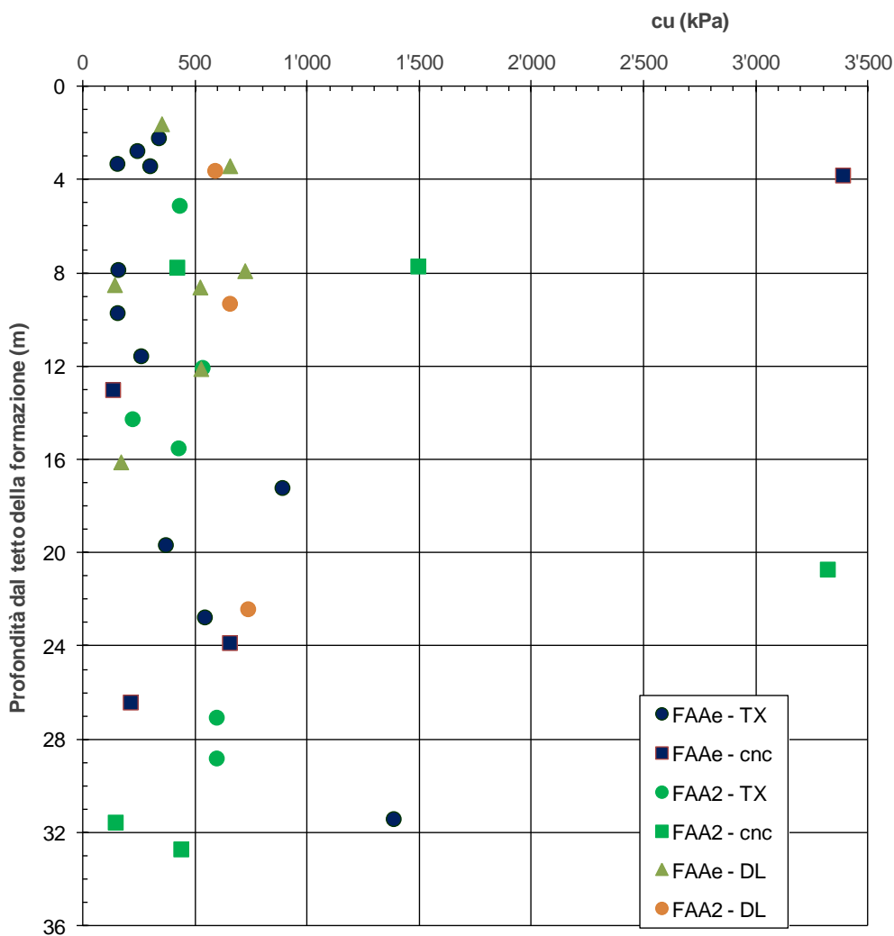
figura 14.11: Resistenza al taglio in condizioni non drenata in funzione della profondità
