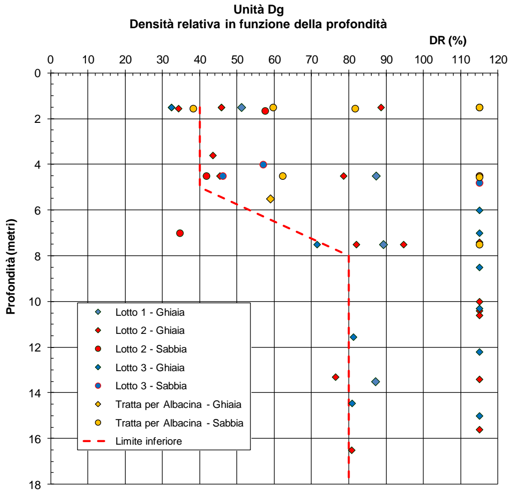
figura 10.20: Densità relativa in funzione della profondità (Skempton 1986)
