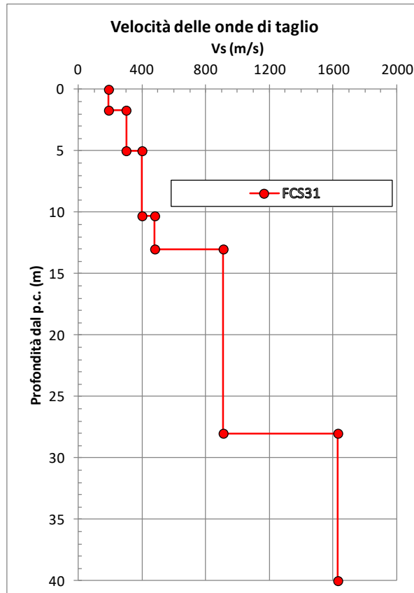
figura 15.10: DH FCS31 - Velocità delle onde di taglio con la profondità
