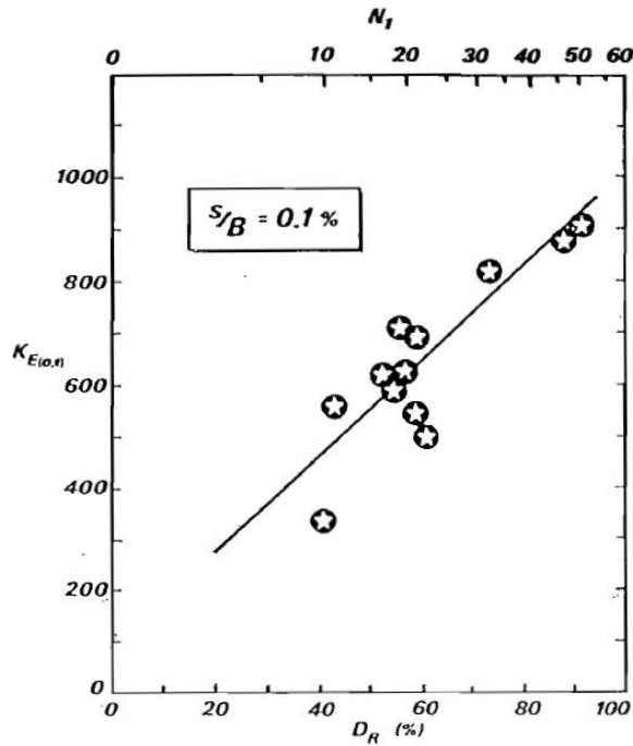
figura 7.2: Correlazione fra densità relativa e K_E
