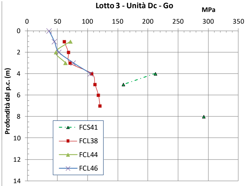
figura 10.13: Modulo Go a piccole deformazioni – Lotto 3
