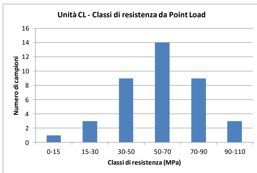
figura 11.6: Point Load – Numero di risultati per classe di resistenza
