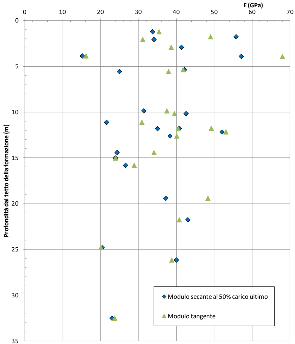
figura 11.7: Modulo elastico E_i formazioni calcaree
