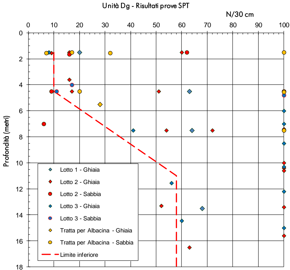
figura 10.18: Risultati prove SPT suddivisi per lotto
