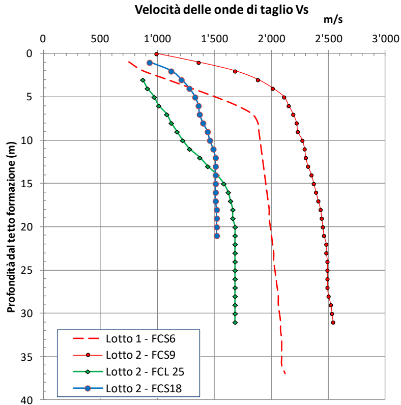
figura 11.12: Velocità delle onde di taglio da prove DH
