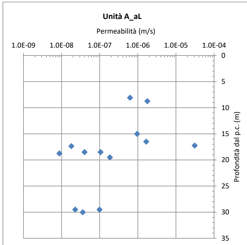
figura 14.7: Risultati prove di permeabilità
