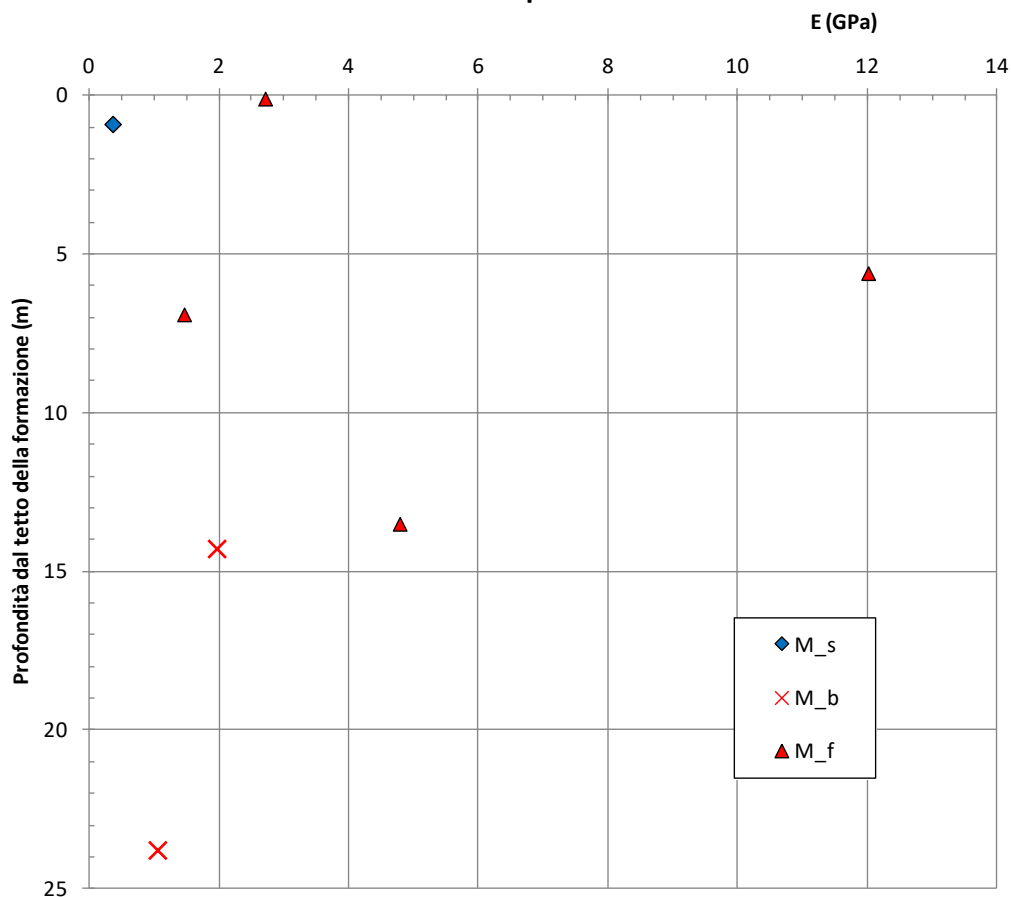
figura 12.14: Moduli elastici E rm da dilatometro, per unità geotecnica
