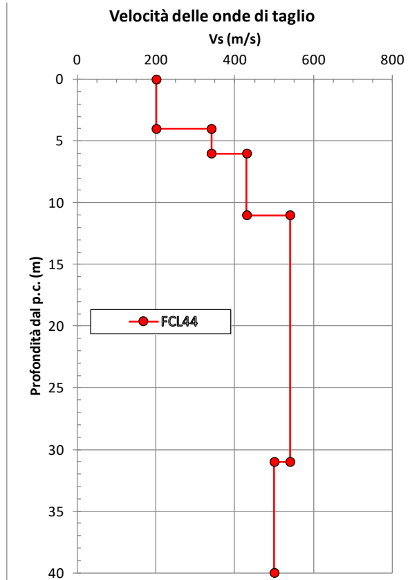
figura 15.18: DH FCL44 - Velocità delle onde di taglio con la profondità
