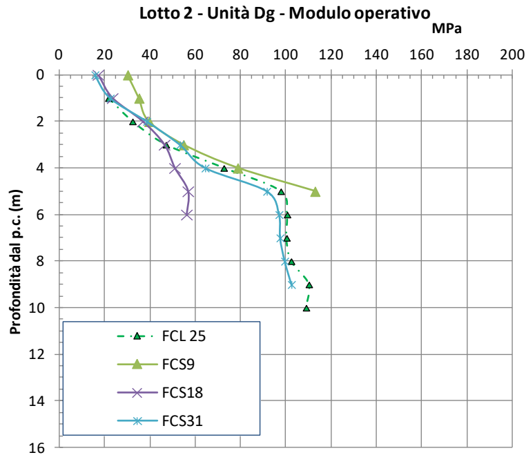
figura 10.25: Lotto 2 –Andamento di E_{op,2} con la profondità
