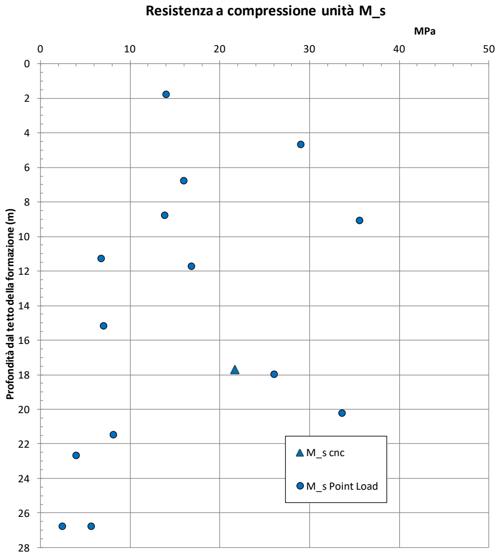
figura 12.5: Resistenza a compressione unità M s
