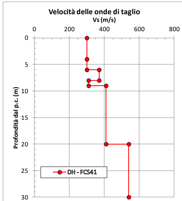
figura 15.15: DH FCS41 - Velocità delle onde di taglio con la profondità
