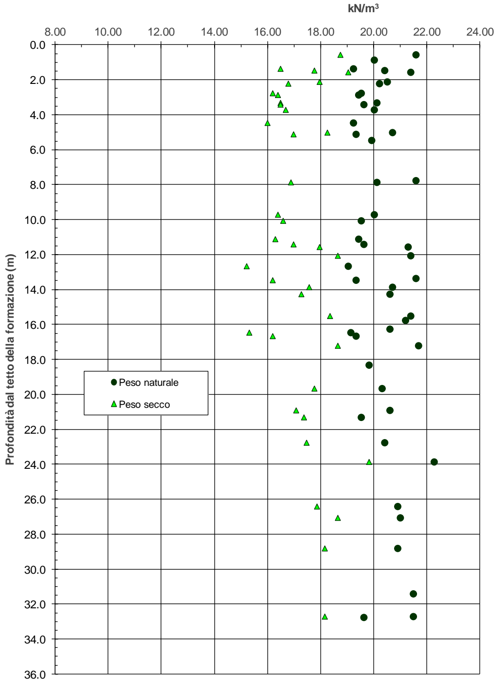
figura 14.3: Peso di volume in funzione della profondità
