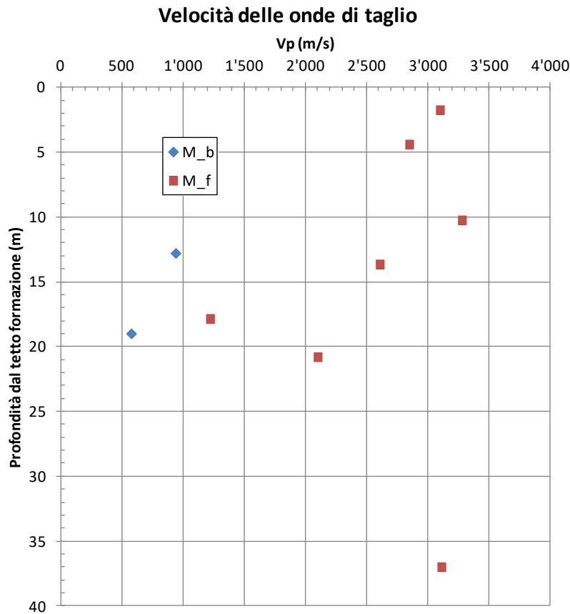
figura 12.10: Velocità delle onde V_s suddivise per unità geotecnica
