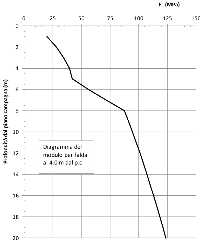
figura 10.27: Modulo di compressibilità per s/B \leq 0.1\%
