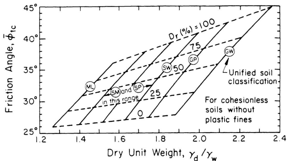
figura 7.1: Angolo di attrito in funzione del tipo di terreno e densità relativa
