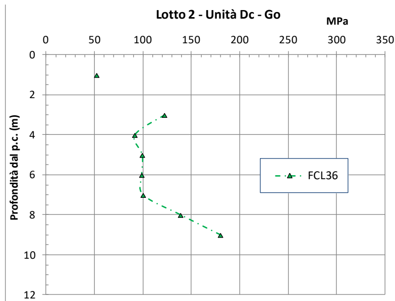
figura 10.12: Modulo G_0 a piccole deformazioni – Lotto 2
