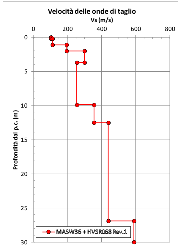
figura 15.12: MASW36 - Velocità delle onde di taglio con la profondità
