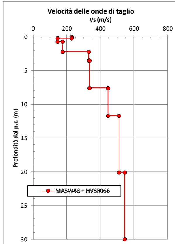
figura 15.20: MASW48 - Velocità delle onde di taglio con la profondità
