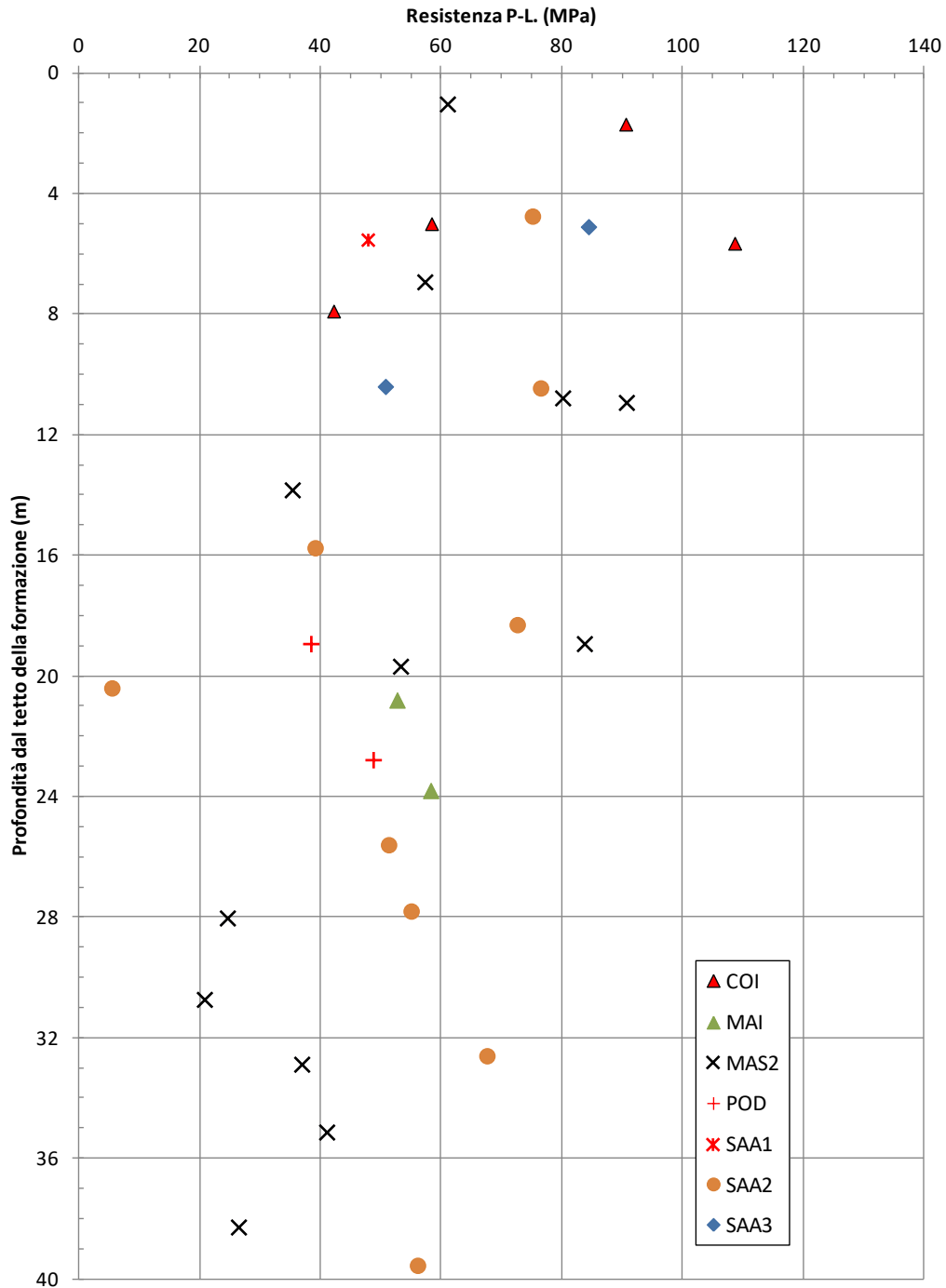
figura 11.4: Resistenza Point Load materiali calcarei per formazione
