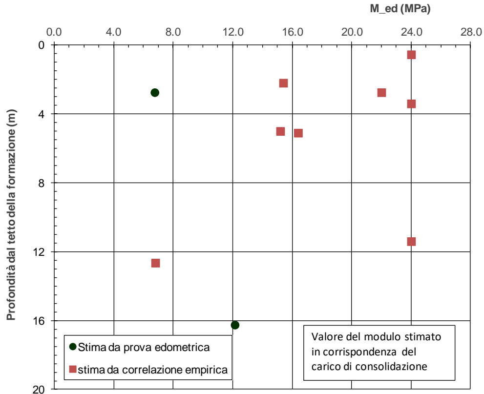
figura 14.9: Modulo edometrico in funzione della profondità
