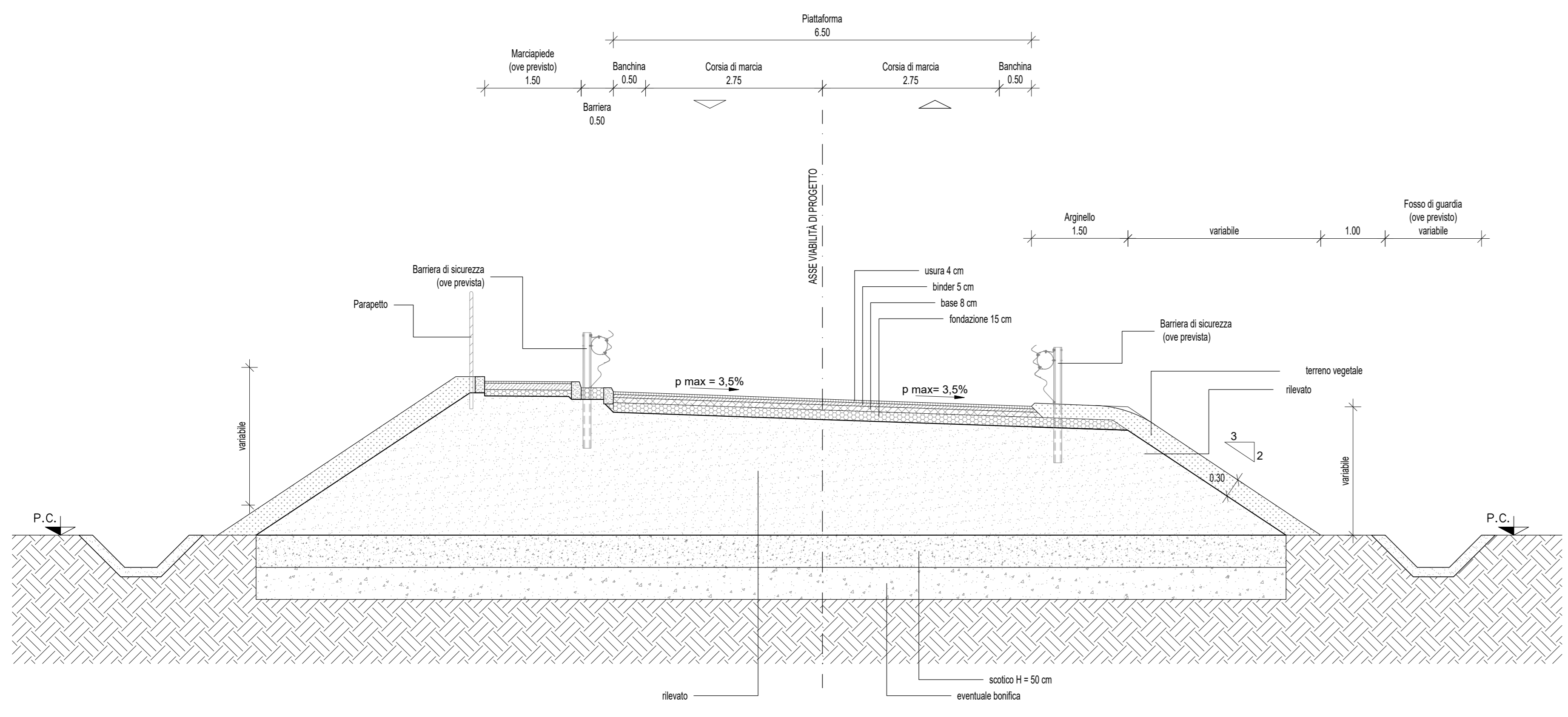
SEZIONI TIPO STRADALI PER VIABILITA' DI STRADE LOCALI A DESTINAZIONE PARTICOLARE IN CURVA - IN RILEVATO SCALA 1:50
