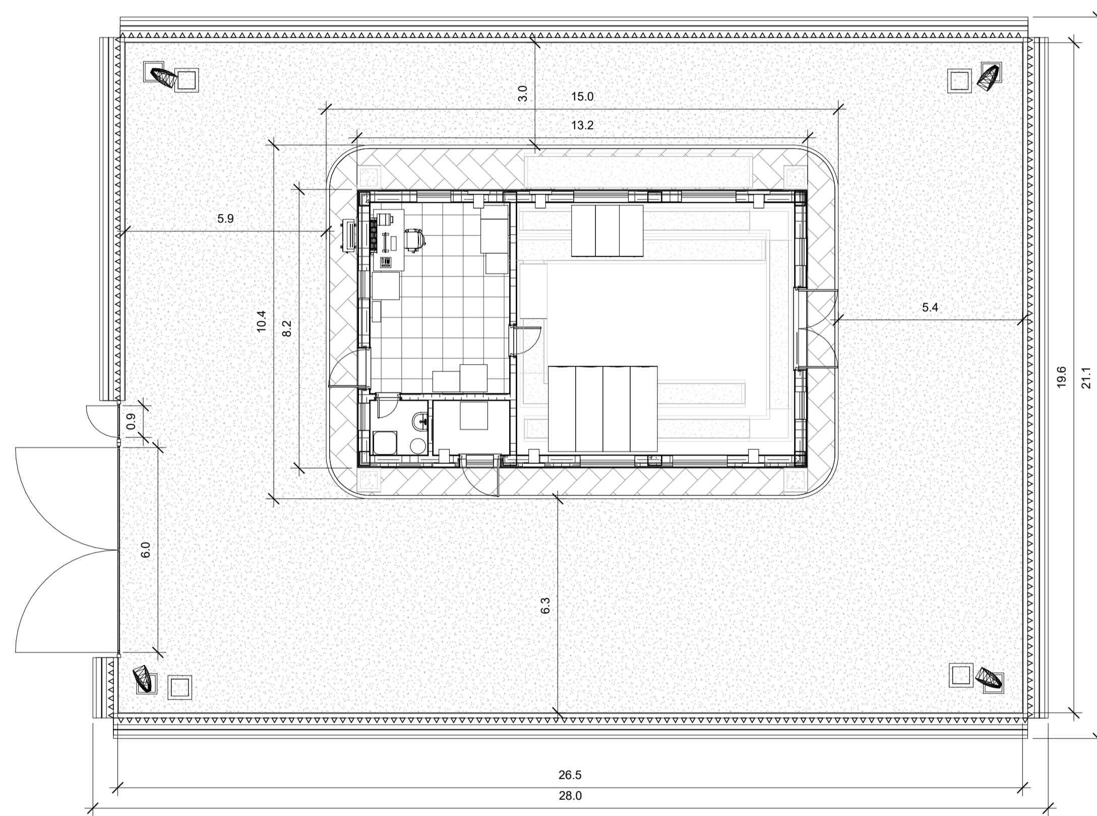
1 Disposizione apparecchiature (Layout) 1 : 100
