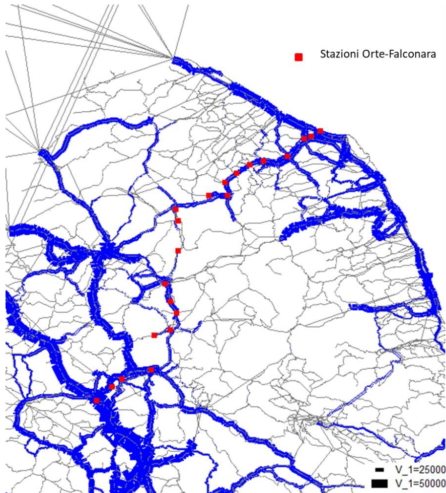
Figura 24 - Flussogrammi auto (veicoli/g), scenario progetto 2035
