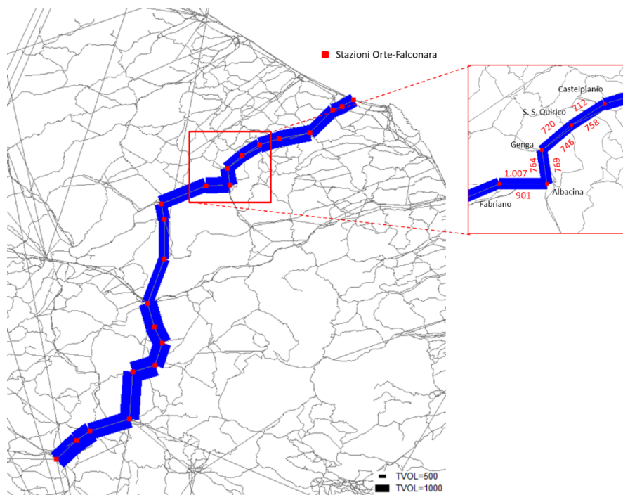
Figura 12 - Flussogramma del trasporto ferroviario (passeggeri/g), direttrice di progetto Orte-Falconara con focus sulle tratte di progetto, scenario 2019
