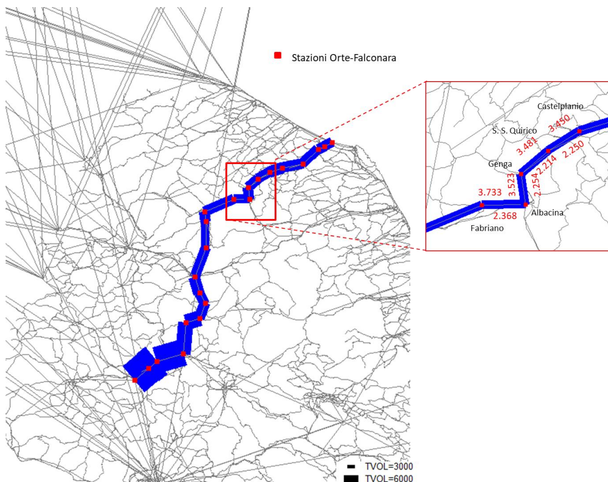
Figura 26 - Flussogrammi trasporto ferroviario (pax/g) linea Orte-Falconara, scenario di progetto 2035
