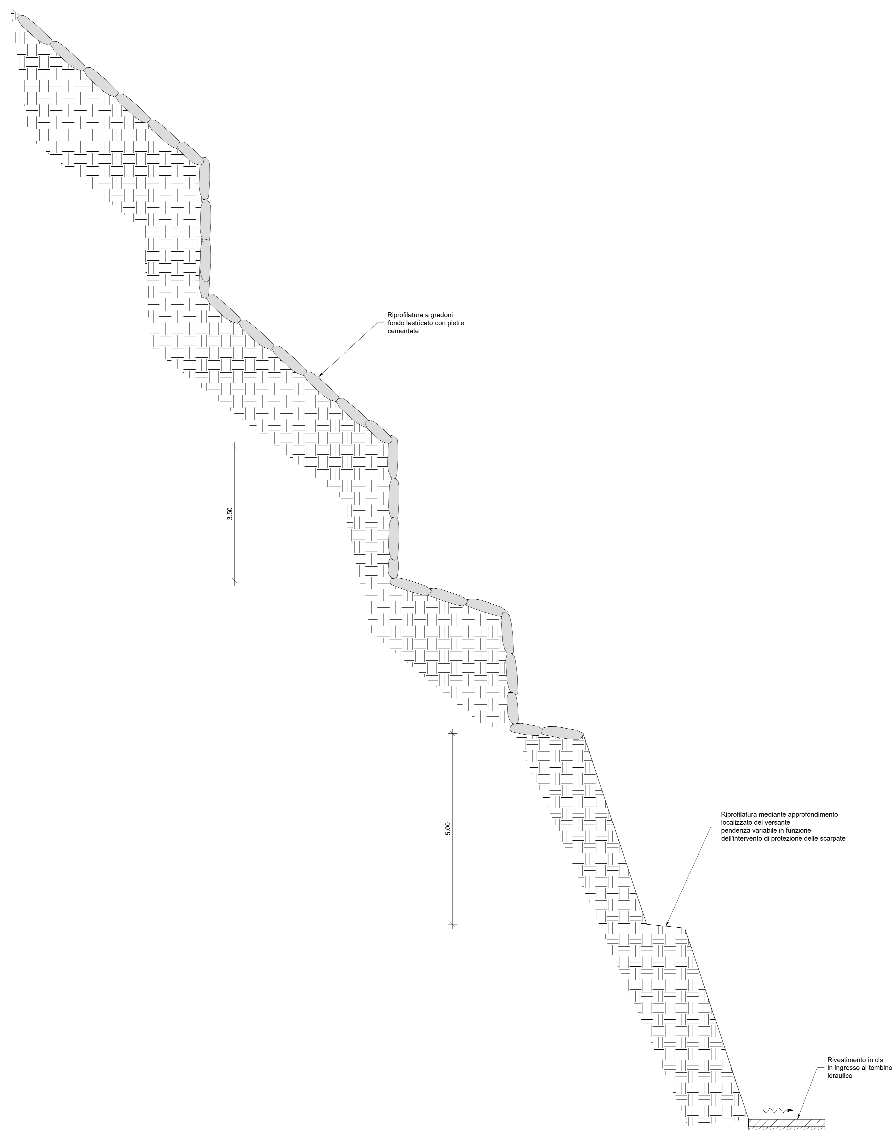
Riprofilatura a gradoni di ingresso ai tombini idraulici scala 1:50
