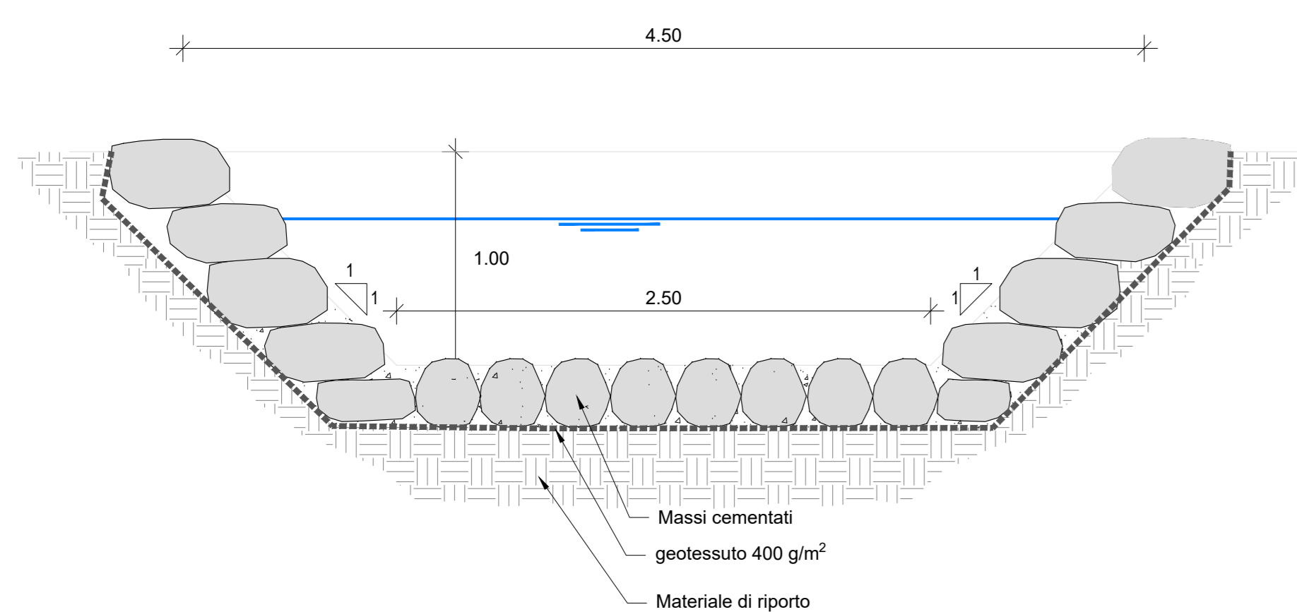
Riprofilatura alveo con canale trapezoidale scala 1:25
