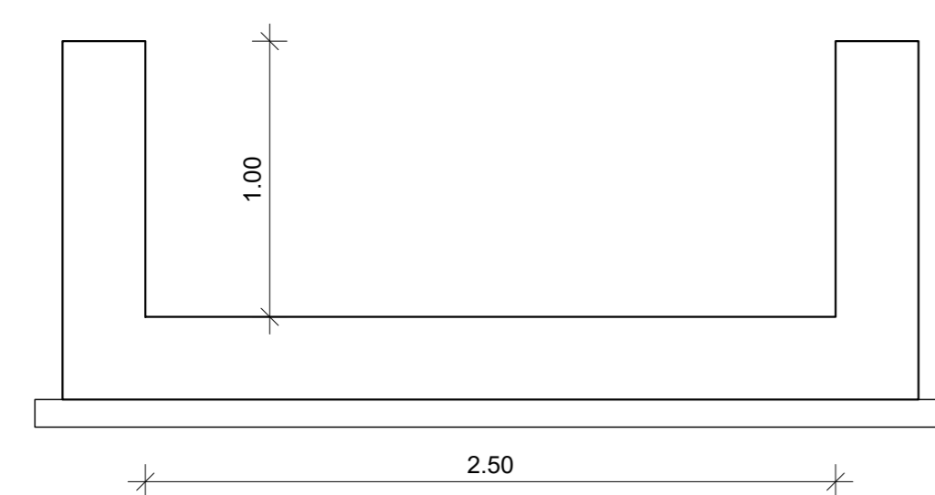
Riprofilatura alveo con canale rettangolare scala 1:25
