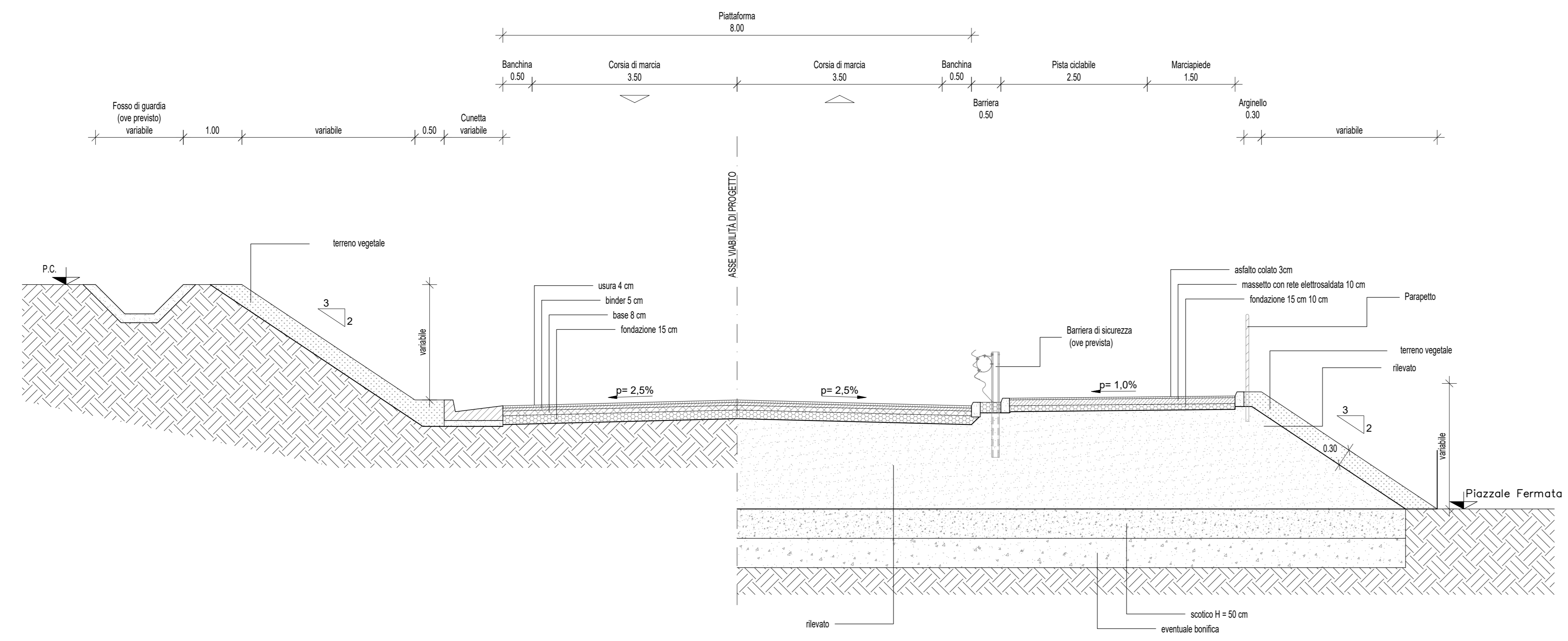
SEZIONE TIPO STRADALE CATEGORIA F LOCALI - AMBITO URBANO - CON CORSIE AUMENTATE A 3.50 m IN RETTIFILLO - MEZZA COSTA SCALA 1:50
