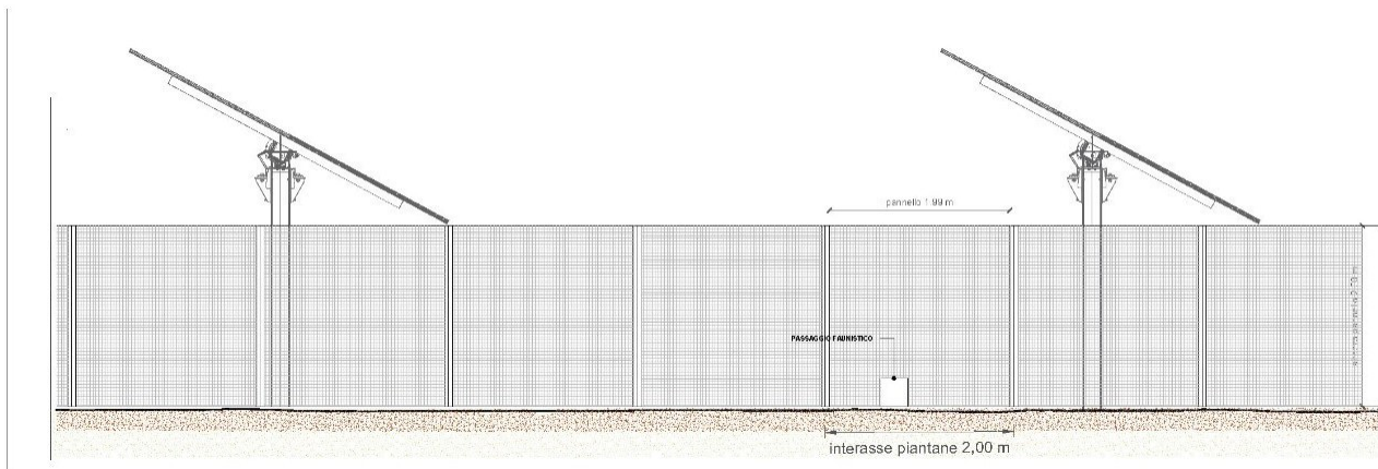
Figura 29 - Prospetto recinzione perimetrale senza mitigazione
