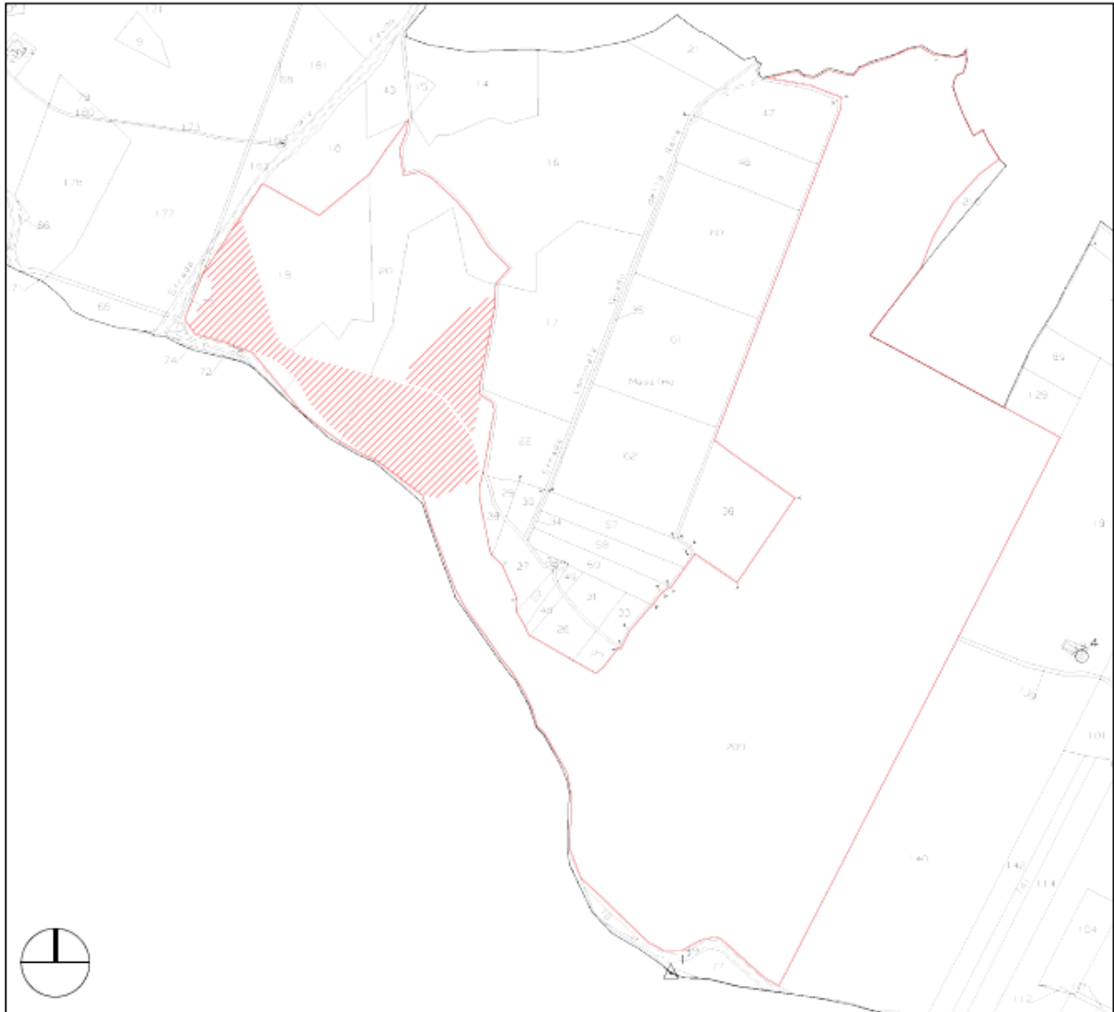
PLANIMETRIA CATASTALE CON IDENTIFICAZIONE DEI LOTTI DI INTERVENTO - scala 1:5000
