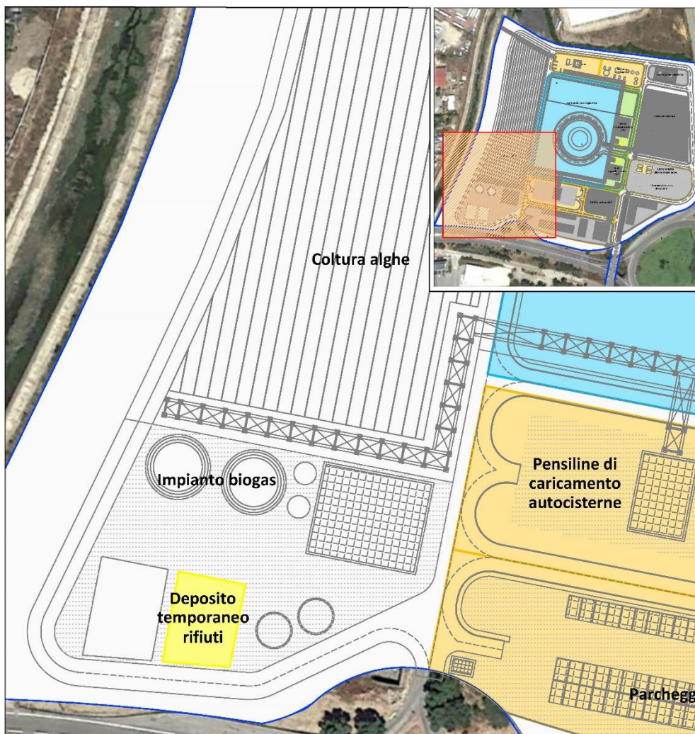
Figura III.12 – Ubicazione deposito temporaneo prima della raccolta
