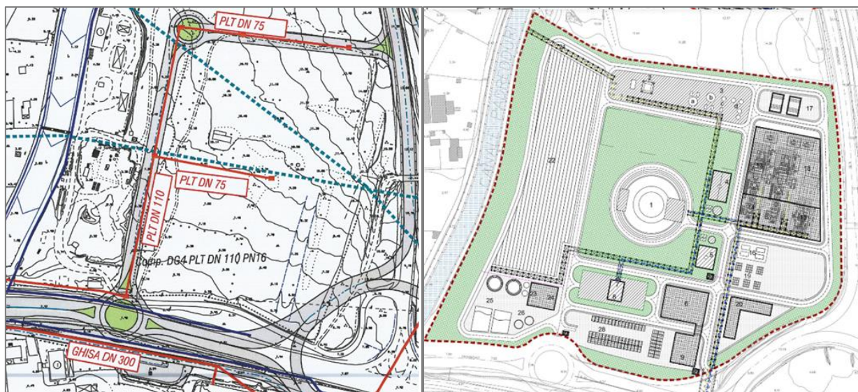
Figura III.6 – Viabilità di accesso e infrastrutture presenti
