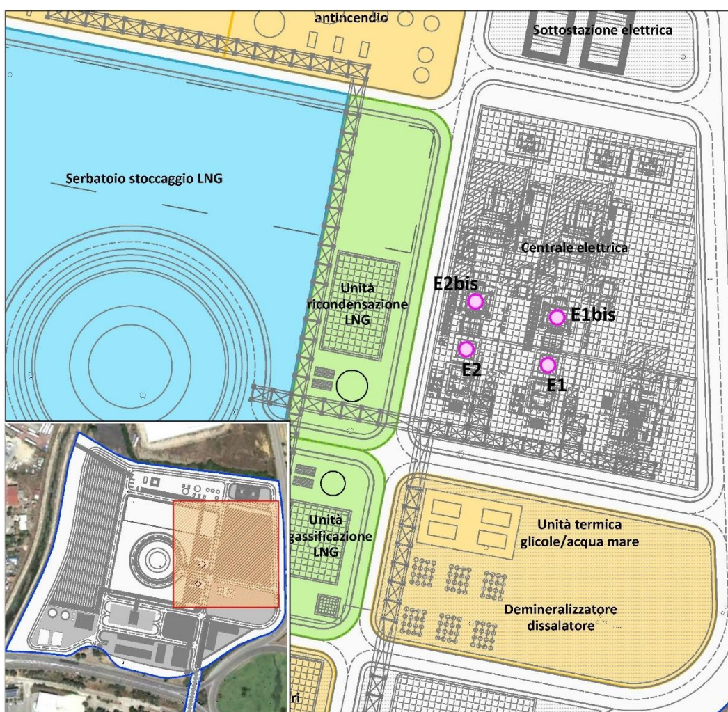
Figura III.9 – Ubicazione punti di emissione in atmosfera
