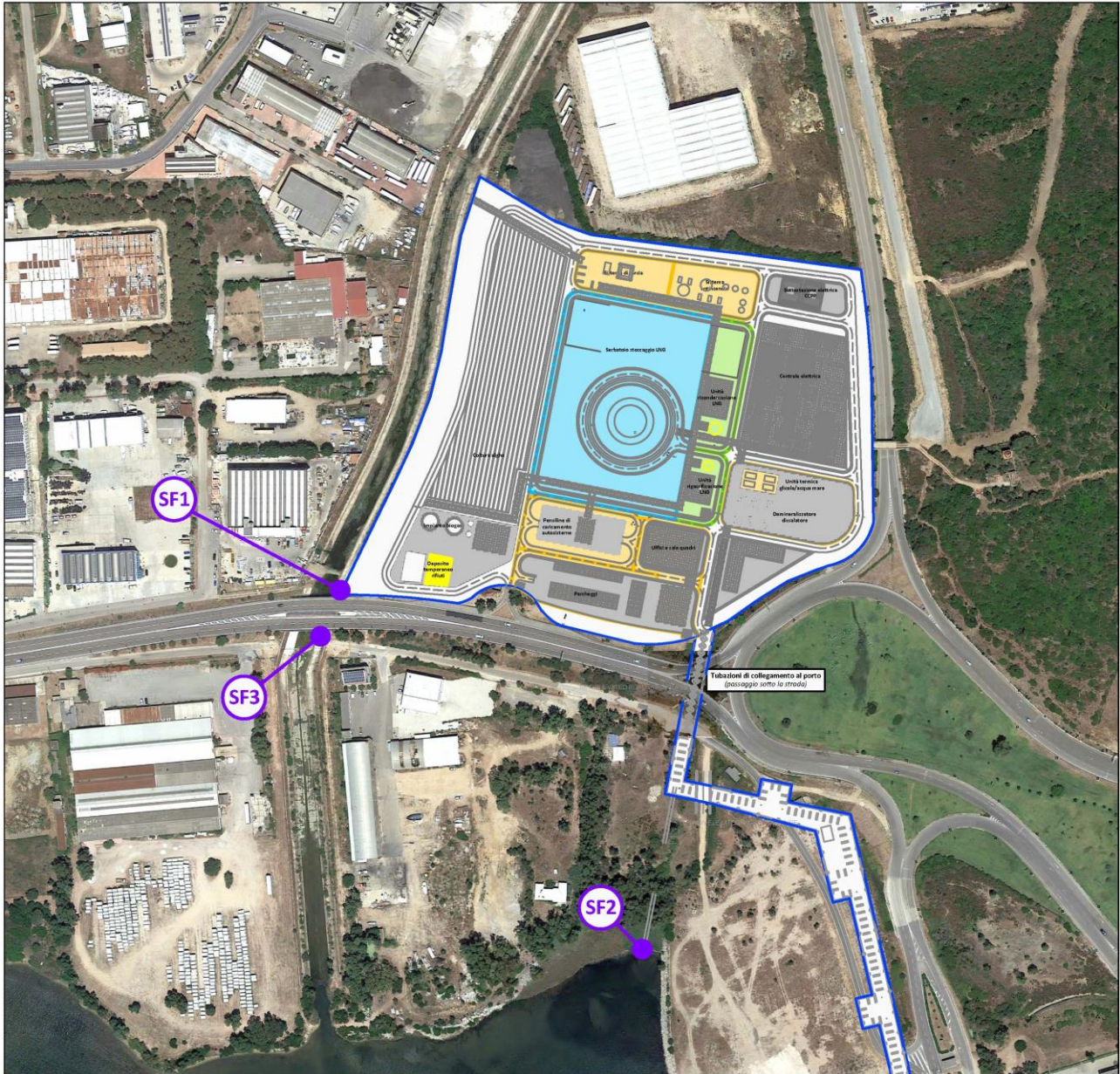
Figura III.11 – Ubicazione scarichi idrici
