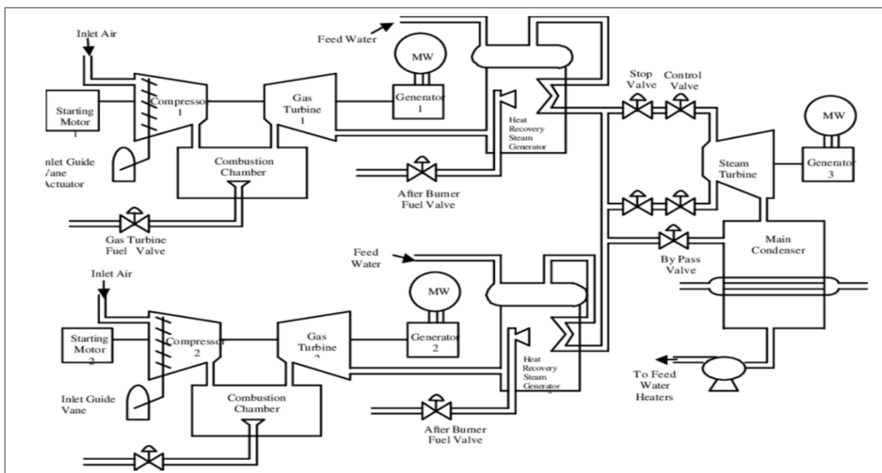
Figura III.5 – Schema a blocchi del Centrale elettrica a ciclo combinato
