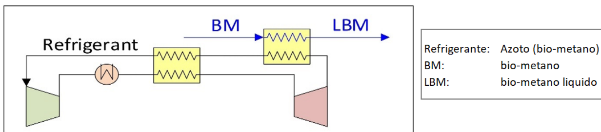
Figura III.4 – Schema liquefattore
