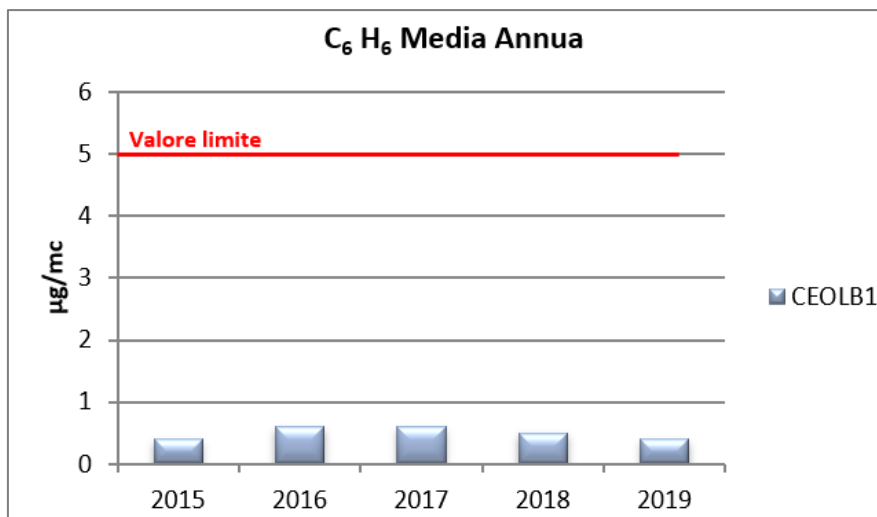
Figura IV.21 - Andamento della media annua del Benzene
