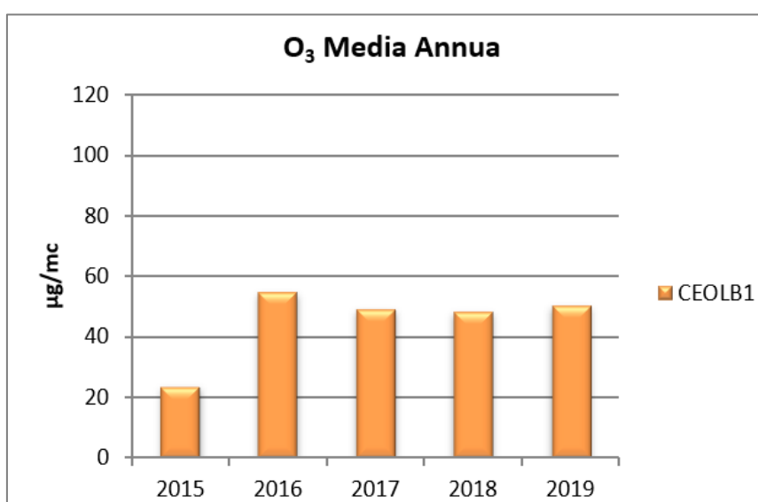
Figura IV.15 - Andamento media annua Ozono
