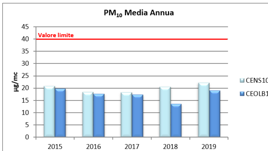
Figura IV.16 - Andamento media annua di PM10
