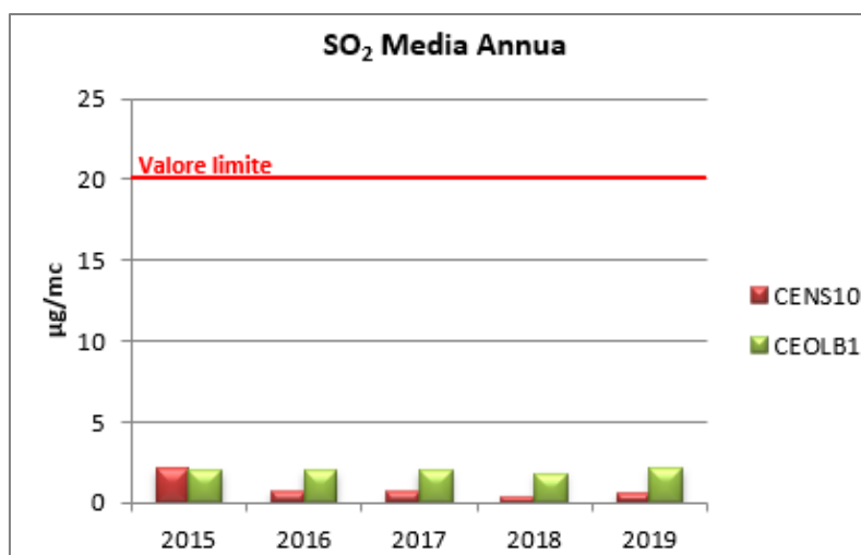
Figura IV.18 - Andamento media annua SO 2
