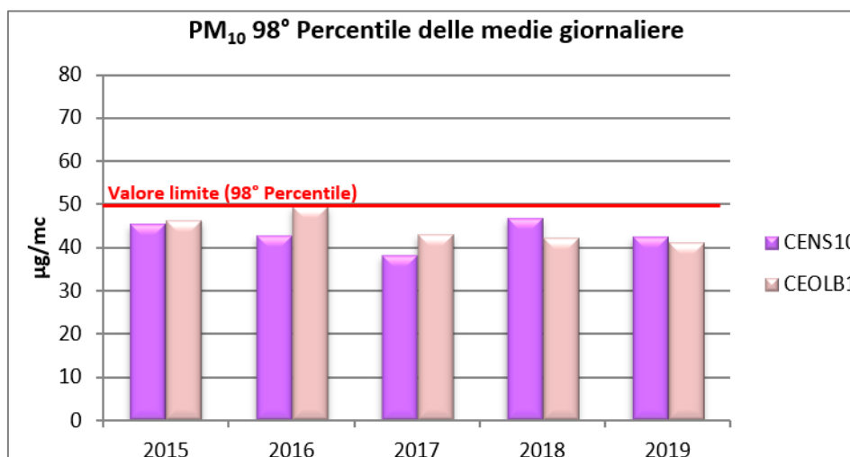
Figura IV.17 - Andamento 98° percentile delle medie giornaliere di PM10
