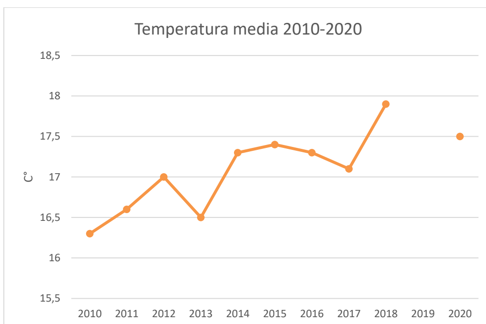
Figura IV.9 – Temperatura media 2010-2020
