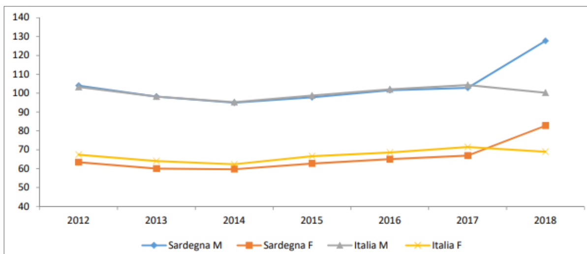
Figura IV.35 - Tasso standardizzato di mortalità (per 10.000 abitanti) in Sardegna e in Italia [Fonte: Istat – HFA]
