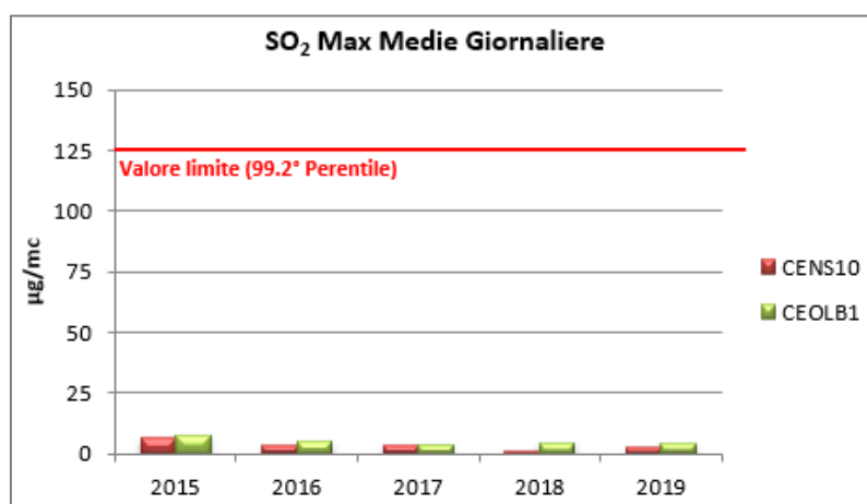
Figura IV.19 - Andamento massime medie giornaliere SO 2
