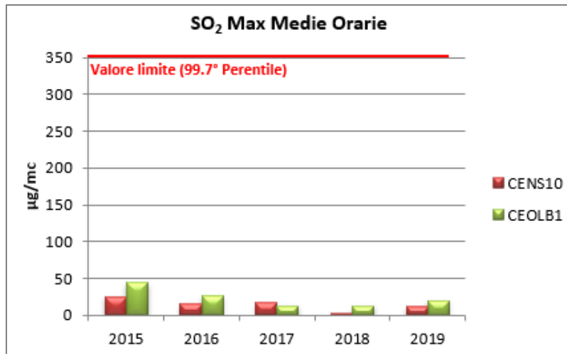
Figura IV.20 - Andamento massime medie orarie SO 2
