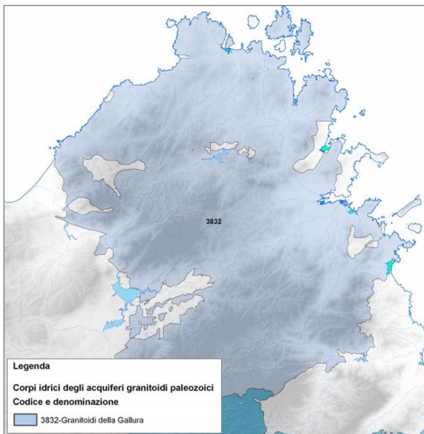
Figura IV.23 – Granitoidi della Gallura
