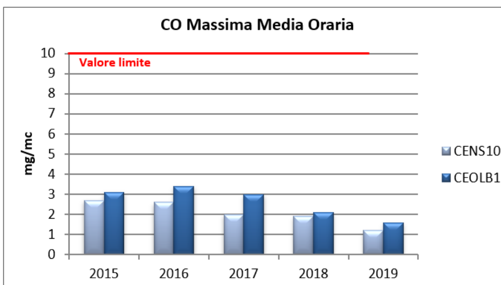
Figura IV.12 - Andamento massima media oraria CO
