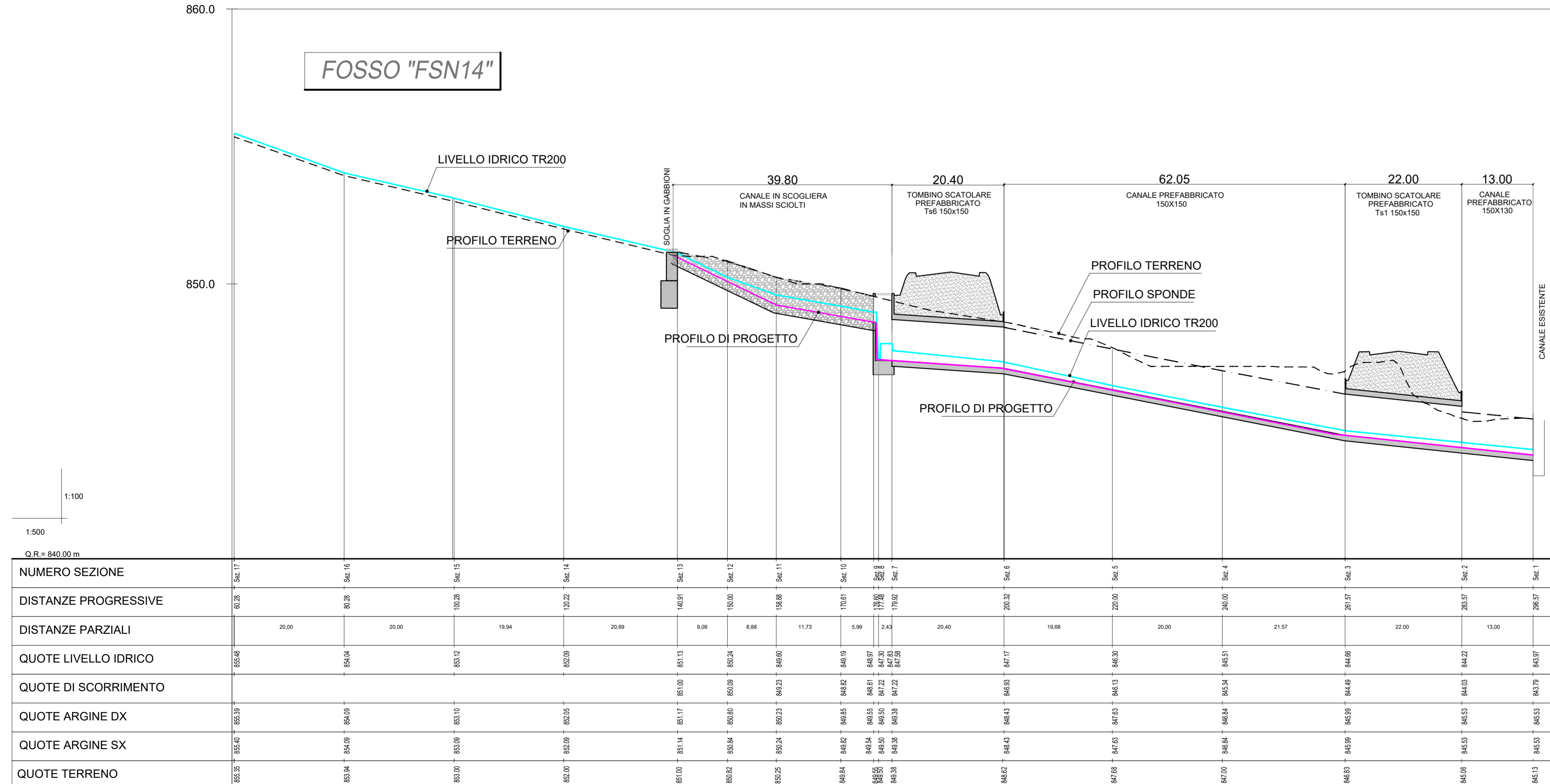
PROFILO LONGITUDINALE 1:500/100
