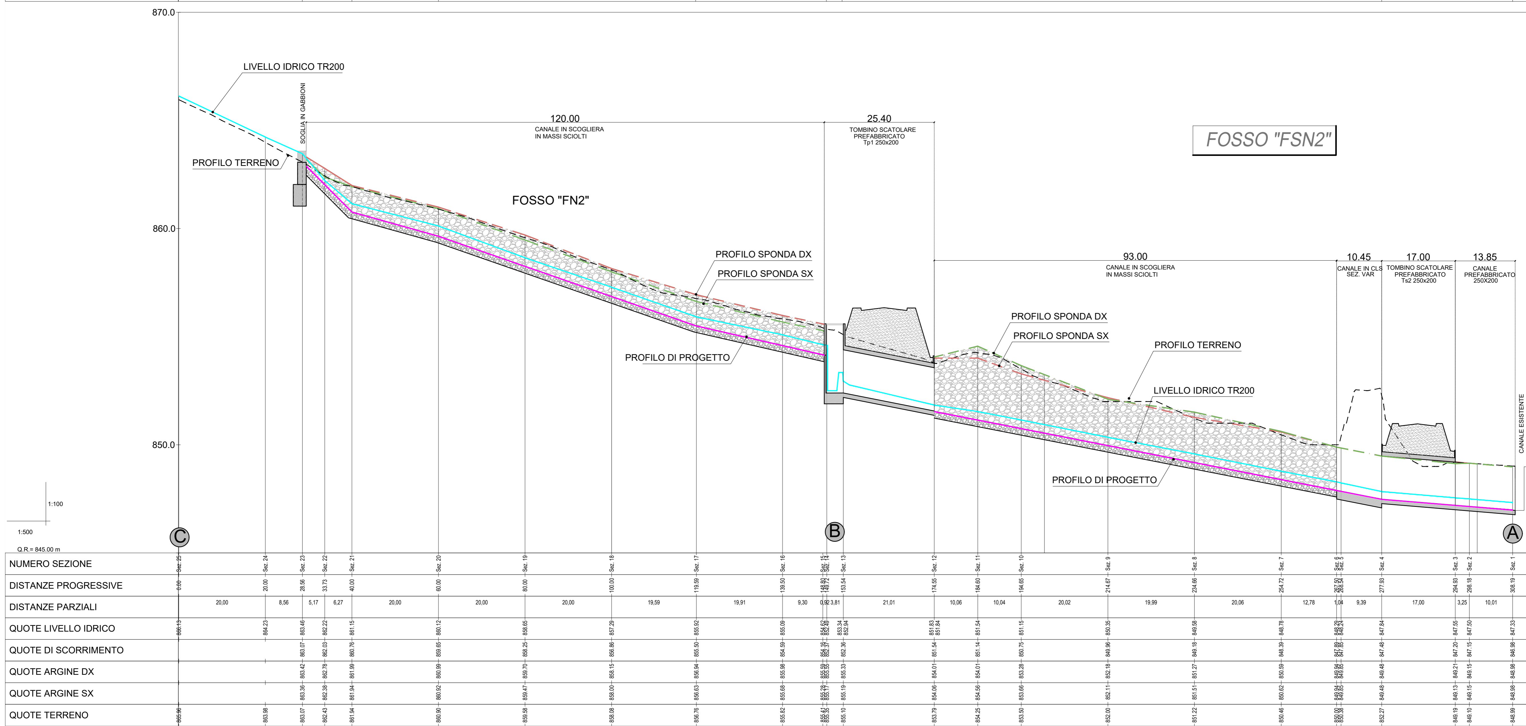
PROFILO LONGITUDINALE 1:500/100
