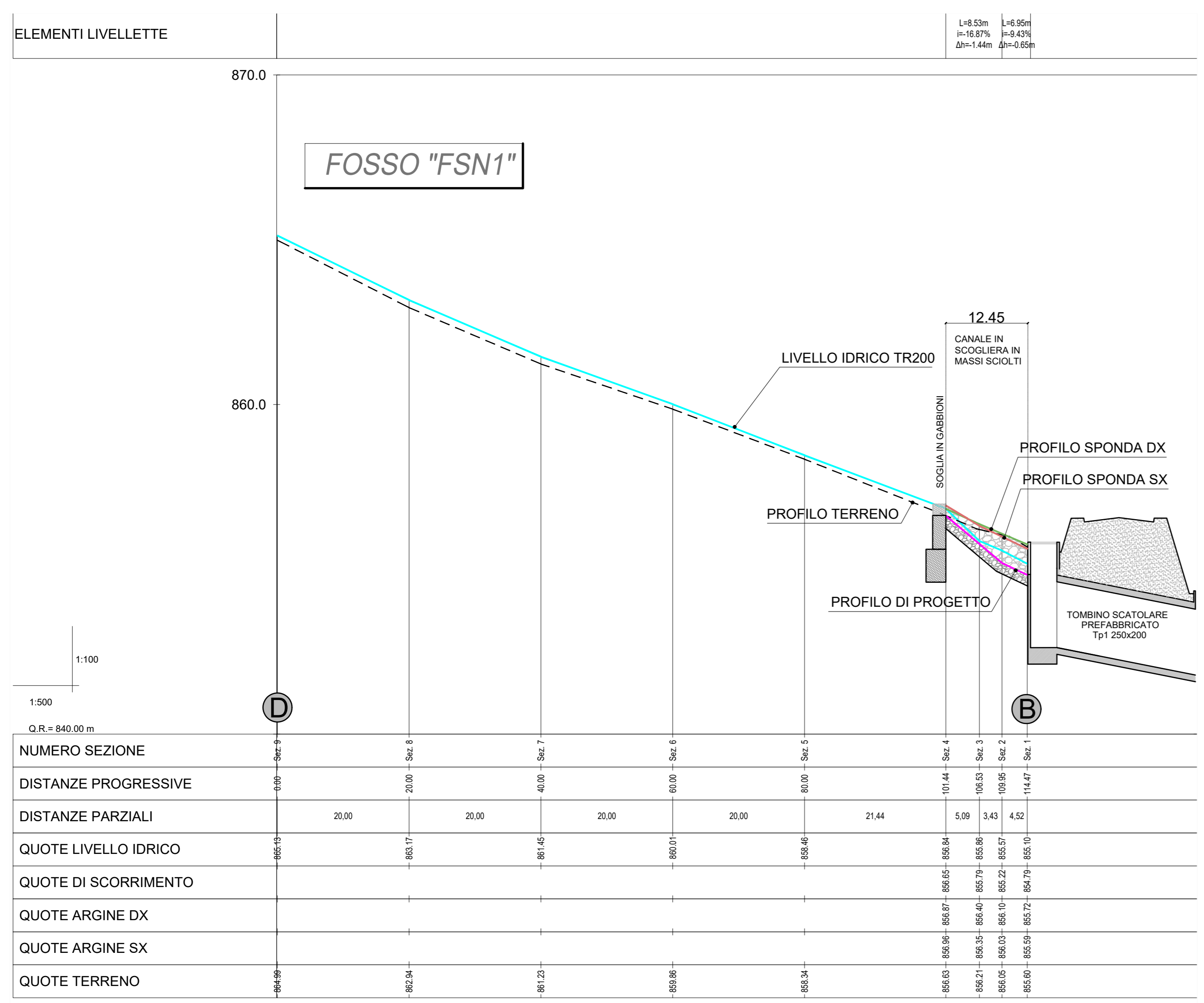
PROFILO LONGITUDINALE 1:500/100
