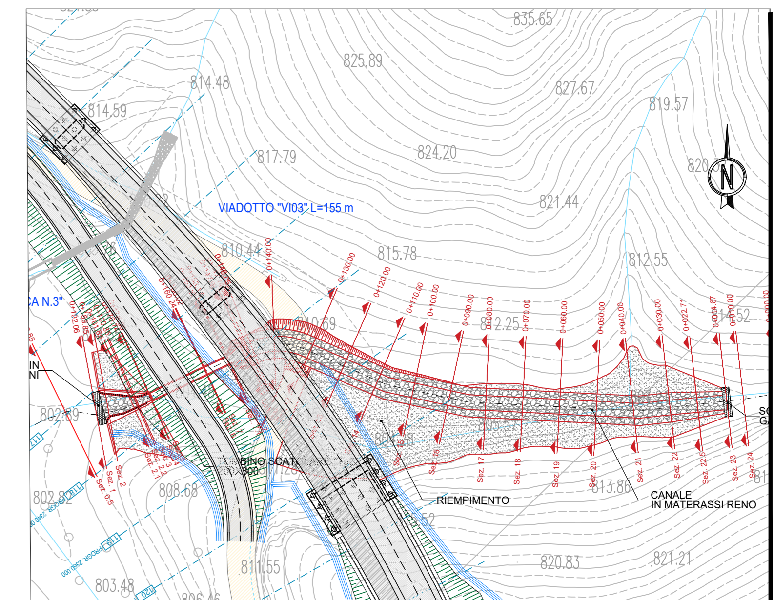
STRALCIO PLANIMETRICO 1:1.000
