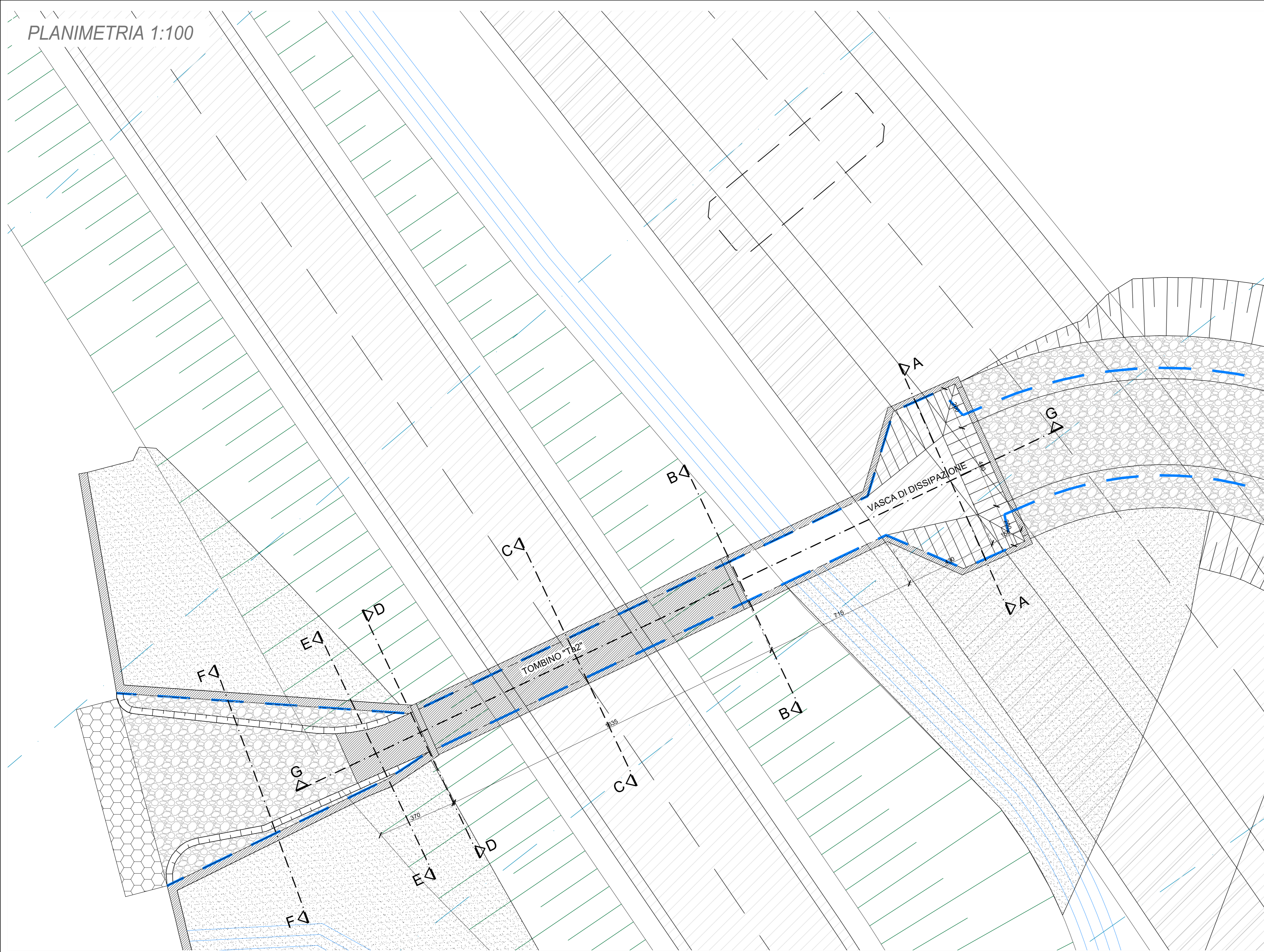
SEZIONE "G"- "G" VASCA DI DISSIPAZIONE E TOMBINO SCALA 1:100
