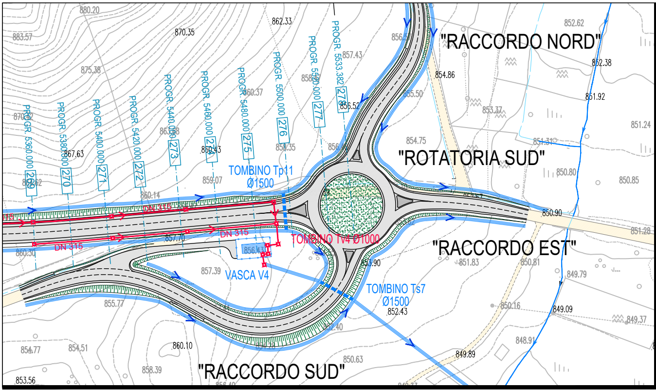
TOMBINO Tp11 - STRALCIO PLANIMETRICO 1:2.000
