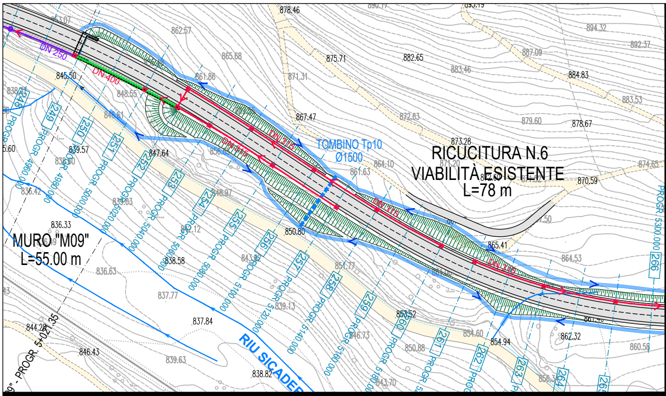
TOMBINO Tp10 - STRALCIO PLANIMETRICO 1:2.000
