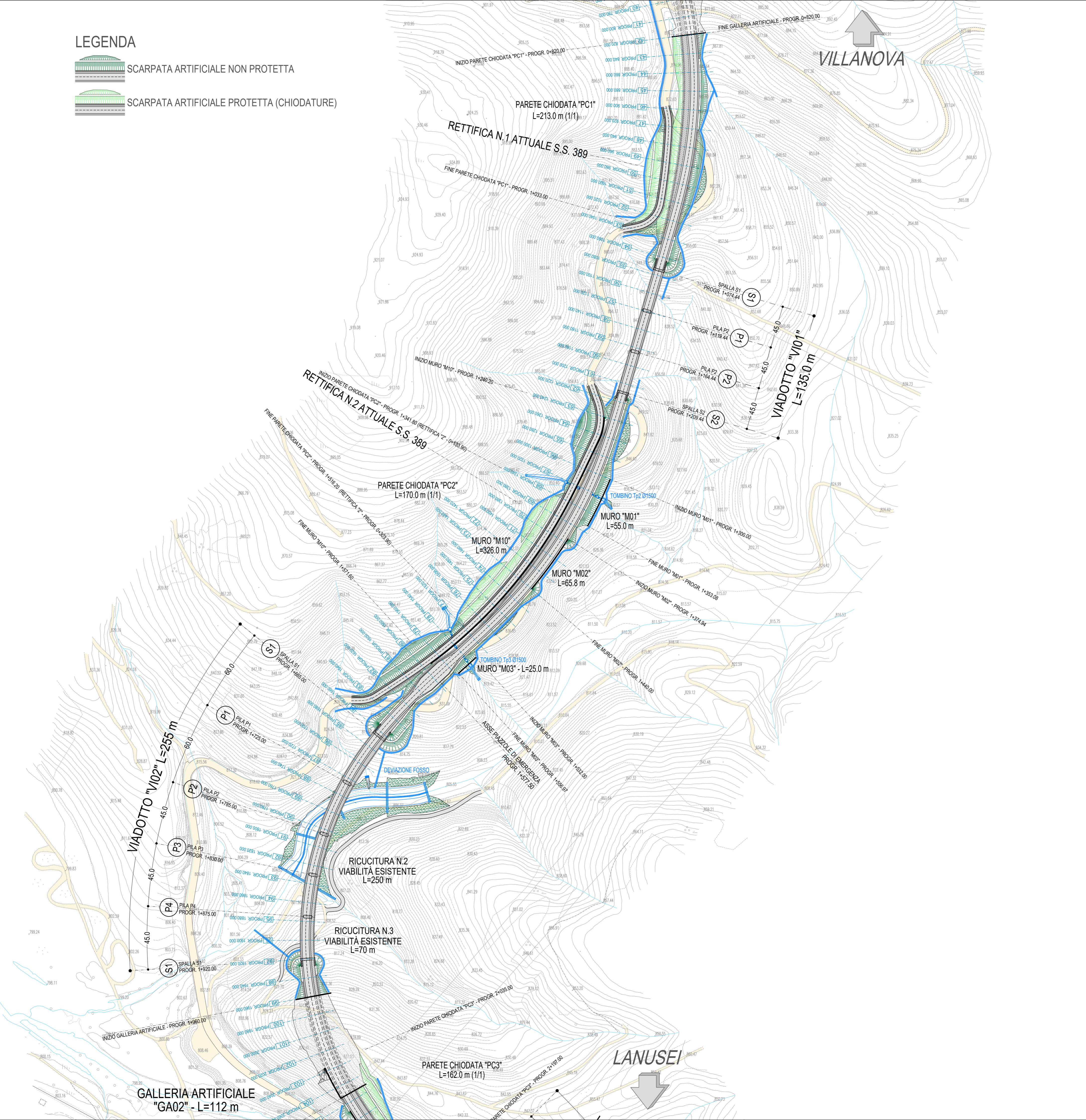
QUADRO DI UNIONE
