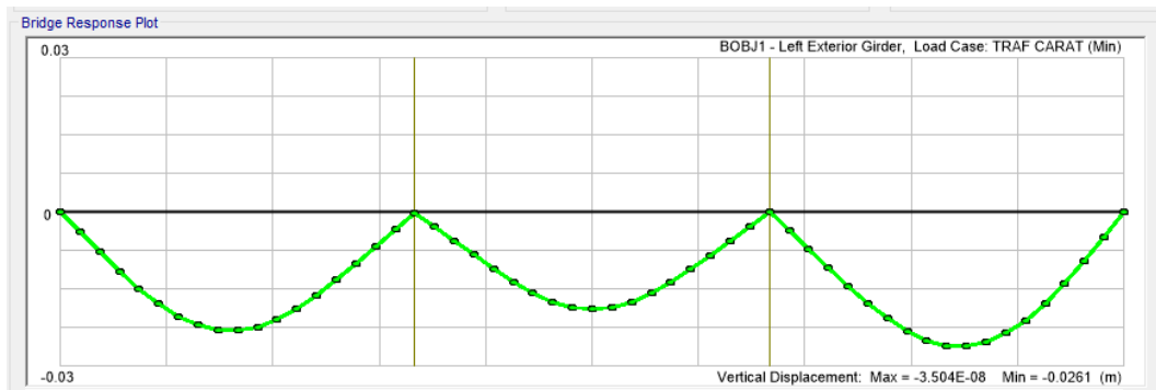
Figura 7.7 -. Abbassamento traffico 0.026m
