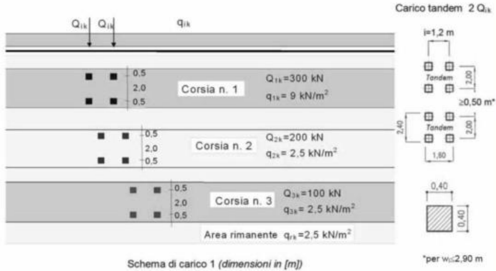
Figura 8.17 - Impronta di carico 1
