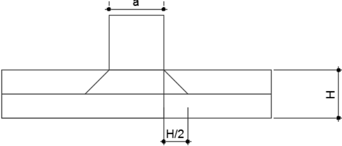
Figura 8.15 - Diffusione nella soletta
