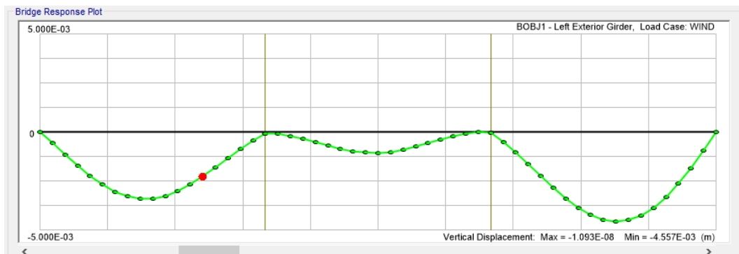
Figura 7.8 -. Abbassamento vento 0.0045m
