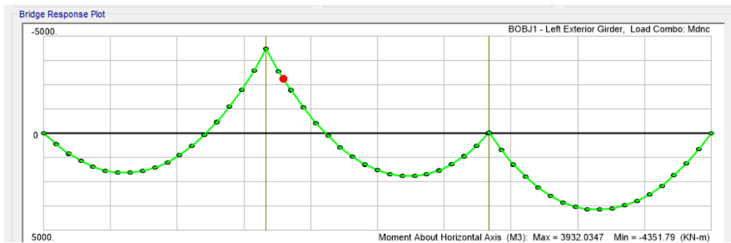
Figura 7.10 -. Momento flettente (kN*m)
