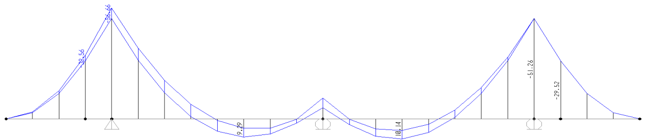
Figura 8.30 -diagramma momenti FASE 2
