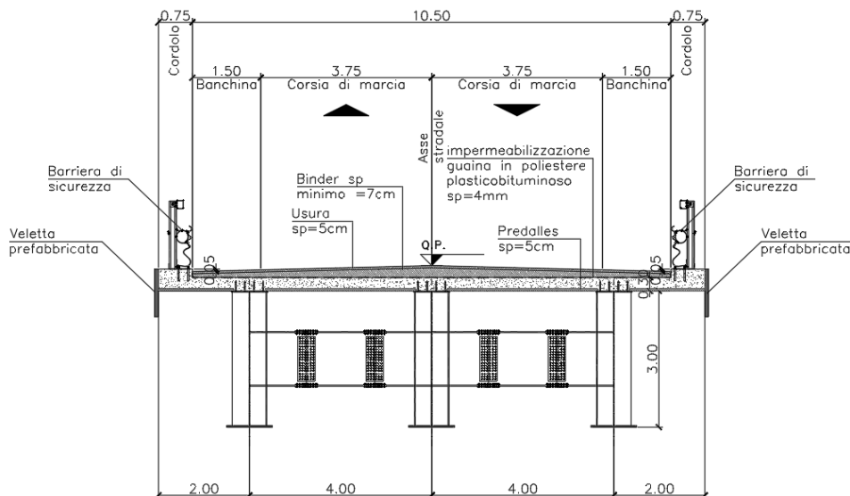
Figura 1.1 - Sezione trasversale dell'impalcato
