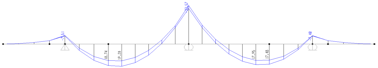
Figura 8.29 -diagramma momenti FASE 1
