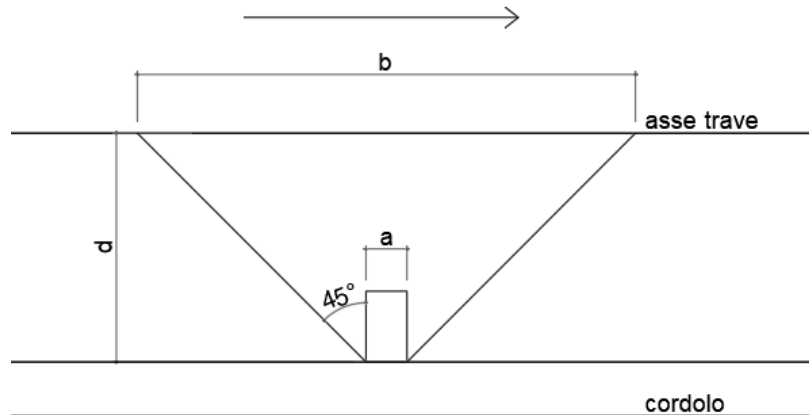
Figura 8.26 -. Schema diffusione carico
