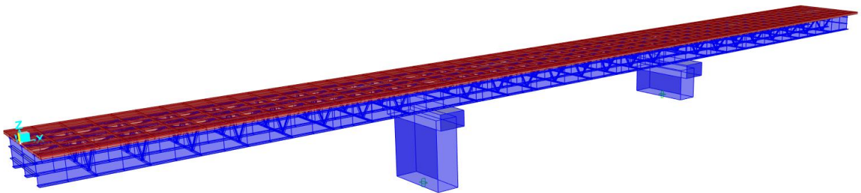
Figura 4.1 -. Modello di FEM
