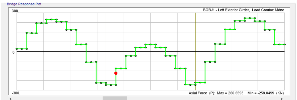
Figura 6.7 -. Sforzo Normale (kN)
