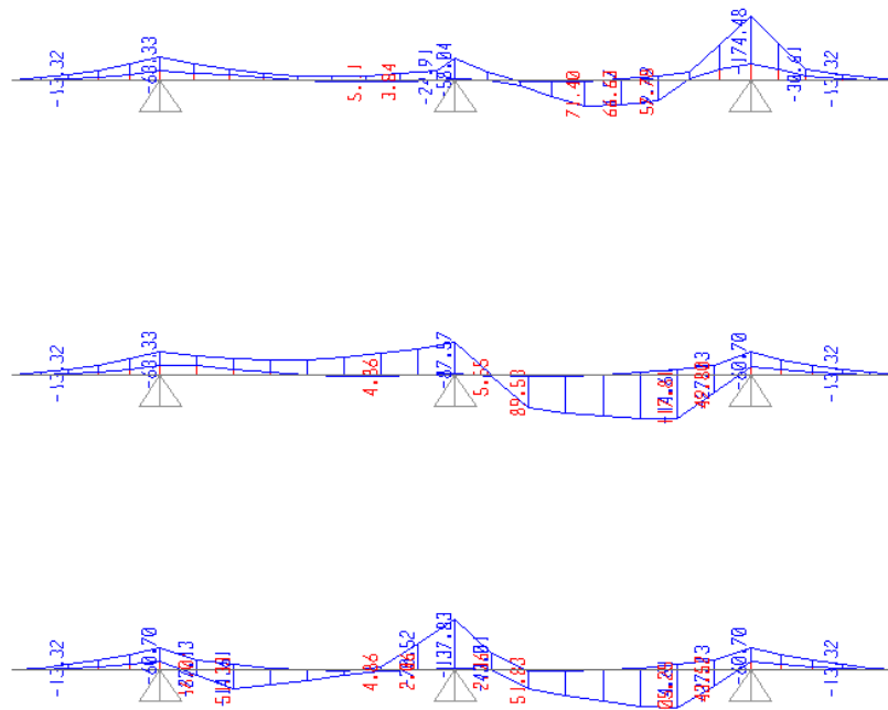
Figura 8.23 - involucro momento flettente SLU
