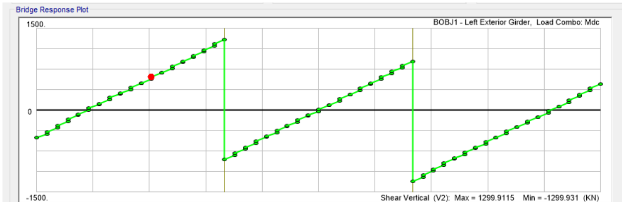
Figura 6.9 -. Taglio (kN)
