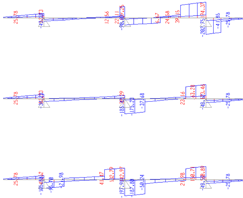
Figura 8.24 - involucro taglio SLU
