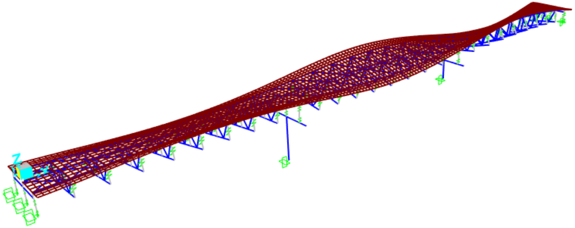
Figura 6.2 - Modo 2
