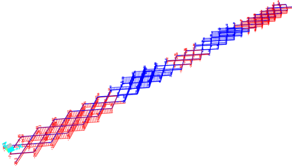
Figura 8.12 -. Sforzo Normale (kN)
