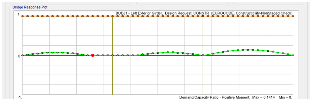
Figura 7.11 -. Verifica momento positivo
