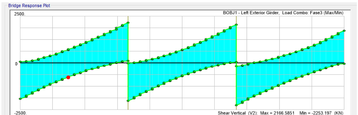
Figura 6.12 -. Taglio (kN)
