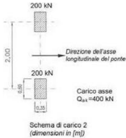
Figura 8.18 - Impronta di carico 2
