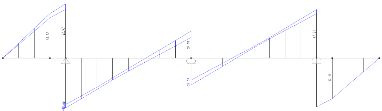
Figura 8.32 -diagramma taglio FASE 2
