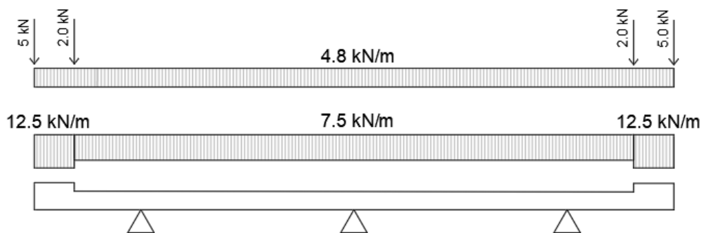
Figura 8.14 -. Carichi permanenti
