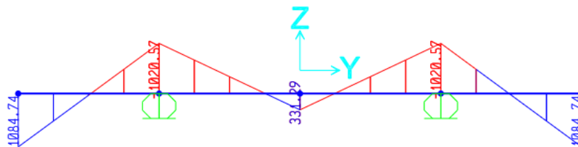
Figura 8.7 -. Momento flettente (kN*m)
