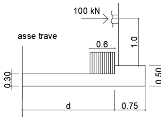
Figura 8.27 -. Schema applicazione carico
