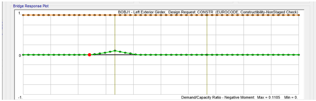
Figura 7.12 - Verifica momento negativo
