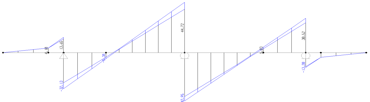
Figura 8.31 -diagramma taglio FASE 1
