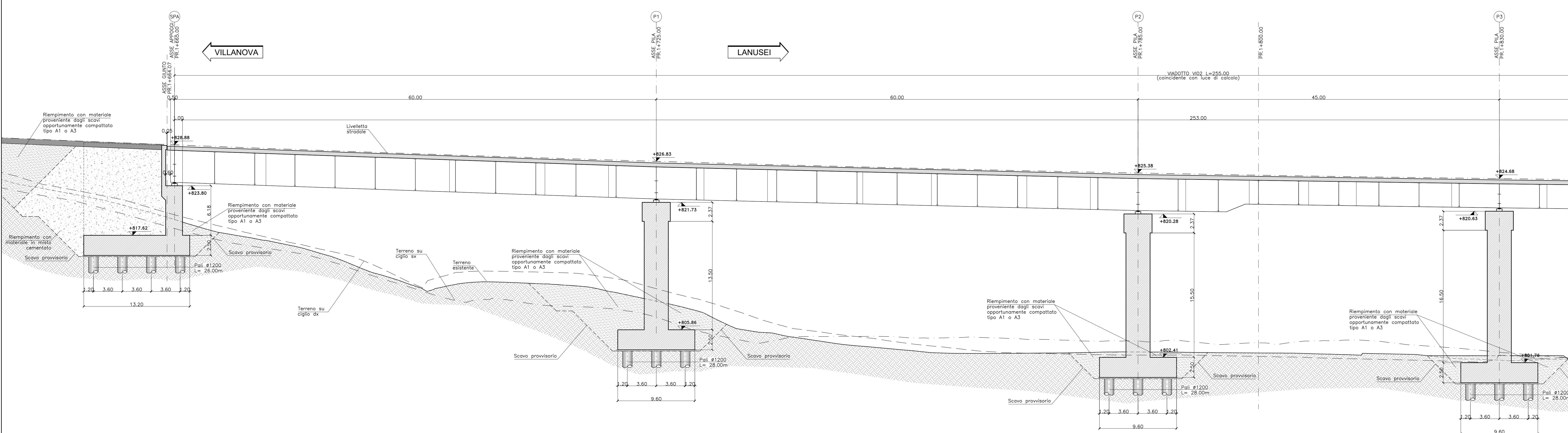
SEZIONE LONGITUDINALE IN ASSE STRADALE SCALA 1:200
