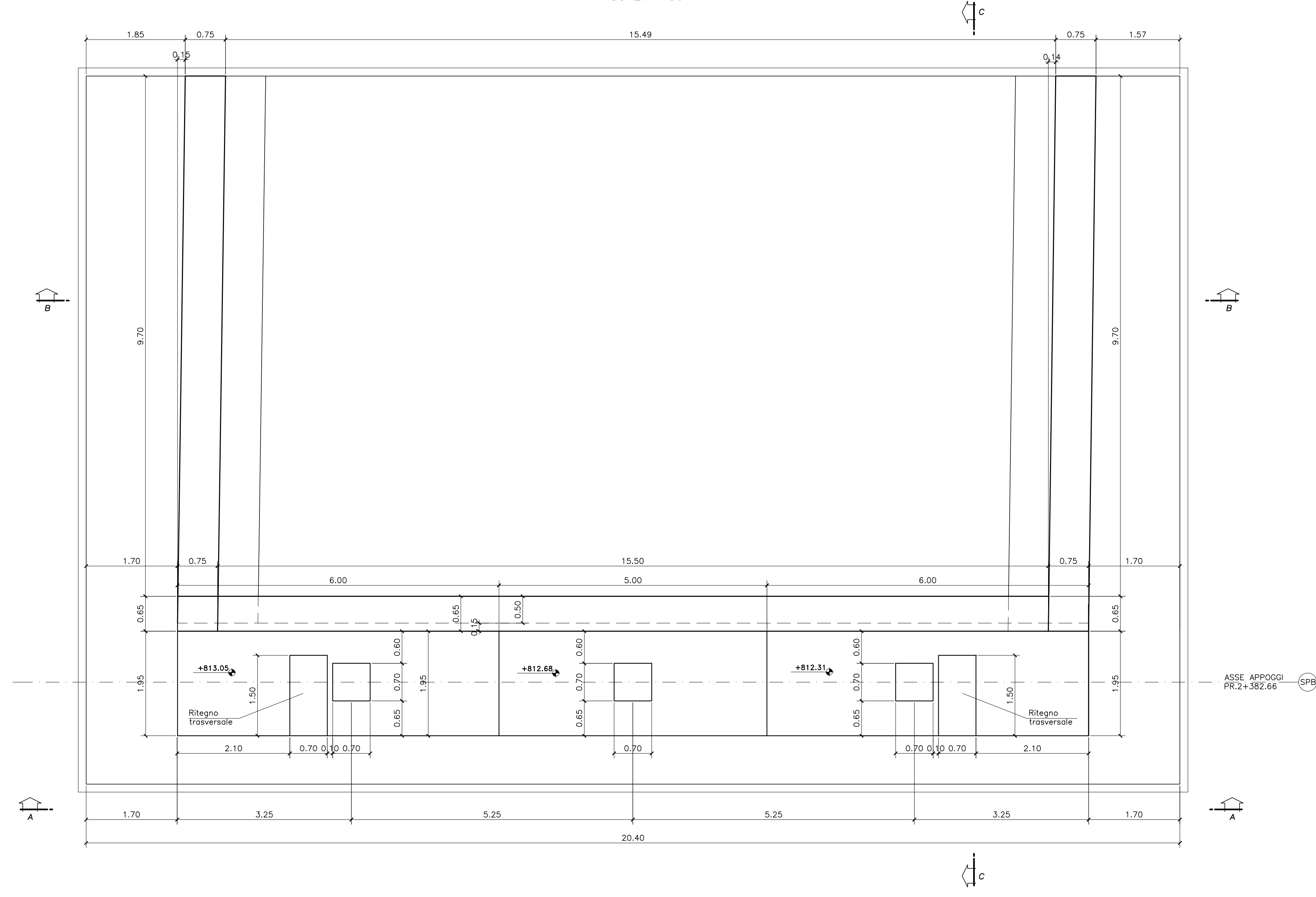
VISTA DALL'ALTO SCALA 1:50
