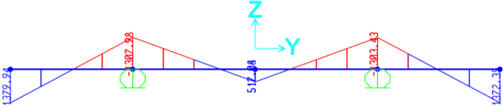
Figura 8.4 -. Momento flettente (kN*m)
