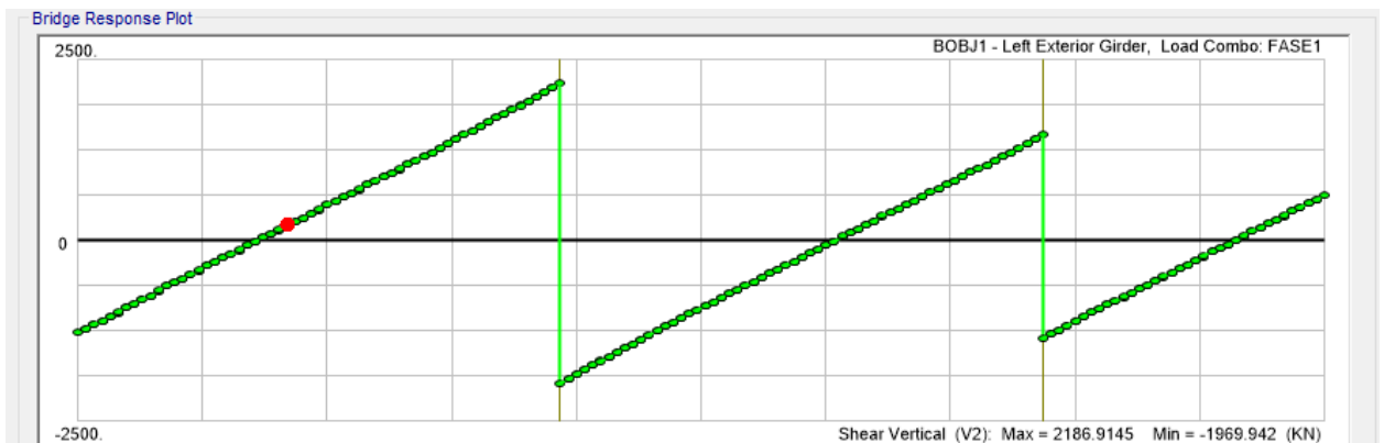
Figura 6.6 -. Taglio (kN)
