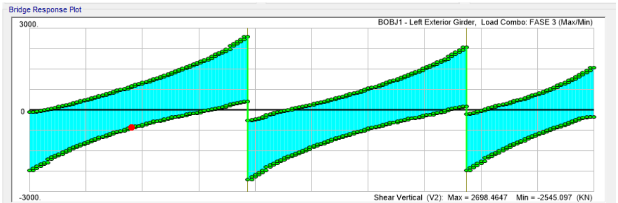
Figura 6.12 -. Taglio (kN)
