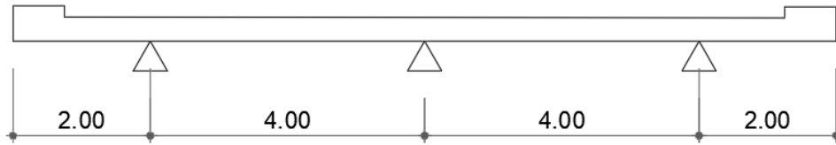
Figura 8.9 - Schema statico
