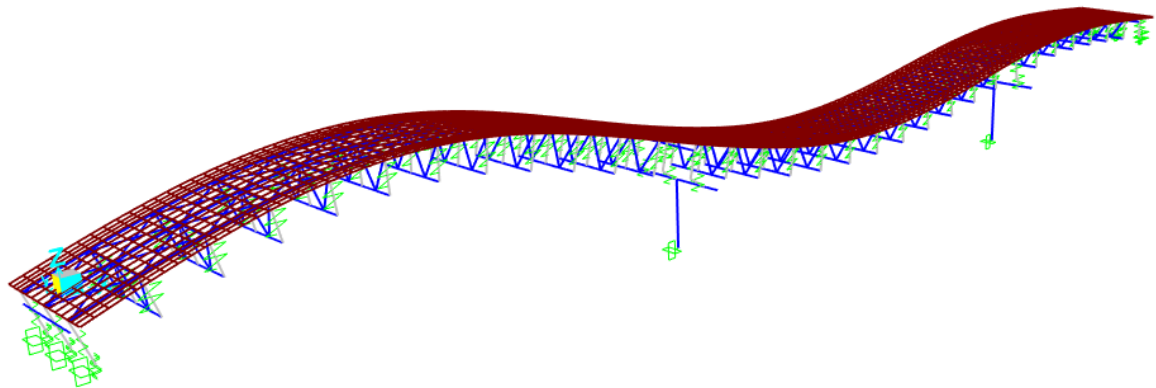
Figura 6.1 - . Modo 1
