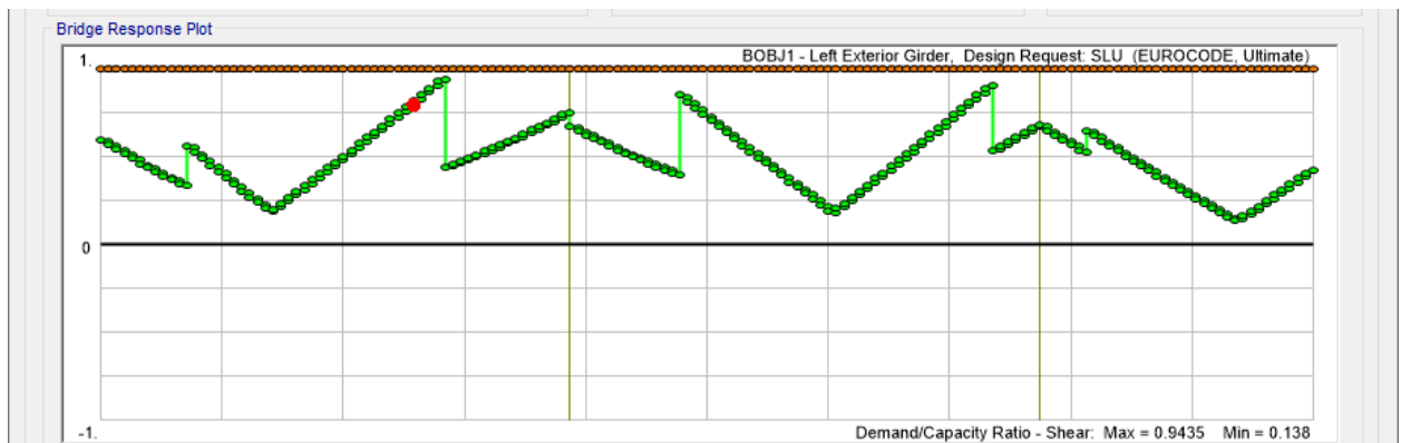
Figura 6.16 -. Verifica taglio
