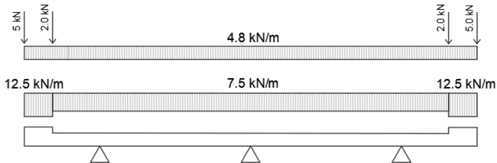
Figura 8.10 - Carichi permanenti
