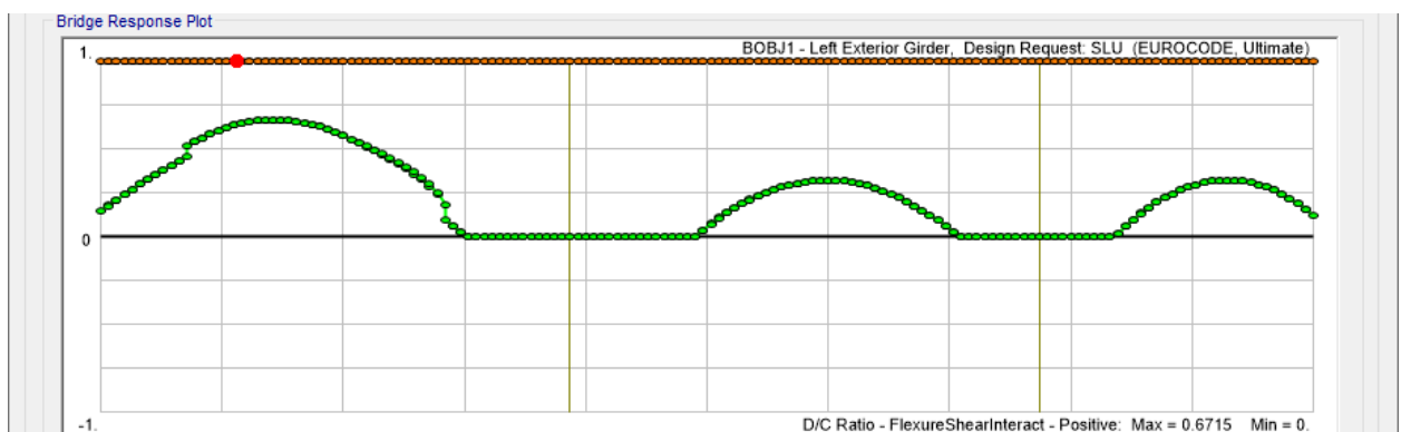
Figura 6.17 -. Verifica interazione taglio/momento positivo
