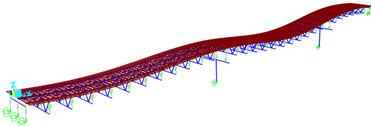
Figura 6.3 - Modo 3
