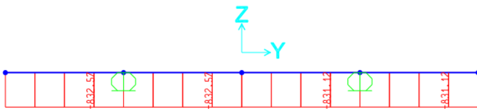
Figura 8.6 -. Sforzo Normale (kN)
