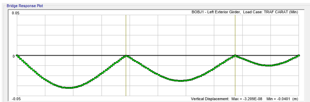
Figura 7.7 -. Abbassamento traffico 0.04m
