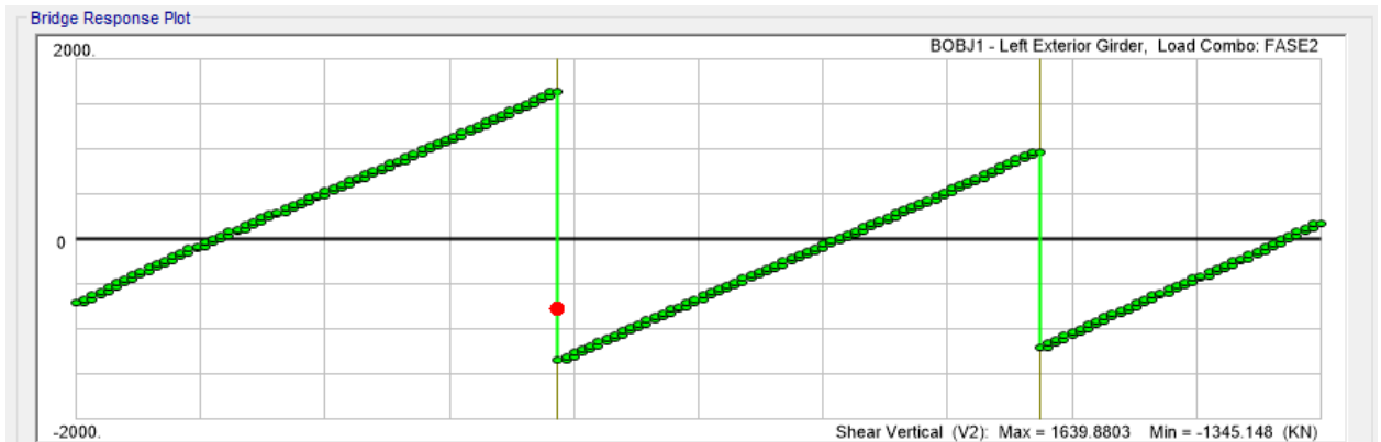
Figura 6.9 -. Taglio (kN)
