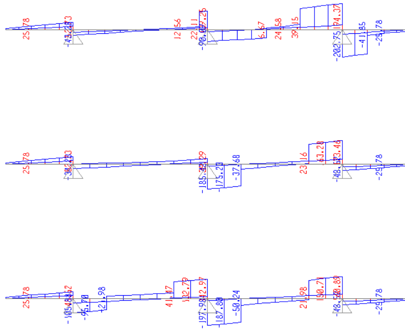
Figura 8.20 - involuppo taglio SLU
