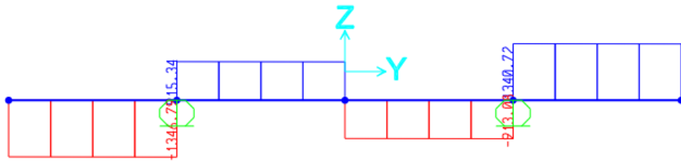
Figura 8.5 -. Taglio (kN)
