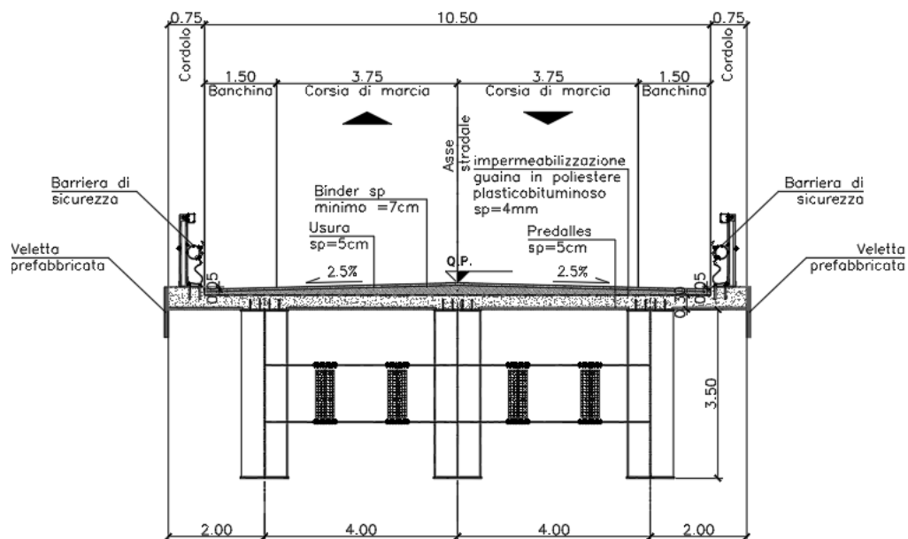
Figura 1.1 - Sezione trasversale dell'impalcato – campata 60m
