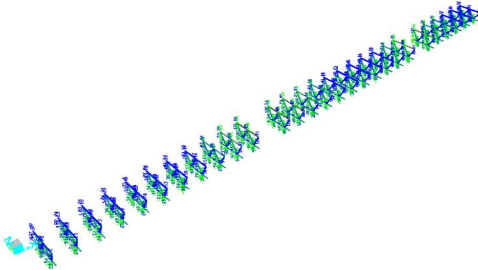
Figura 8.7 -. Sforzo Normale (kN)
