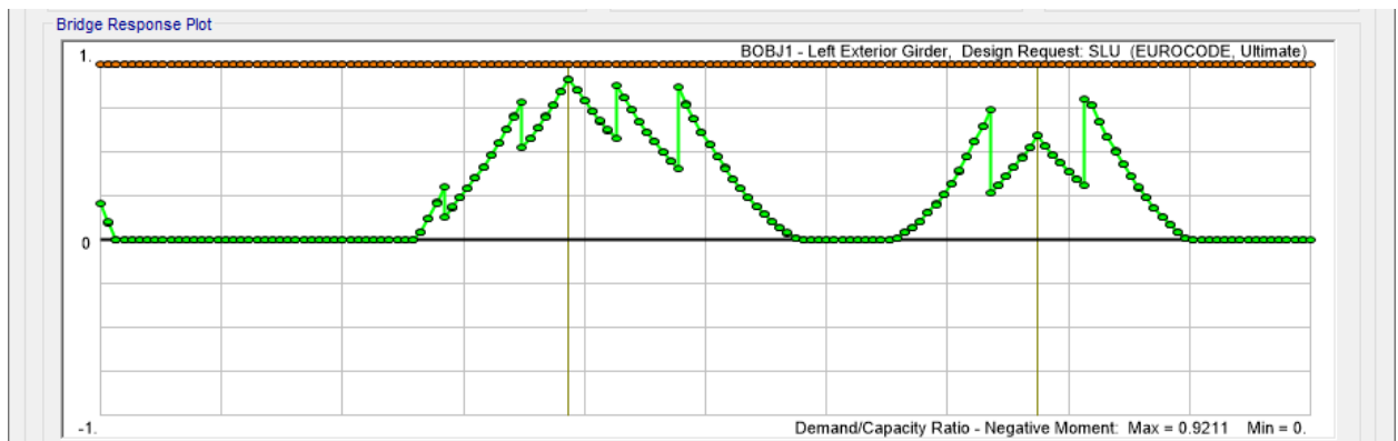
Figura 6.15 -. Verifica momento negativo
