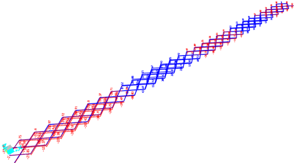
Figura 8.8 -. Sforzo Normale (kN)
