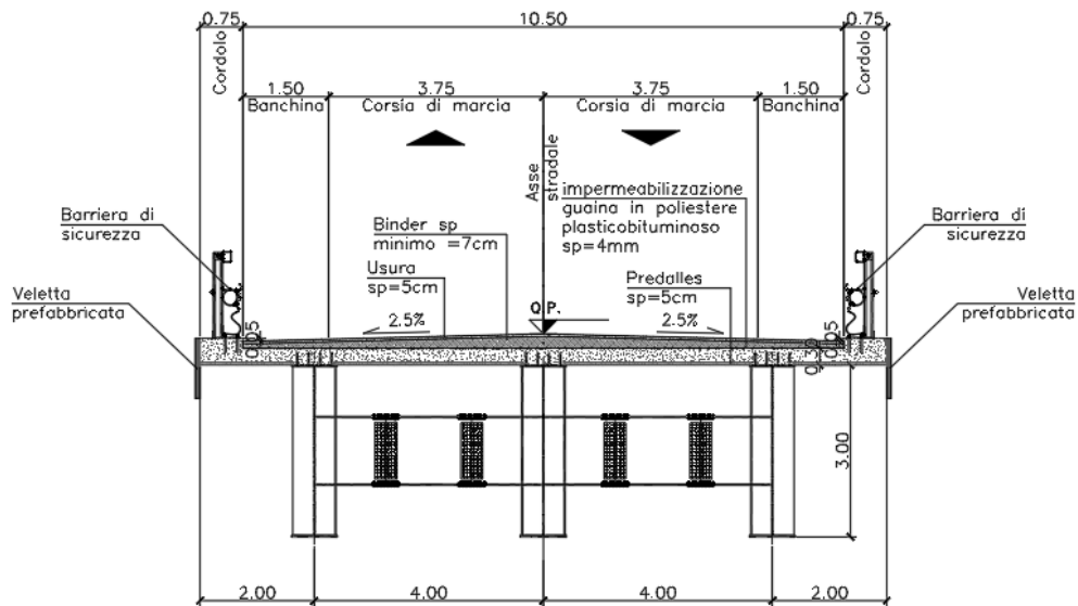
Figura 1.2 - Sezione trasversale dell'impalcato – campata 35m
