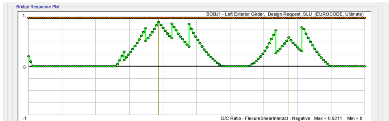
Figura 6.18 -. Verifica interazione taglio/momento negativo
