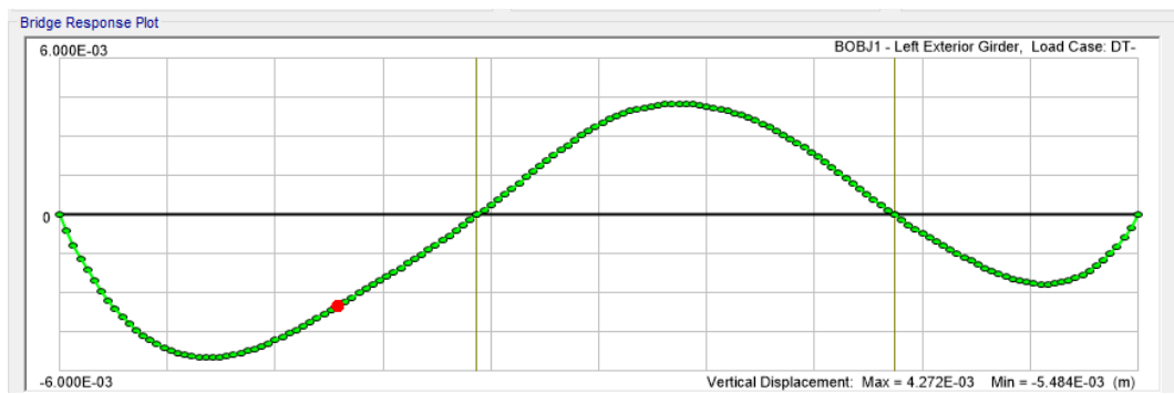
Figura 7.9 -. Abbassamento temperatura 0.0055m
