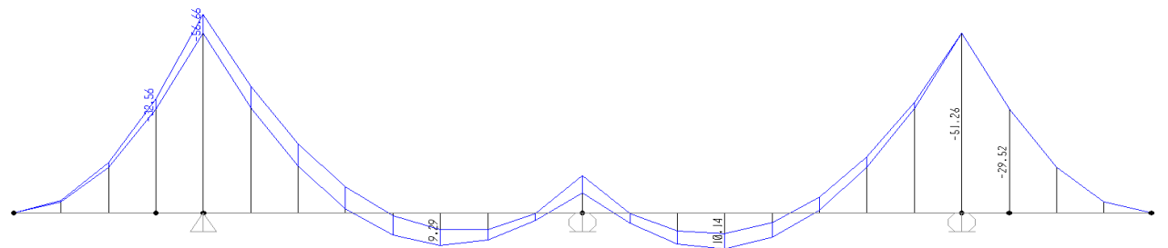
Figura 8.26 -diagramma momenti FASE 2
