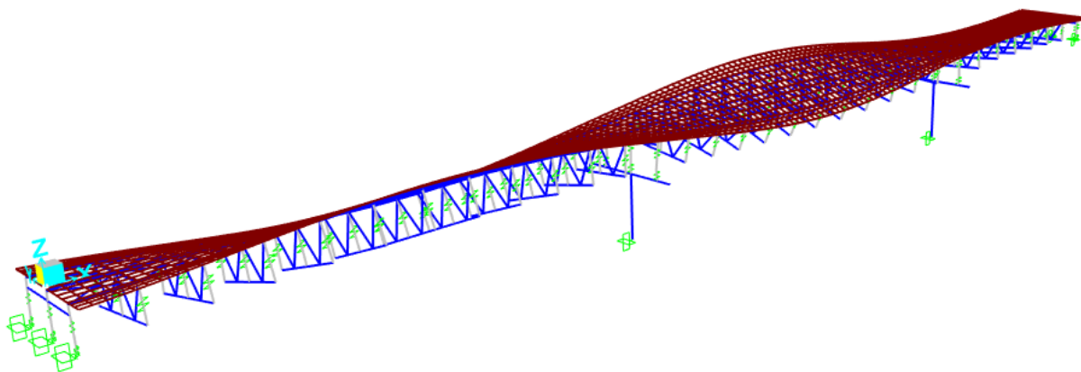
Figura 6.2 - Modo 2
