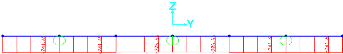
Figura 8.5 - Taglio (kN)
