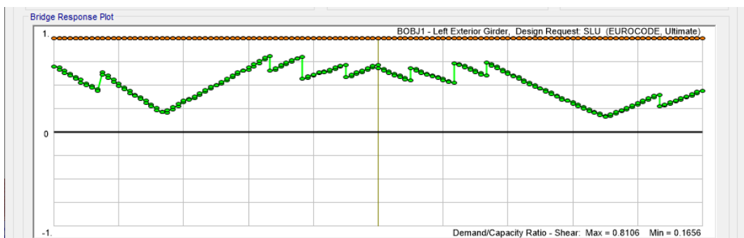
Figura 6.16 -. Verifica taglio
