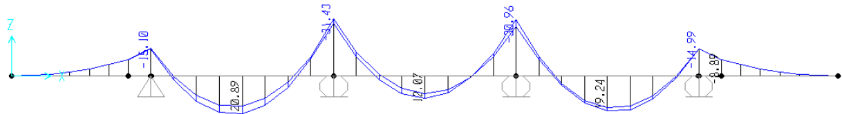
Figura 8.25 -diagramma momenti FASE 1
