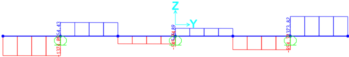
Figura 8.5 - Taglio (kN)
