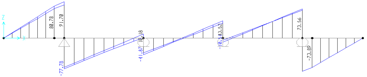
Figura 8.28 -diagramma taglio FASE 2
