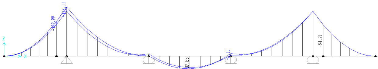
Figura 8.26 -diagramma momenti FASE 2
