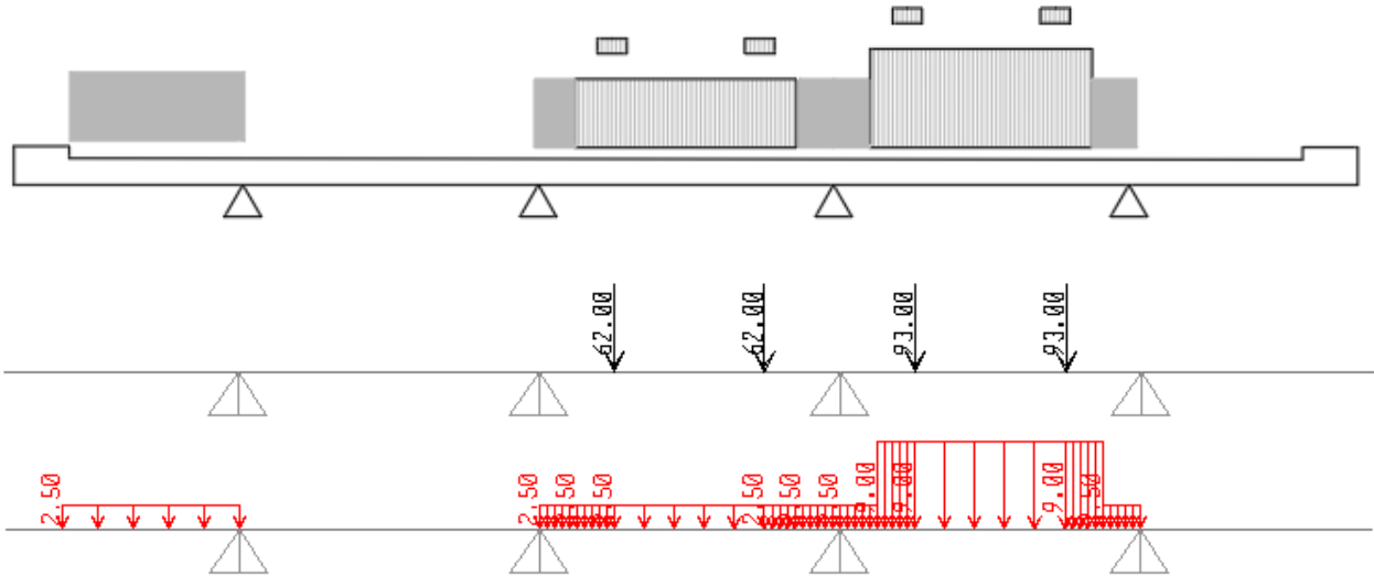
Figura 8.18 -. Condizione di carico 3
