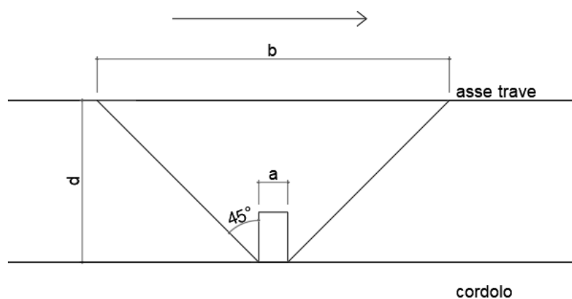
Figura 8.22 -. Schema diffusione carico
