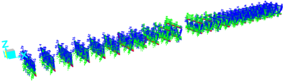
Figura 8.7 - Sforzo Normale (kN)
