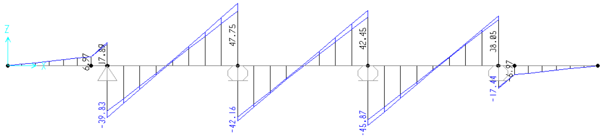
Figura 8.27 -diagramma taglio FASE 1
