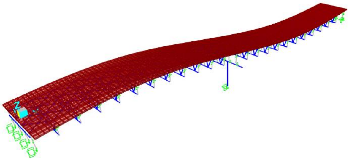
Figura 6.1 - . Modo 1
