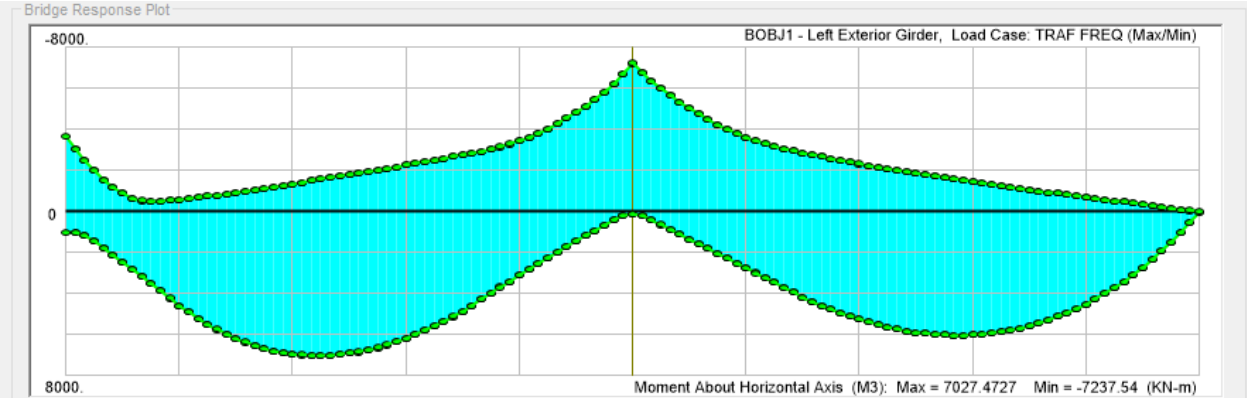
Figura 7.5 -. Momento flettente (kN*m)
