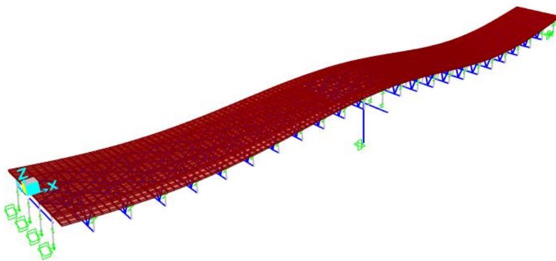
Figura 6.2 - Modo 2
