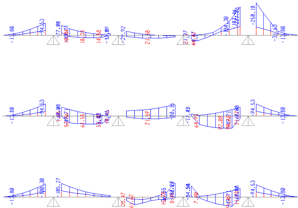
Figura 8.19 - involuppo momento flettente SLU
