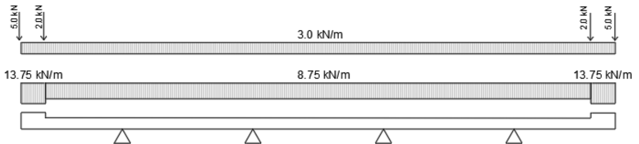
Figura 8.10 -. Carichi permanenti
