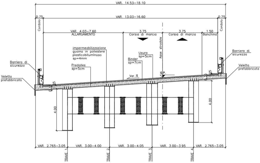
Figura 1.1 - Sezione trasversale dell’impalcato – 1° impalcato
