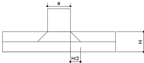
Figura 8.11 -. Diffusione nella soletta
