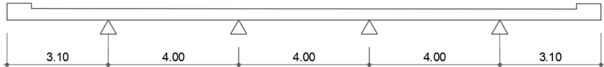
Figura 8.9 -. Schema statico
