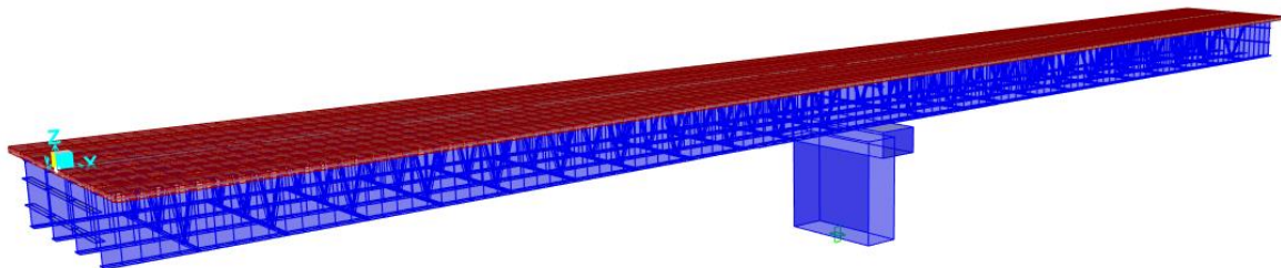
Figura 4.1 -. Modello di FEM
