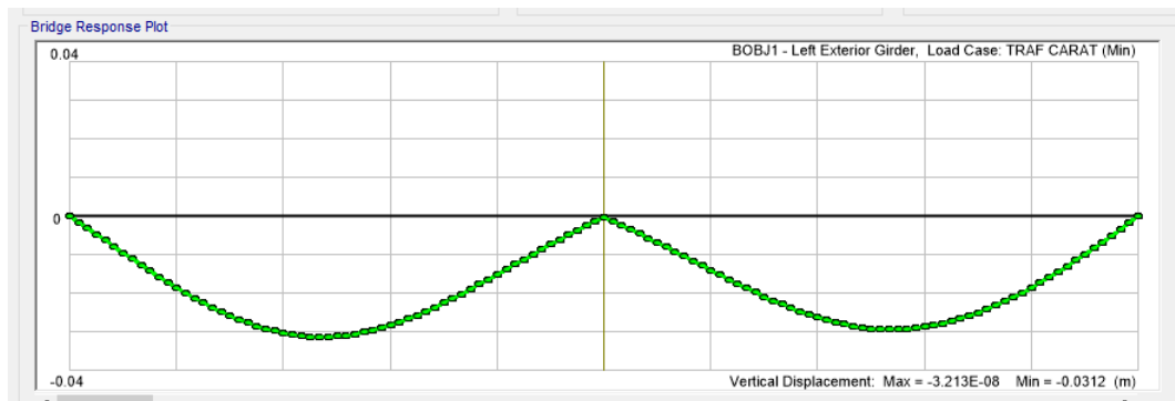
Figura 7.7 -. Abbassamento traffico 0.032m
