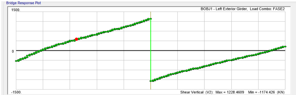
Figura 6.9 -. Taglio (kN)
