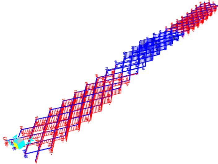
Figura 8.8 -. Sforzo Normale (kN)
