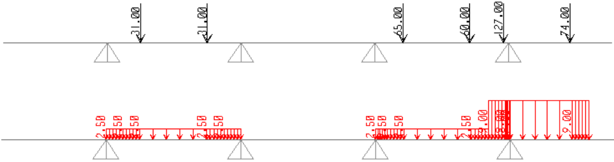
Figura 8.16 -. Condizione di carico 1
