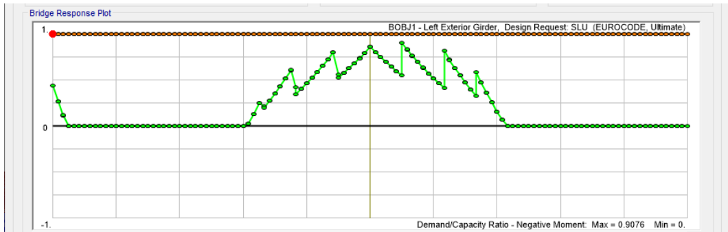
Figura 6.15 -. Verifica momento negativo
