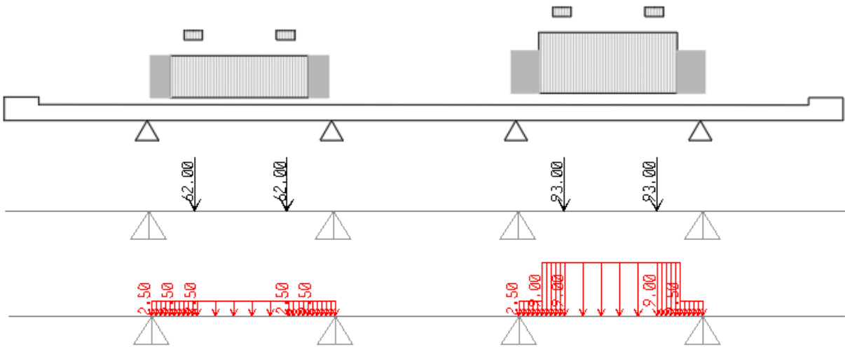
Figura 8.17 -. Condizione di carico 2
