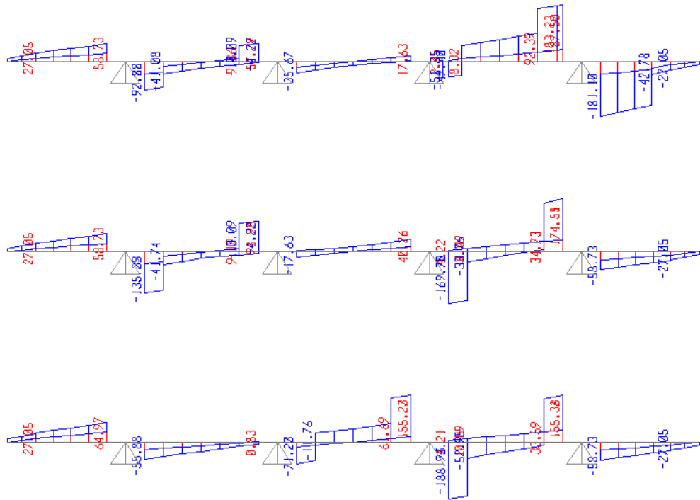
Figura 8.20 - involucro taglio SLU
