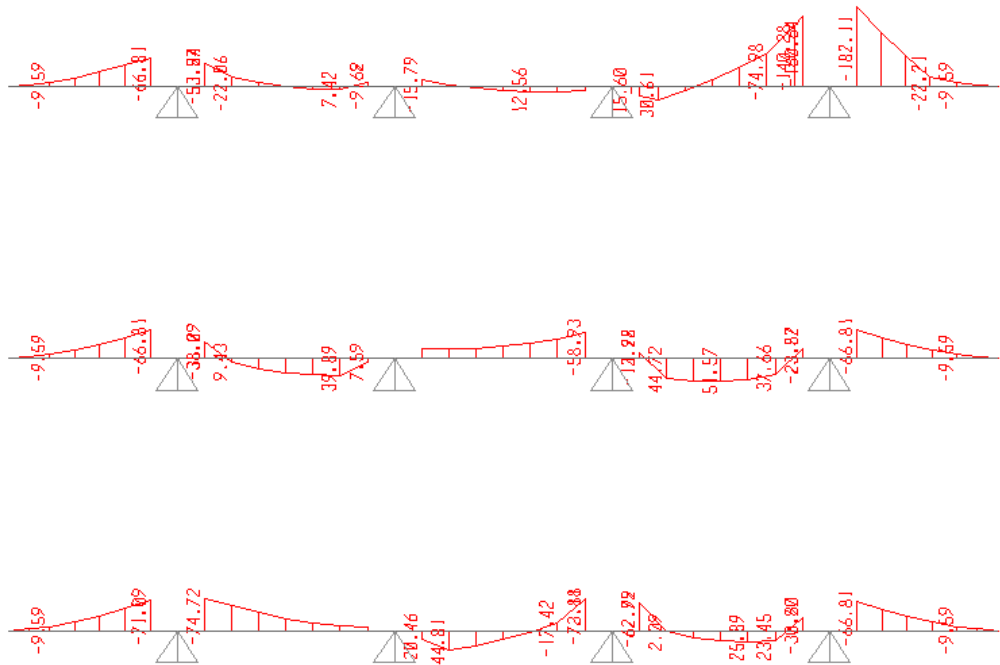
Figura 8.21 - involucro momento flettente SLE -rara
