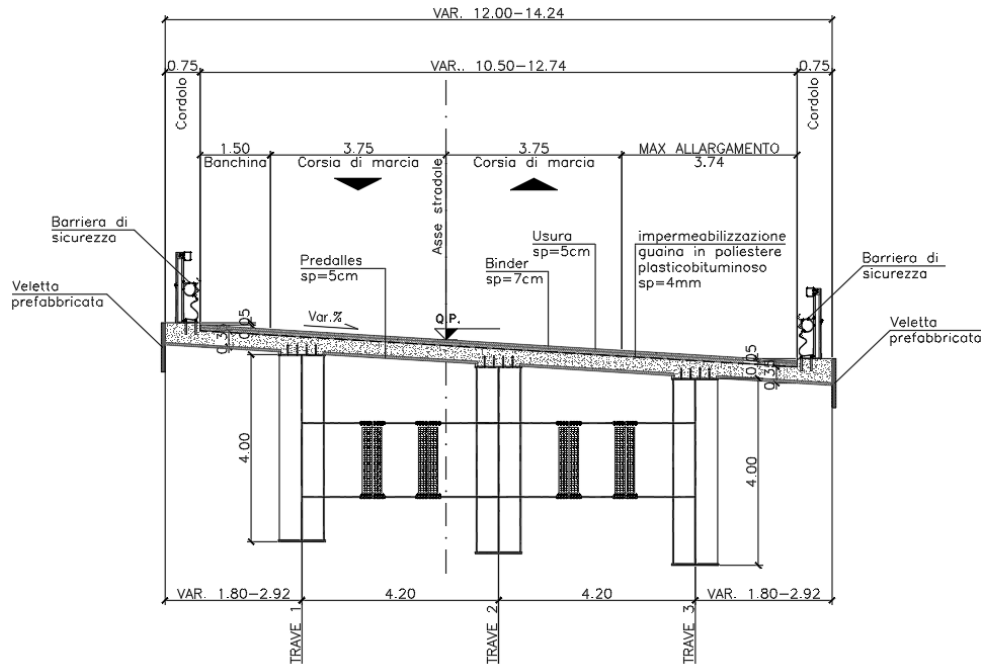
Figura 1.2 - Sezione trasversale dell'impalcato – 2° impalcato
