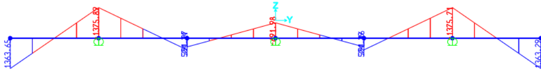
Figura 8.4 - Momento flettente (kN*m)
