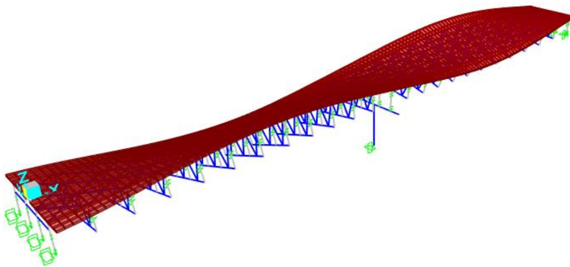
Figura 6.2 - Modo 2
