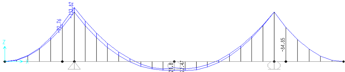
Figura 8.27 -diagramma taglio FASE 1
