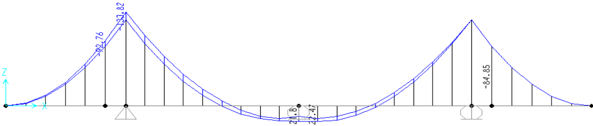
Figura 8.26 -diagramma momenti FASE 2
