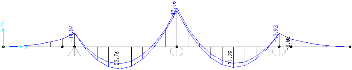
Figura 8.25 -diagramma momenti FASE 1
