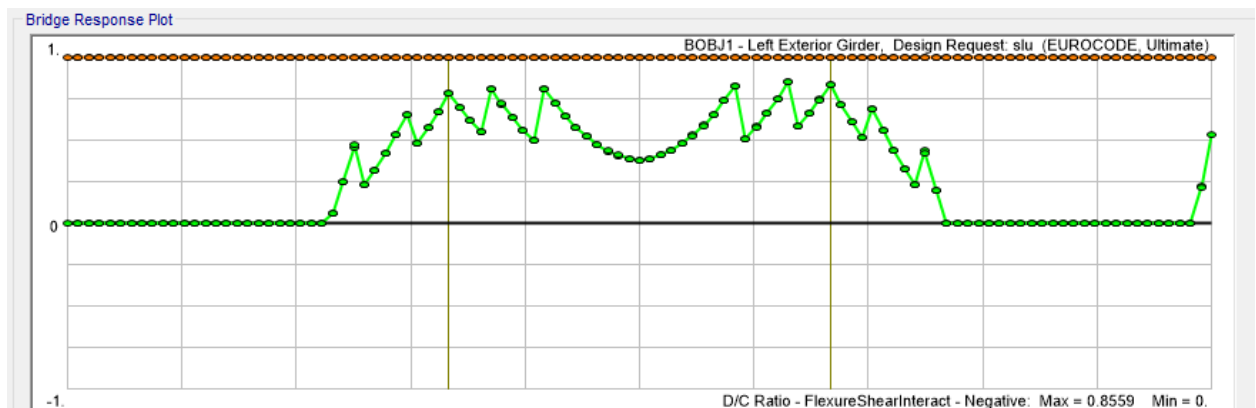
Figura 6.18 -. Verifica interazione taglio/momento negativo
