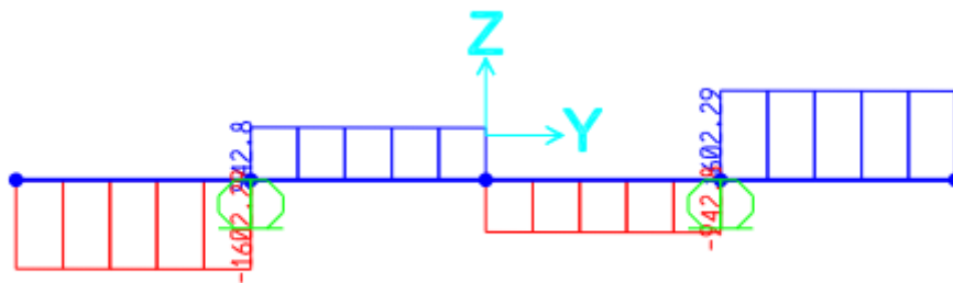
Figura 8.4 -. Momento flettente (kN*m)
