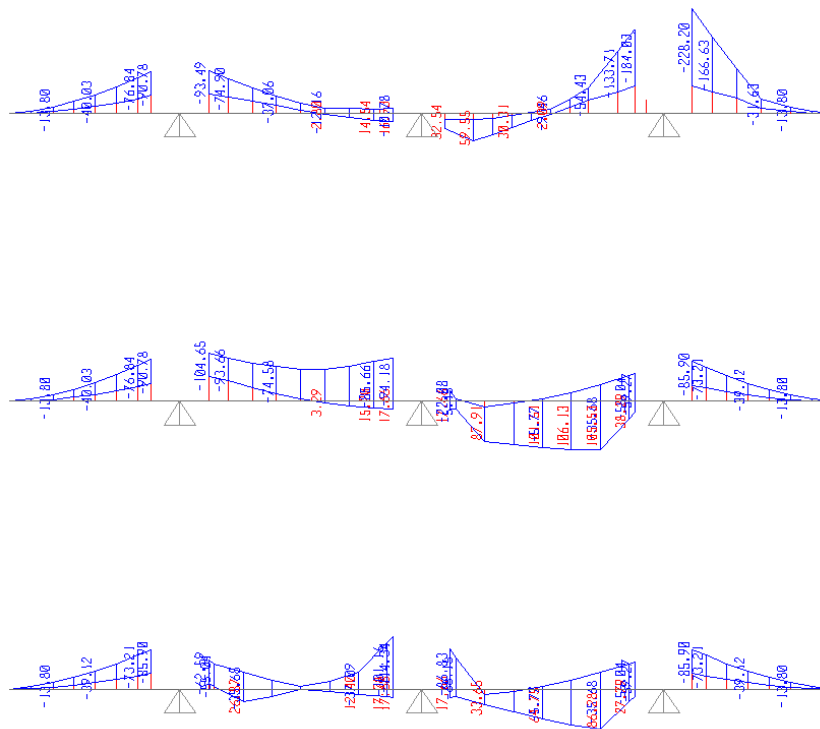
Figura 8.19 - involuppo momento flettente SLU
