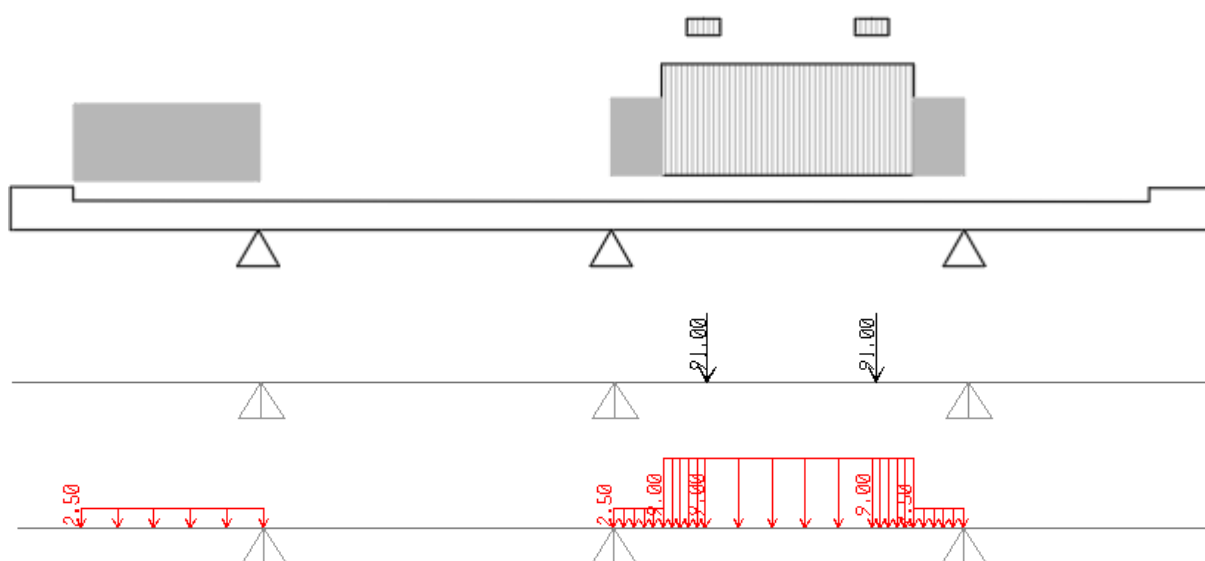
Figura 8.17 -. Condizione di carico 2
