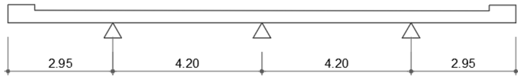
Figura 8.9 - Schema statico
