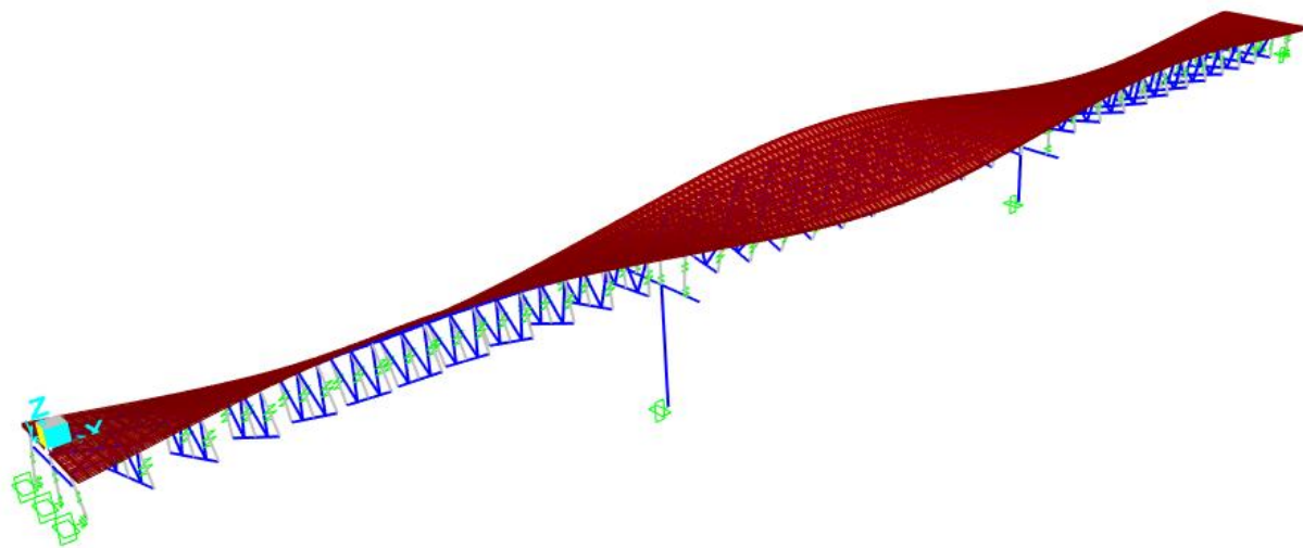
Figura 6.2 - Modo 2
