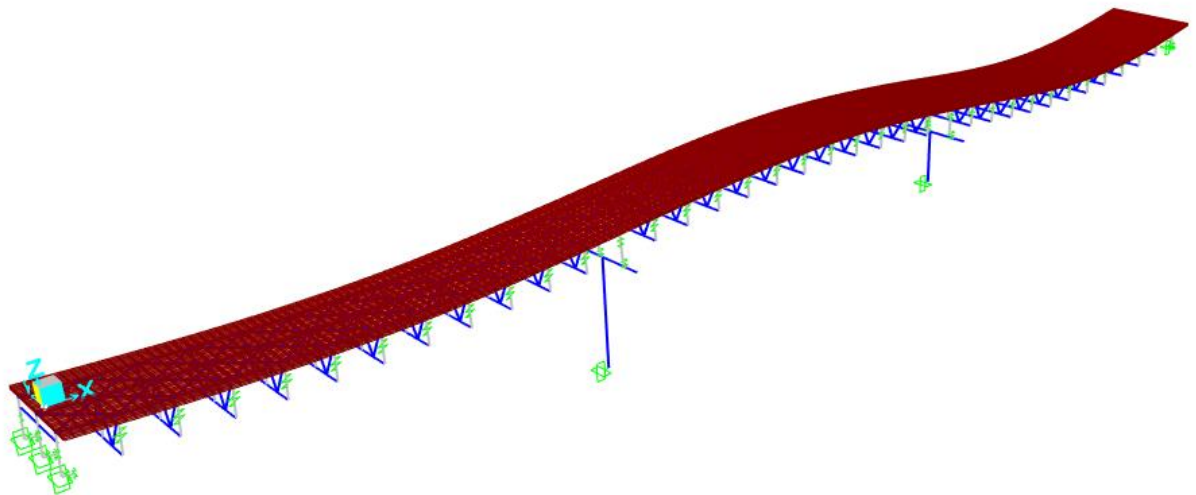
Figura 6.1 - Modo 1
