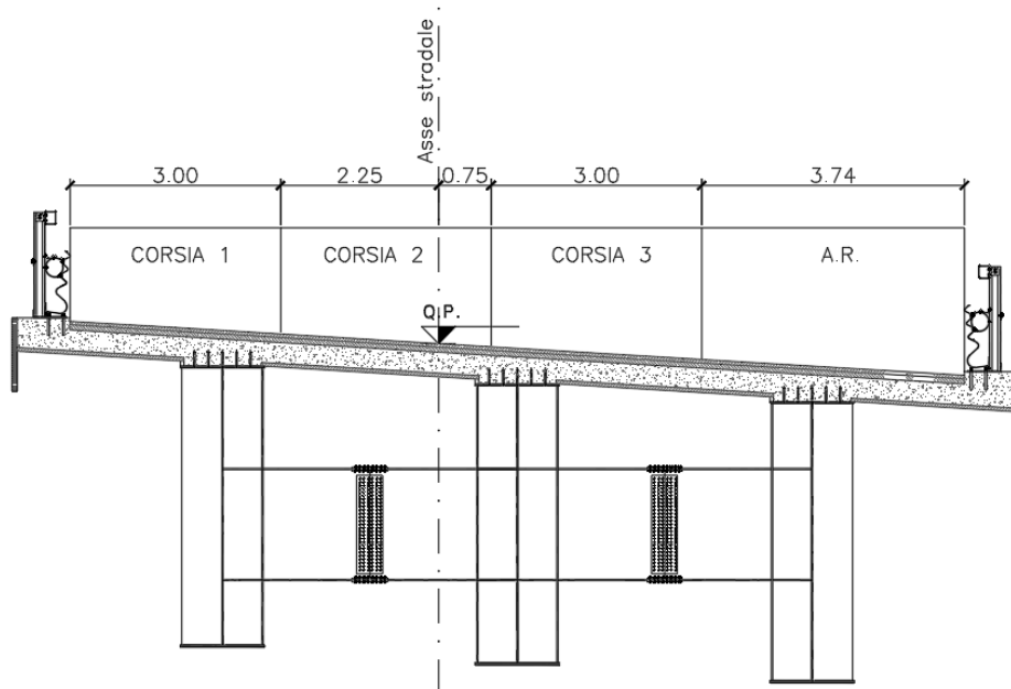
Figura 5.5: Schema di carico
