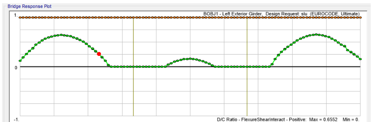
Figura 6.17 -. Verifica interazione taglio/momento positivo
