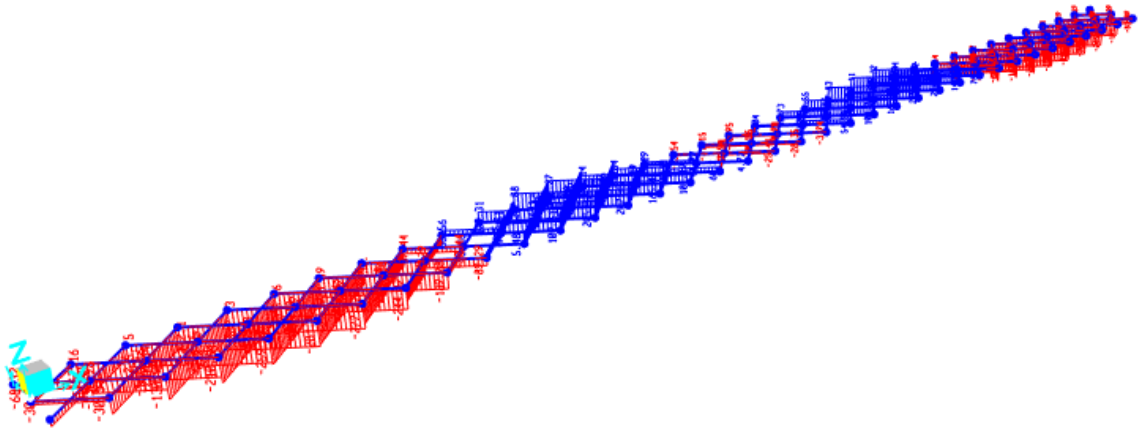
Figura 8.8 -. Sforzo Normale (kN)
