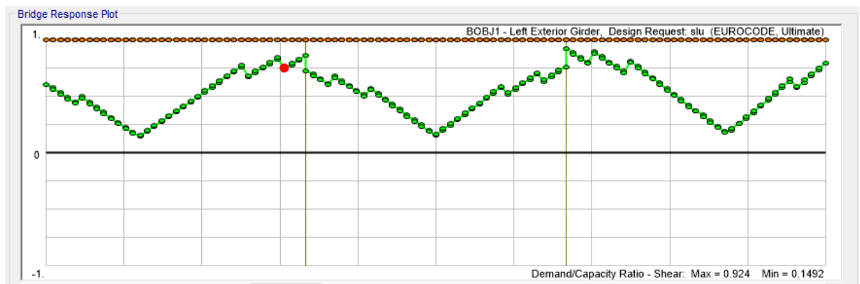
Figura 6.16 -. Verifica taglio
