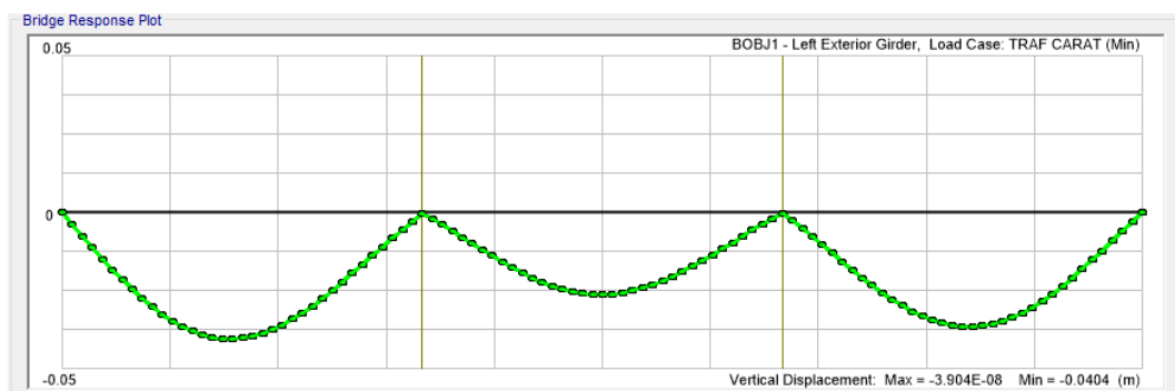
Figura 7.7 -. Abbassamento traffico 0.04m
