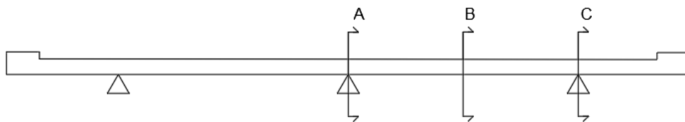
Figura 8.15 - sezioni di interesse per la massimizzazione delle sollecitazioni
