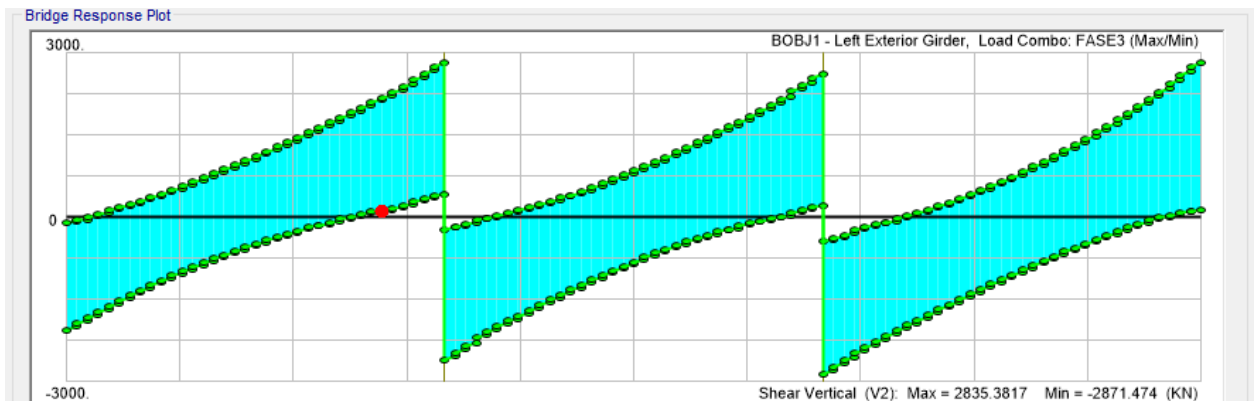
Figura 6.12 -. Taglio (kN)
