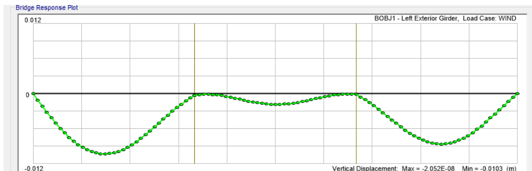
Figura 7.8 -. Abbassamento vento 0.001m
