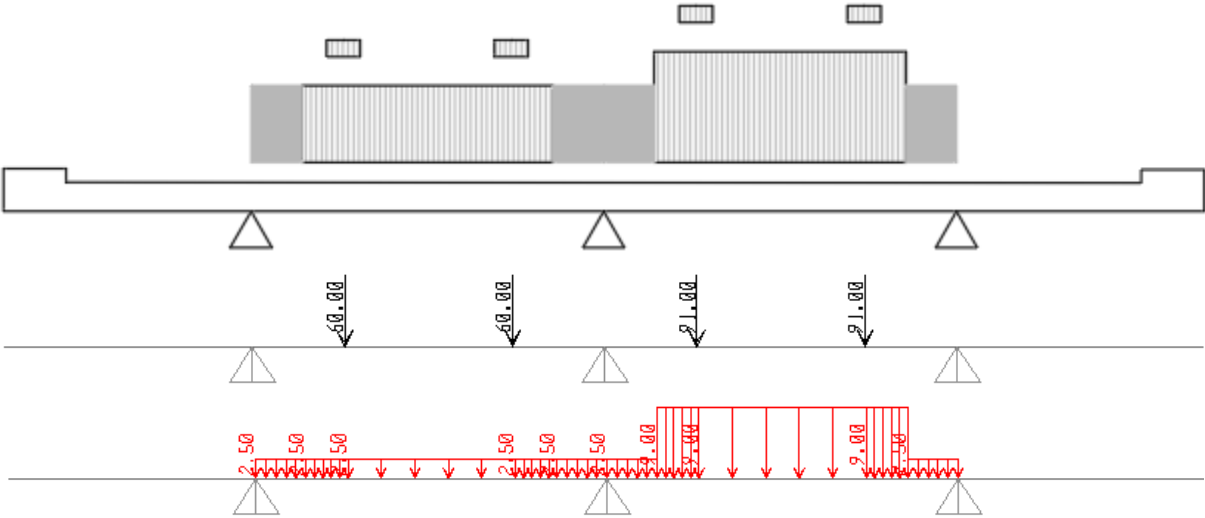
Figura 8.18 -. Condizione di carico 3
