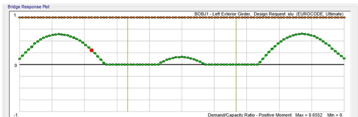
Figura 6.14 -. Verifica momento positivo
