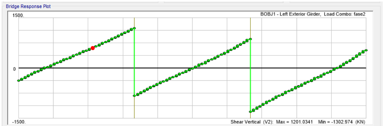
Figura 6.9 -. Taglio (kN)
