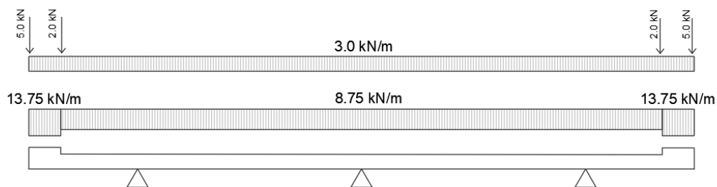
Figura 8.10 - Carichi permanenti
