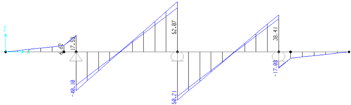
Figura 8.28 -diagramma taglio FASE 2
