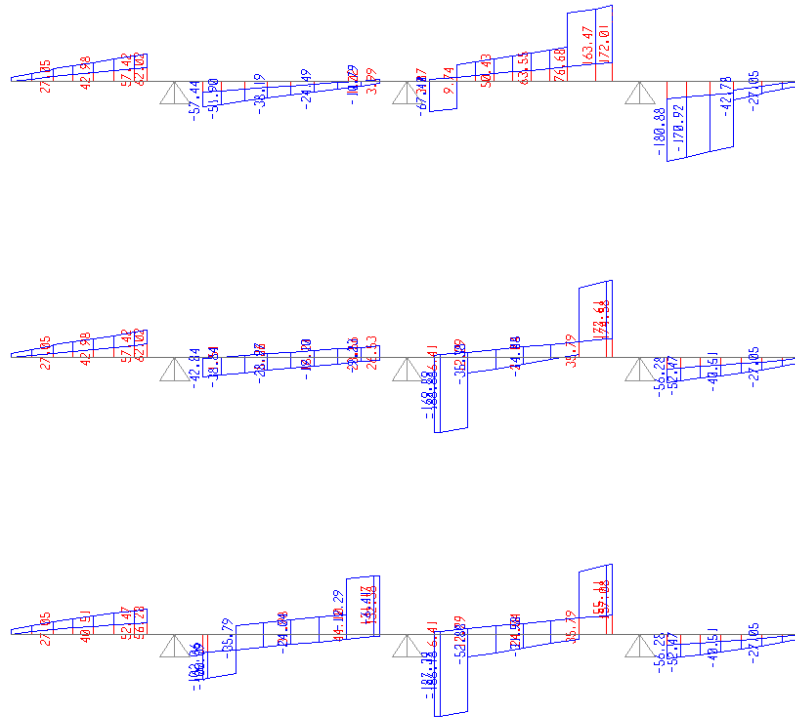
Figura 8.20 - involucro taglio SLU
