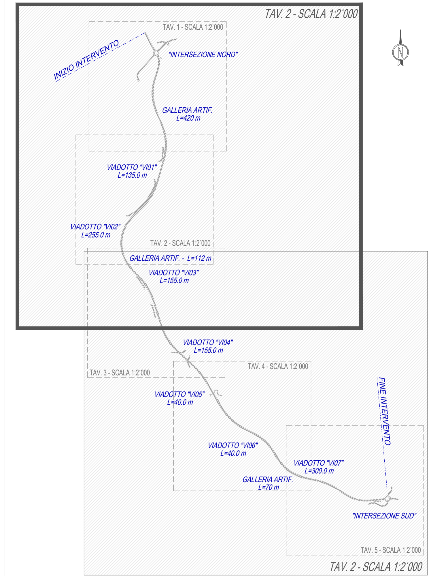
QUADRO DI UNIONE 1:5.000
