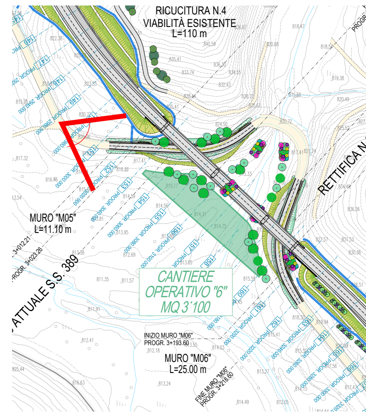
Viadotto V104
