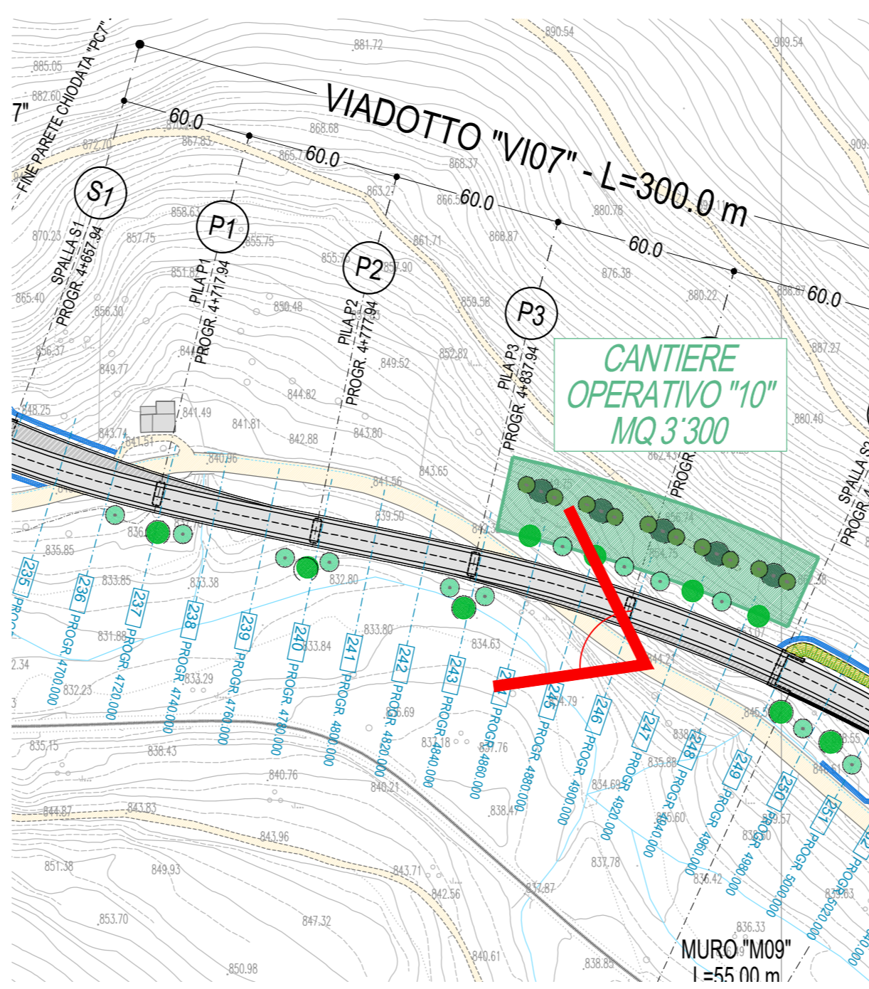
Viadotto V107
