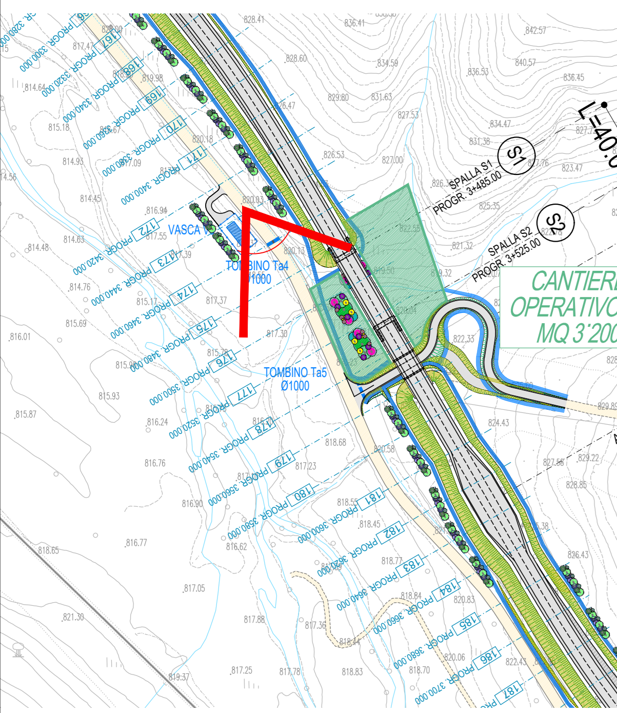
Viadotto V105
