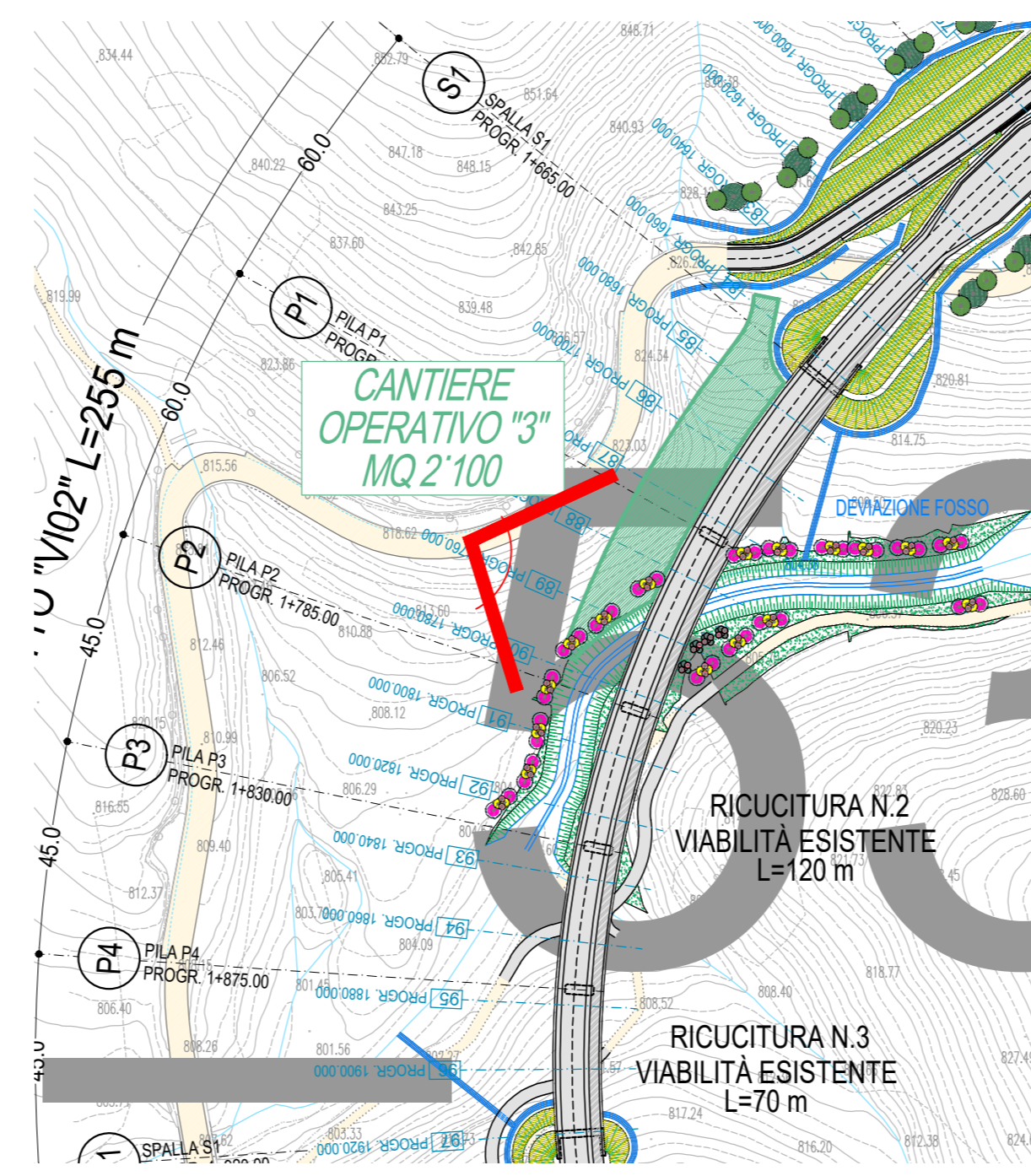
Viadotto V102
