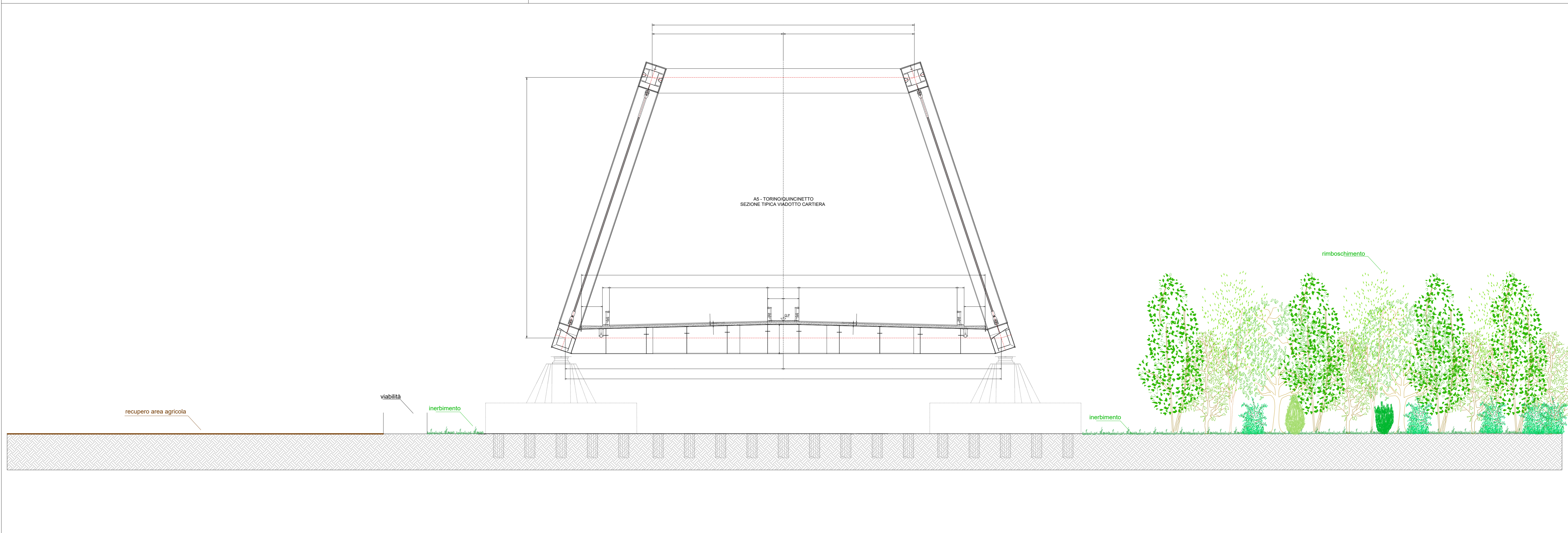
SEZIONE TIPOLOGICA C - OPERE A VERDE VIADOTTO CARTIERA - scala 1:200
