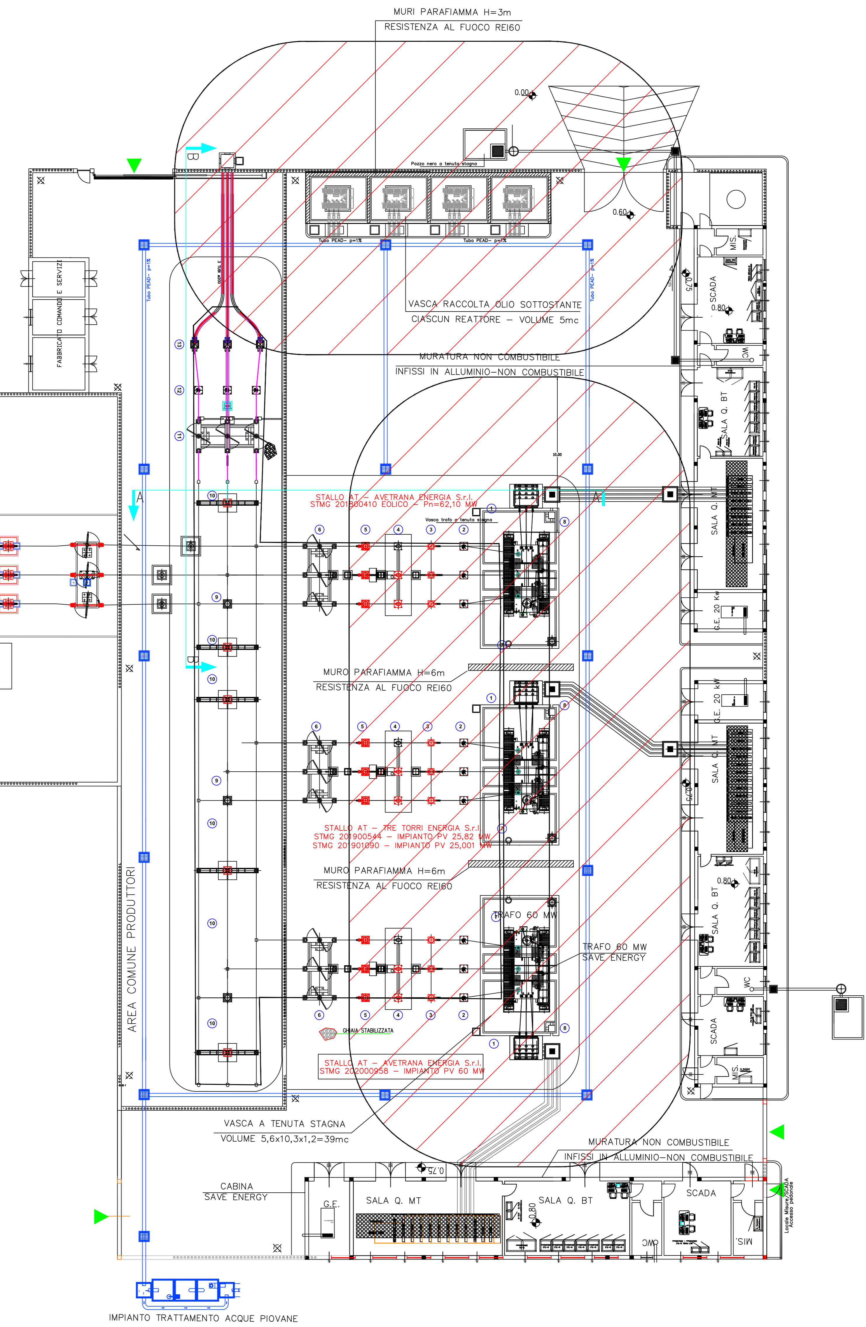
DISTANZE DI SICUREZZA INTERNA ALLA CABINA (Capo 1 art.2.2 Tab. 2 – DM 15 luglio 2014)
