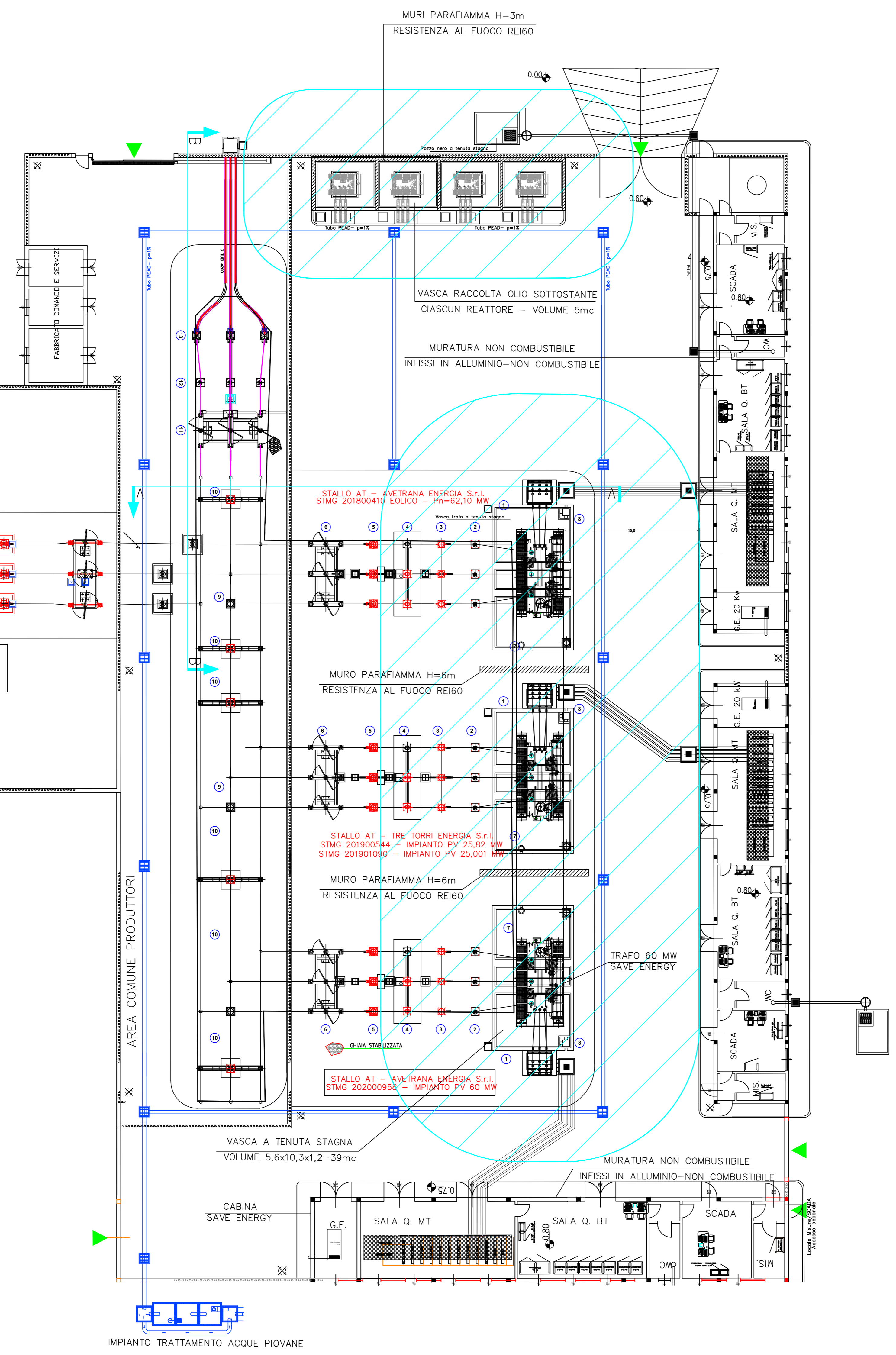
DISTANZE DI SICUREZZA INTERNA ALLA CABINA (Capo 1 art.2.1 Tab. 1 – DM 15 luglio 2014)
