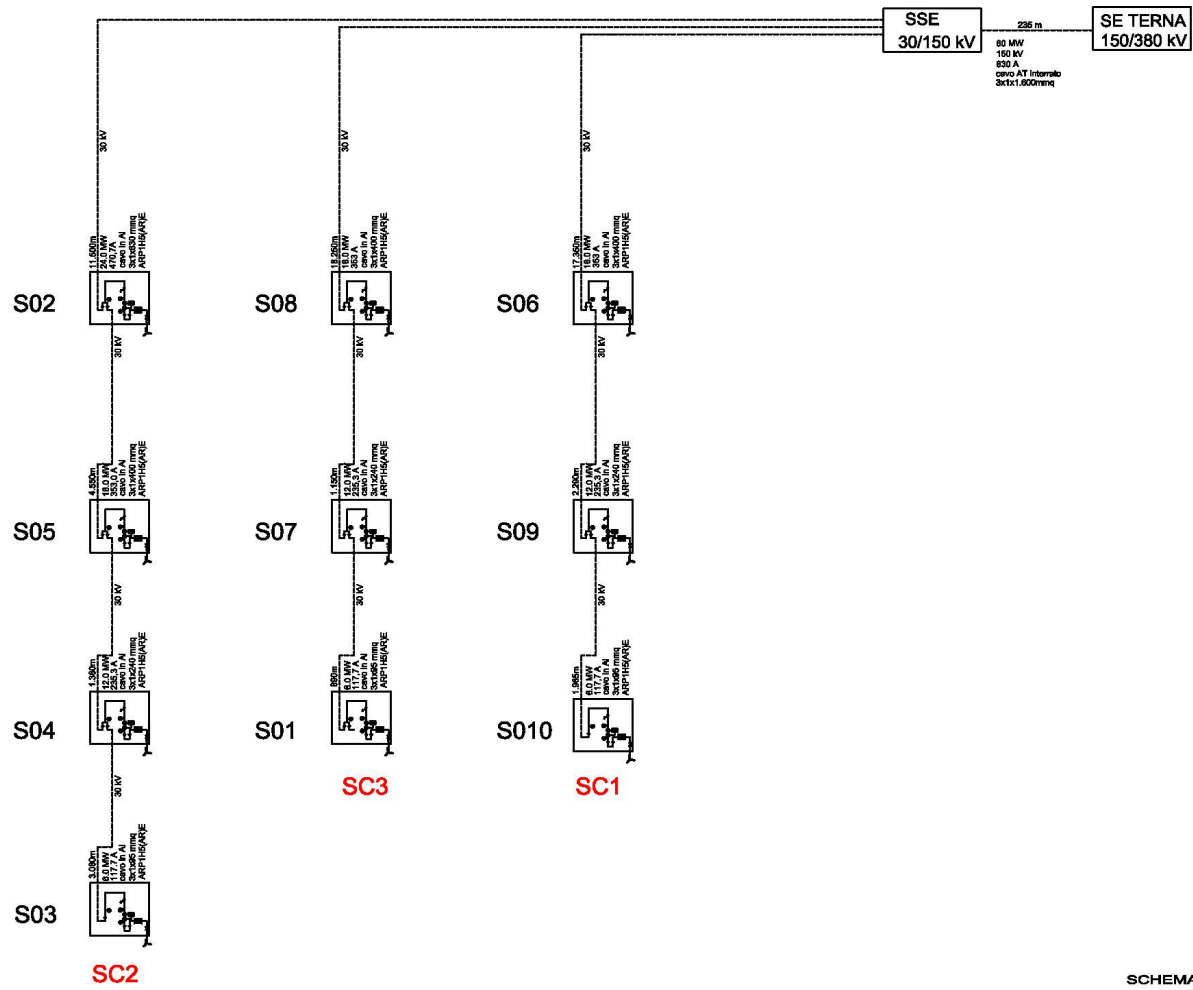
SCHEMA A BLOCCHI RETE MT PARCO EOLICO
