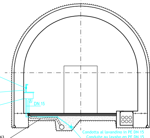
GALLERIA DI COLLEGAMENTO SEZIONE A-A 1:50 GALLERIE DE LIAISON COUPE A-A 1:50
