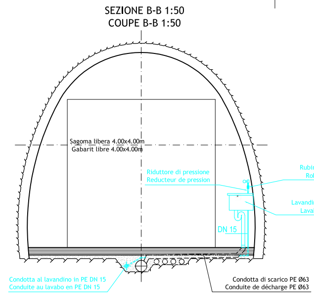
SEZIONE B-B 1:50 COUPE B-B 1:50
