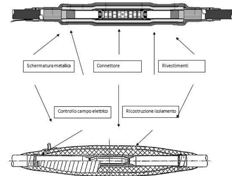
Figura 10: Principali elementi costituenti una giunzione
