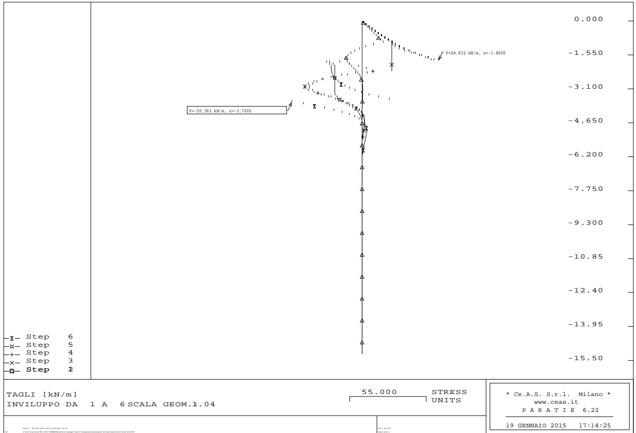
Figura 25 - Condizioni statiche - Inviluppo del taglio
