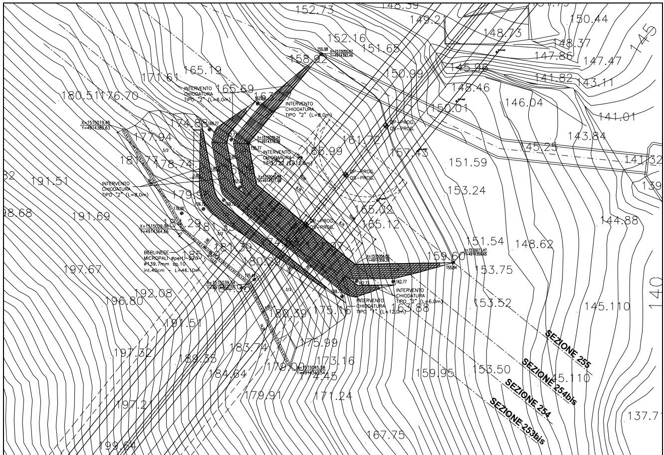
Figura 2: Disposizione planimetrica delle opere di imbocco
