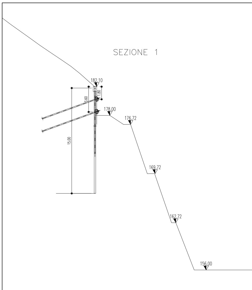
Figura 6: Sezione di calcolo
