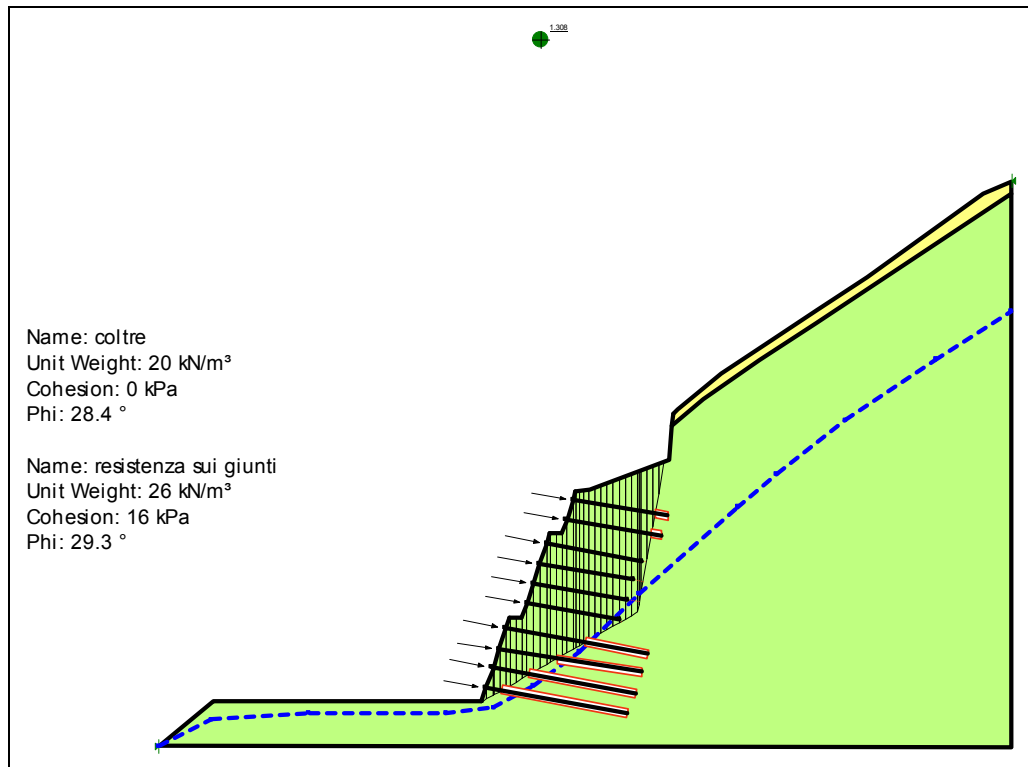
Figura 30: Risultati analisi di stabilità scavi con barre in acciaio - Condizioni statiche
