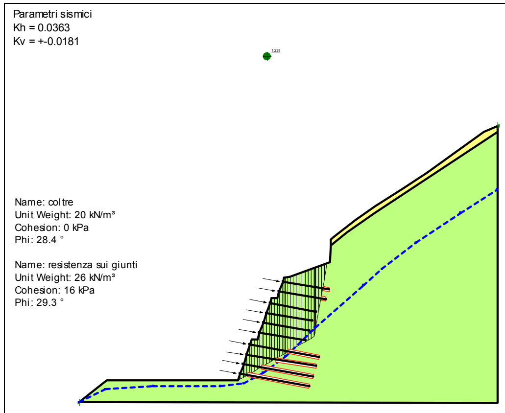
Figura 32: Risultati analisi di stabilità scavi con barre in acciaio - Condizioni sismiche
