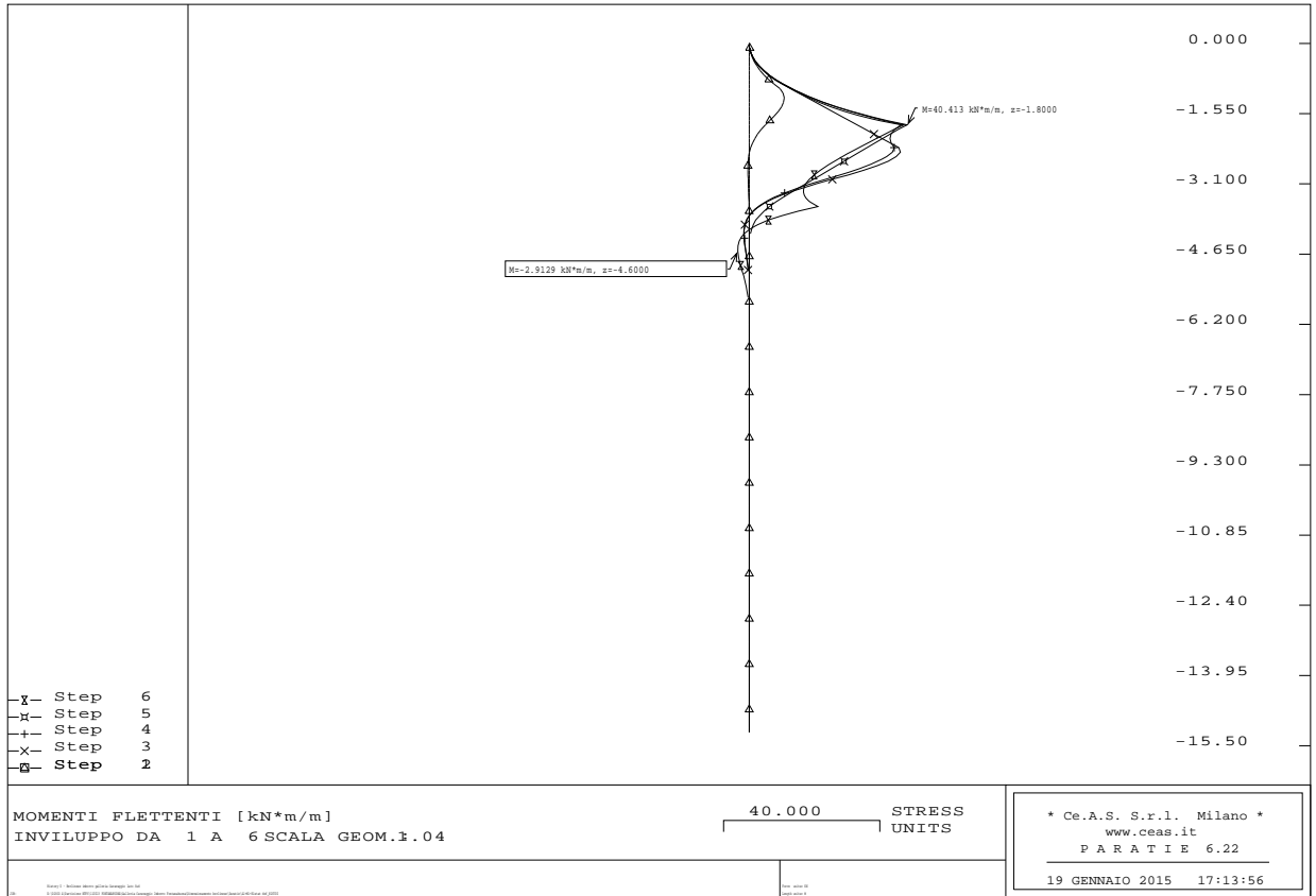
Figura 24 - Condizioni statiche - Inviluppo del momento flettente
