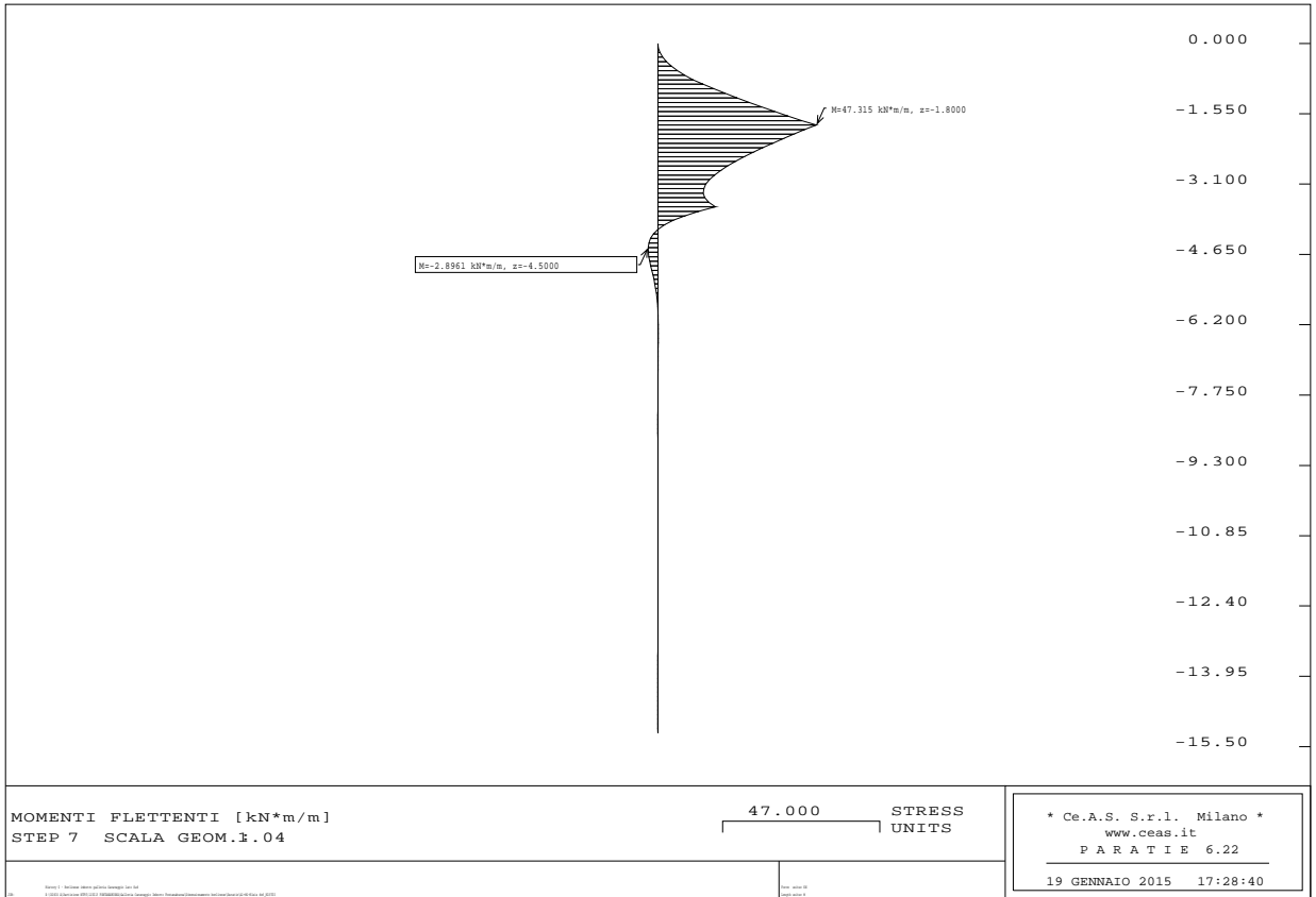
Figura 27: Programma Paratie - Diagramma del momento flettente - condizioni sismiche
