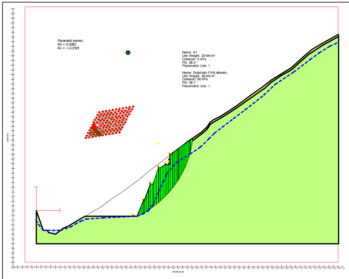
Figura 26 - Verifica di stabilità globale in campo sismico
