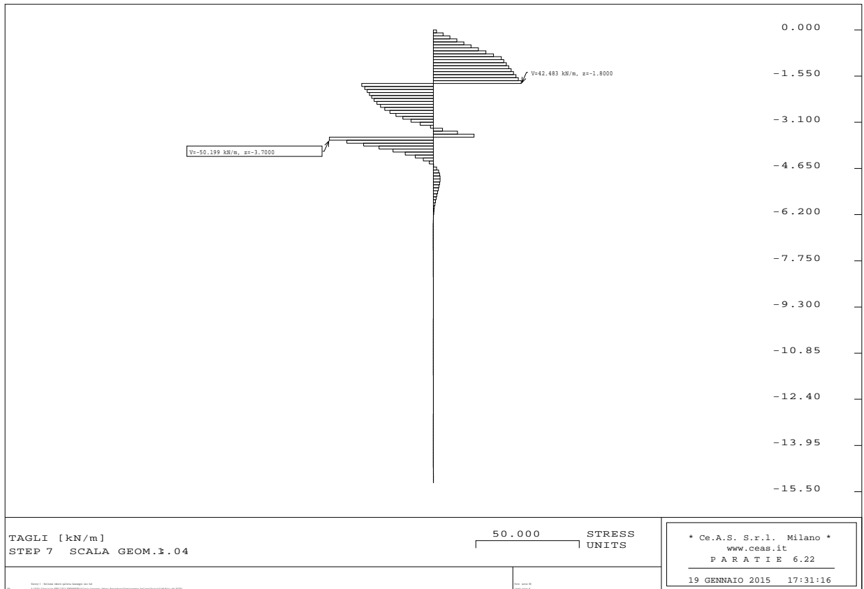
Figura 28: Programma Paratie - Diagramma del taglio - condizioni sismiche
