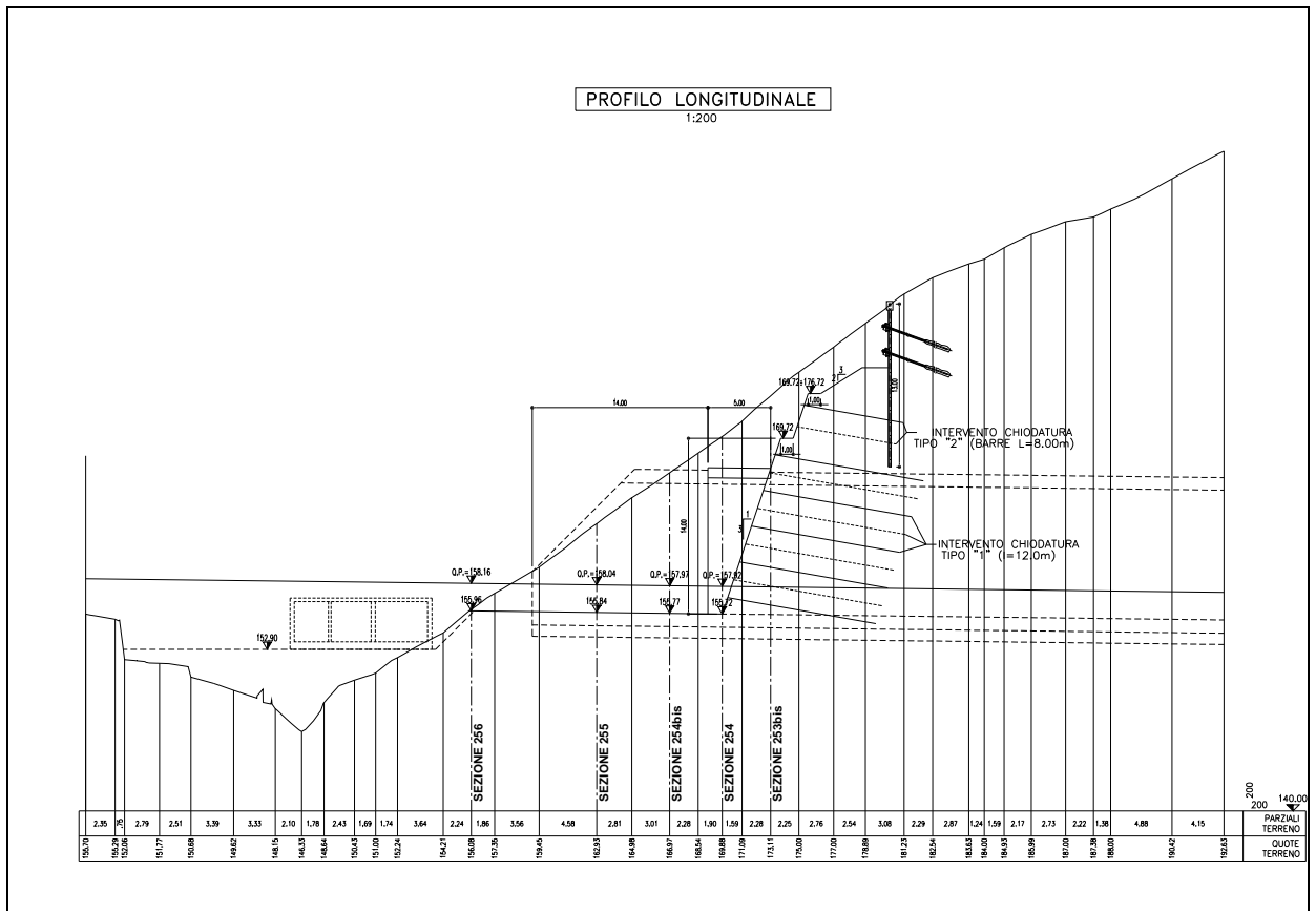
Figura 17: Sezione di calcolo chiodature in VTR
