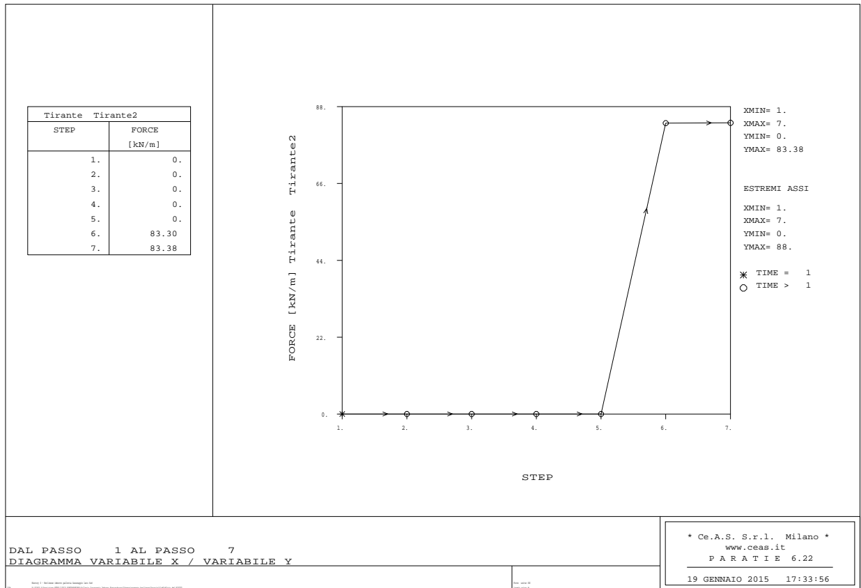
Figura 23 - Programma Paratie - Tiro 2° ordine tiranti
