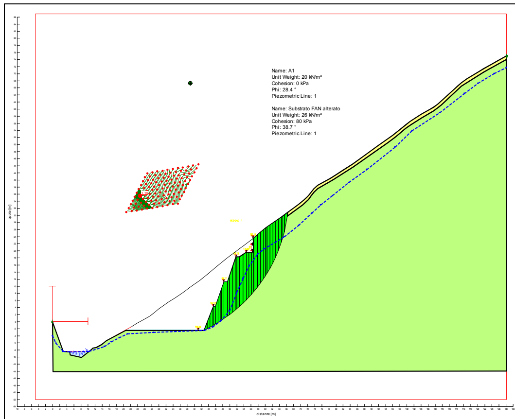
Figura 21: Verifica di stabilità globale in campo statico
