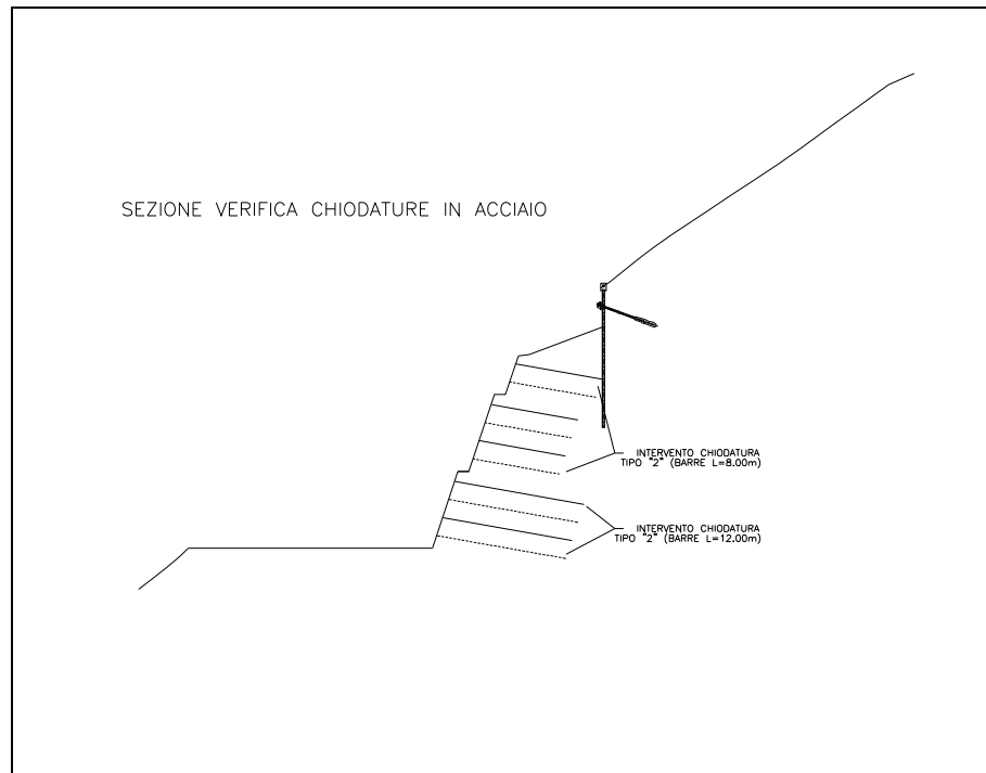
Figura 16: Sezione di calcolo chiodature in acciaio
