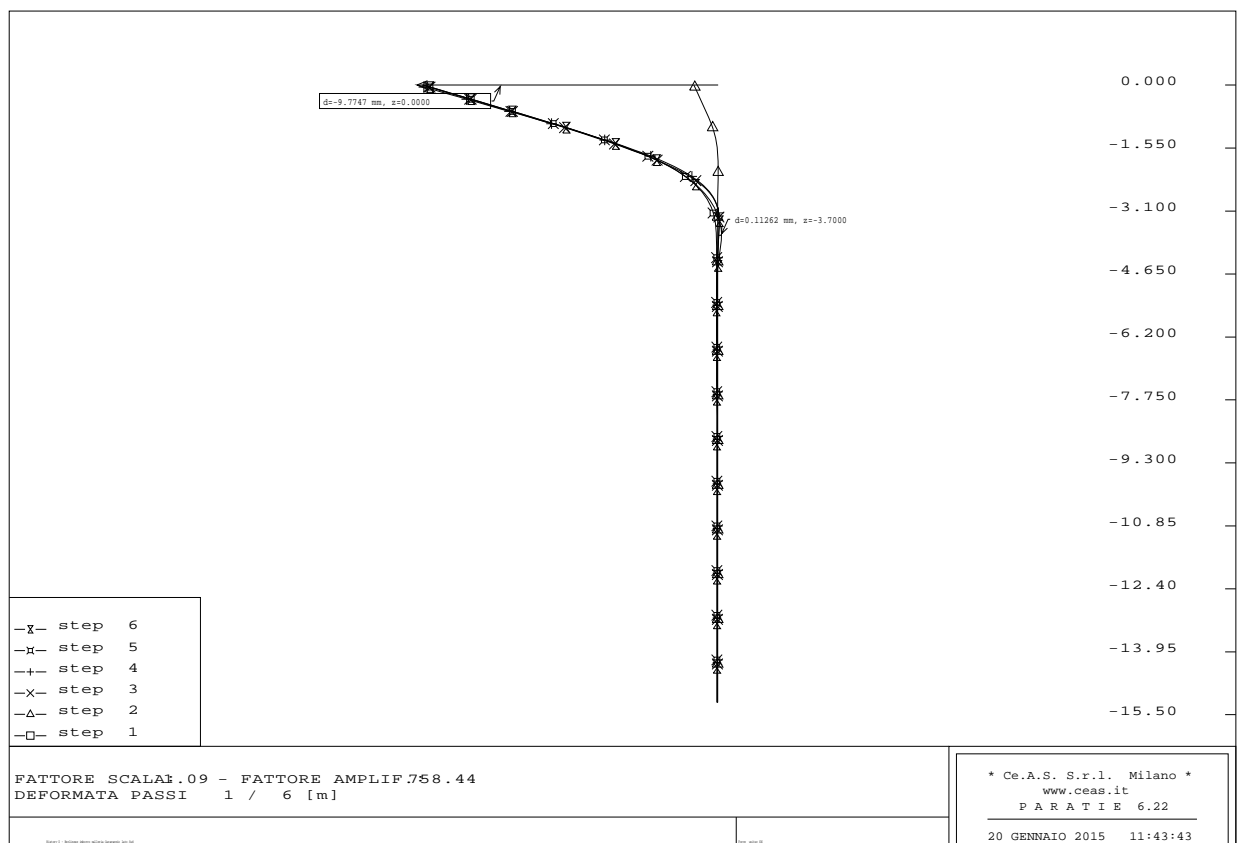
Figura 29: Programma Paratie - Inviluppo degli spostamenti lungo la paratia (SLE)
