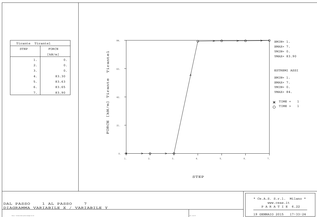
Figura 22 - Programma Paratie - Tiro 1° ordine tiranti
