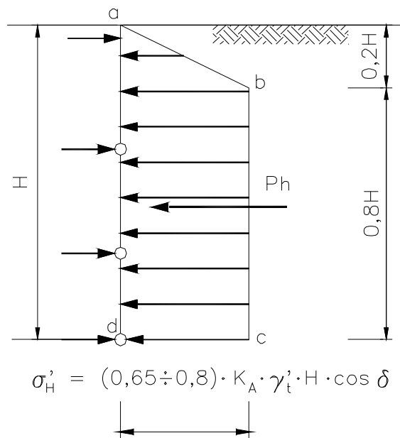
Figura 39: Spinta delle terre in condizioni drenate agente su pareti di sostegno multiancorate in terreni privi di coesione
