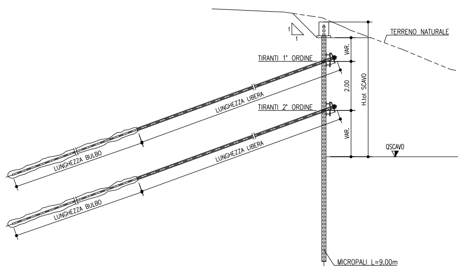
Figura 18: Sezione di calcolo 1
