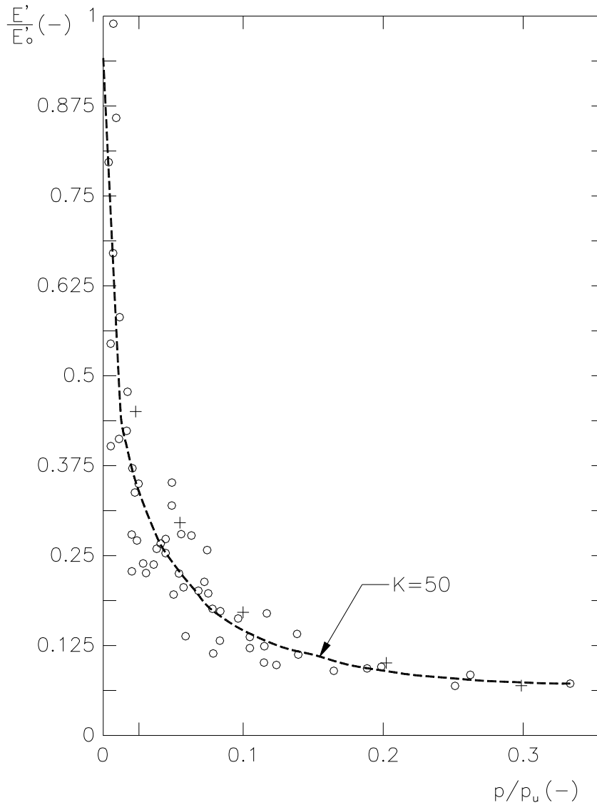
Figura 35: Variazione del modulo di elasticità in funzione del grado mobilitazione: sabbie e ghiaie sovraconsolidate
