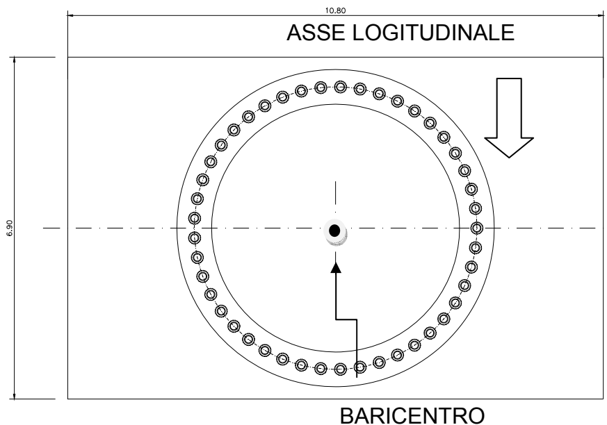
Figura 2: Pile Vtto TONGUSCI - Sistema di riferimento strutturale
