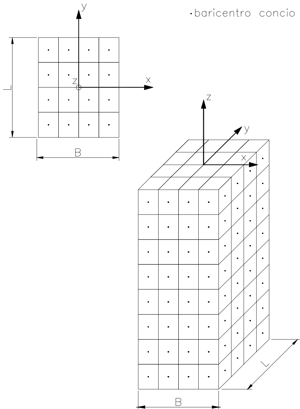
Figura 34: Schema di suddivisione in conci del pozzo
