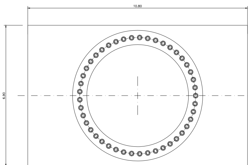
Figura 12: Pianta delle fondazioni
