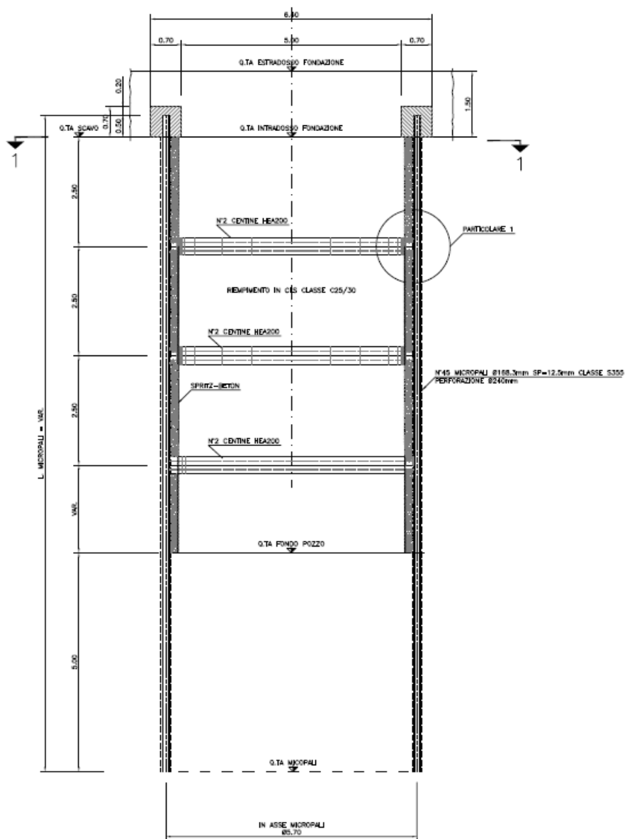
Figura 4: Sezione tipo del pozzo
