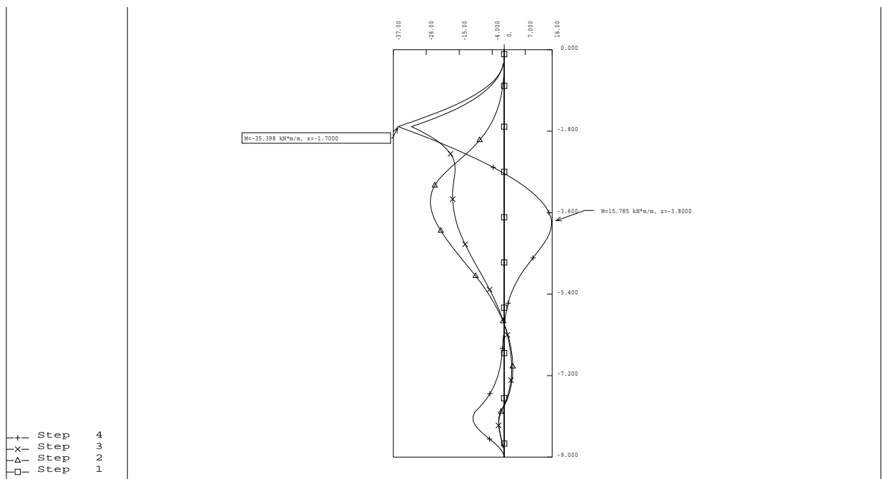
Figura 23: Paratia Sezione 2– Momento Flettente
