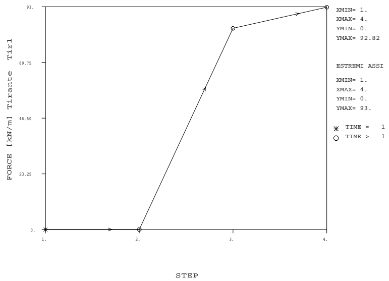
Figura 29: Sezione 2 tirante 1 Combinazione A1+M1
