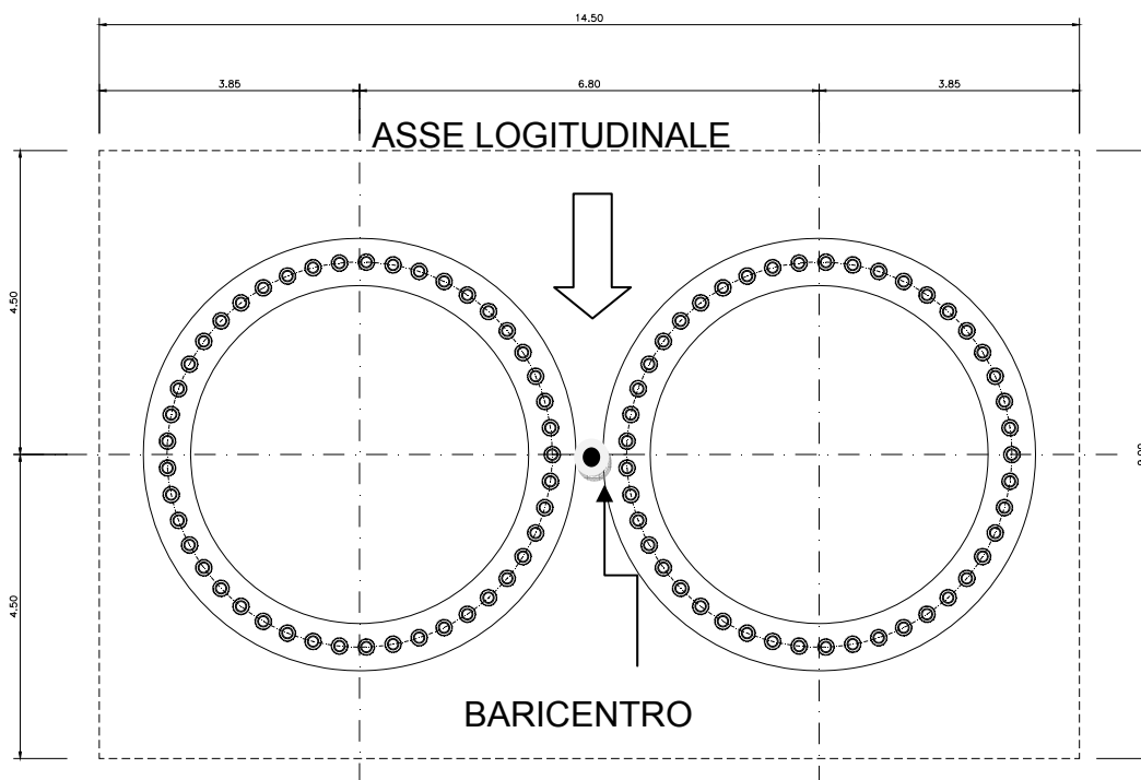
Figura 2: Pile Vtto TONGUSCI - Sistema di riferimento strutturale
