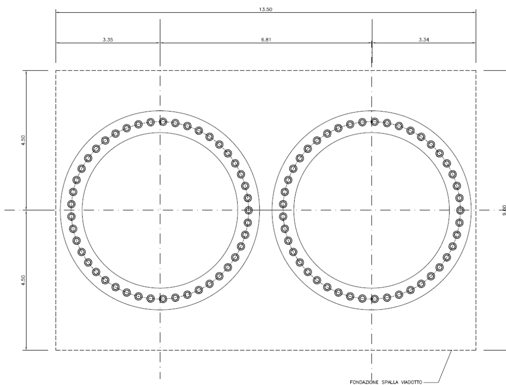
Figura 6: Pianta delle fondazioni
