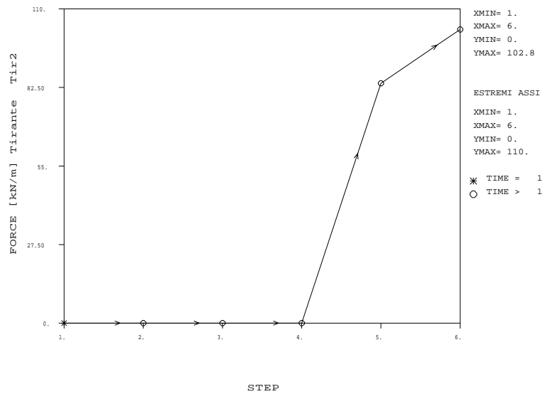
Figura 28: Sezione 1 tirante 2 Combinazione A1+M1
