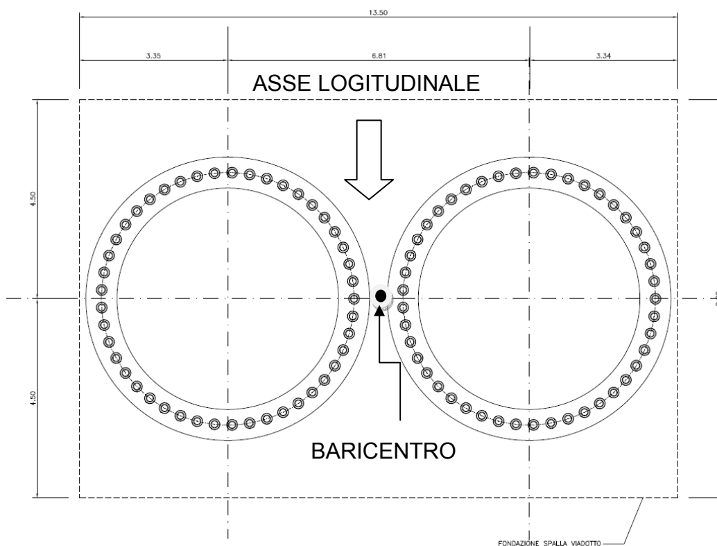
Figura 1: Spalla A Vtto TONGUSCI - Sistema di riferimento strutturale
