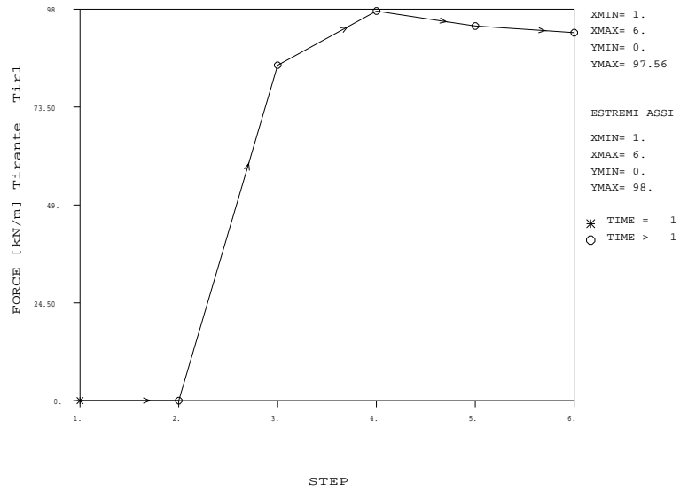
Figura 27: Sezione 1 tirante 1 Combinazione A1+M1
