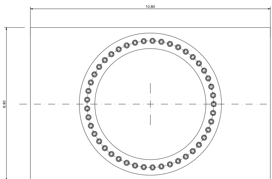
Figura 9: Pianta delle fondazioni
