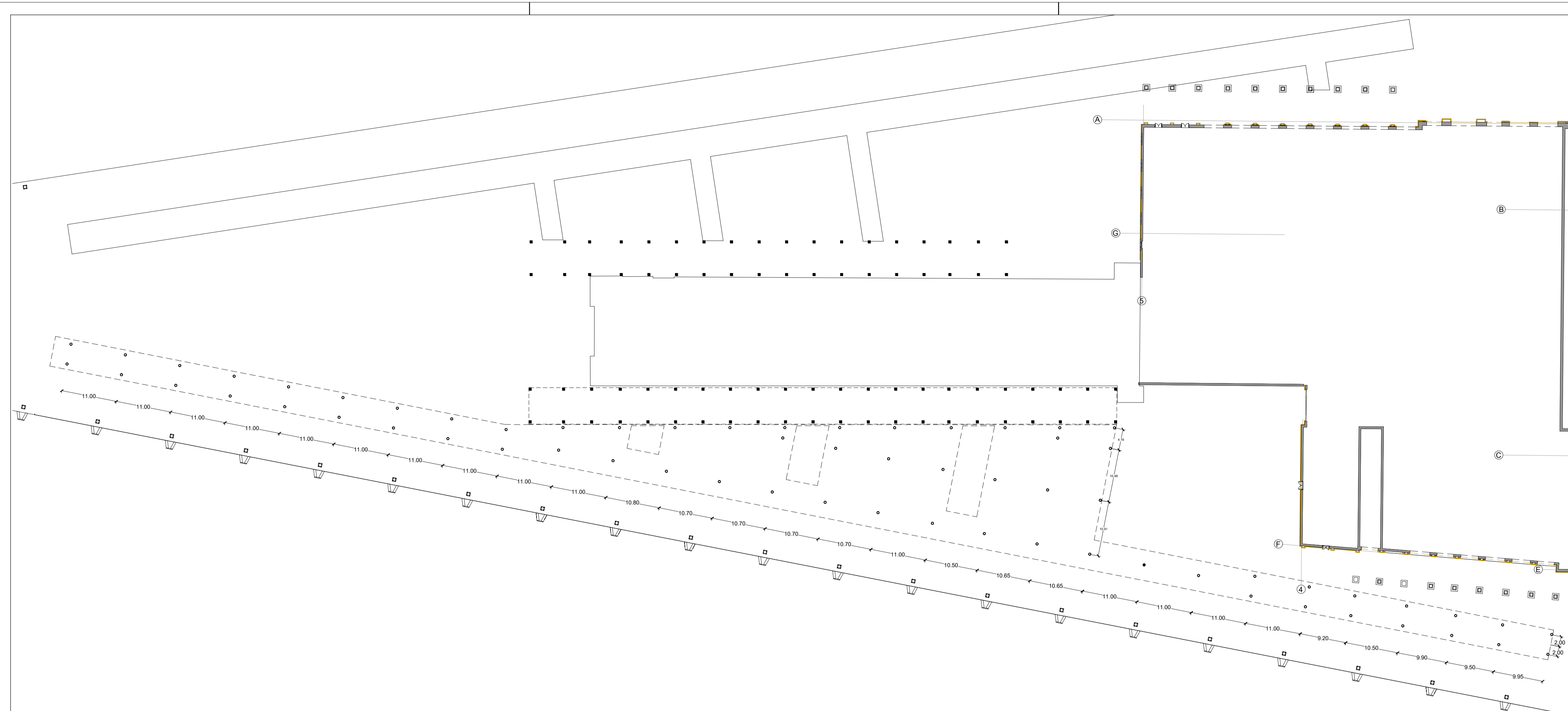
PLANIMETRIA QUOTA BANCHINA scala 1:500
