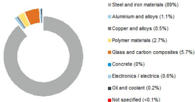
Figura 2 - % in massa composizione turbina V150
