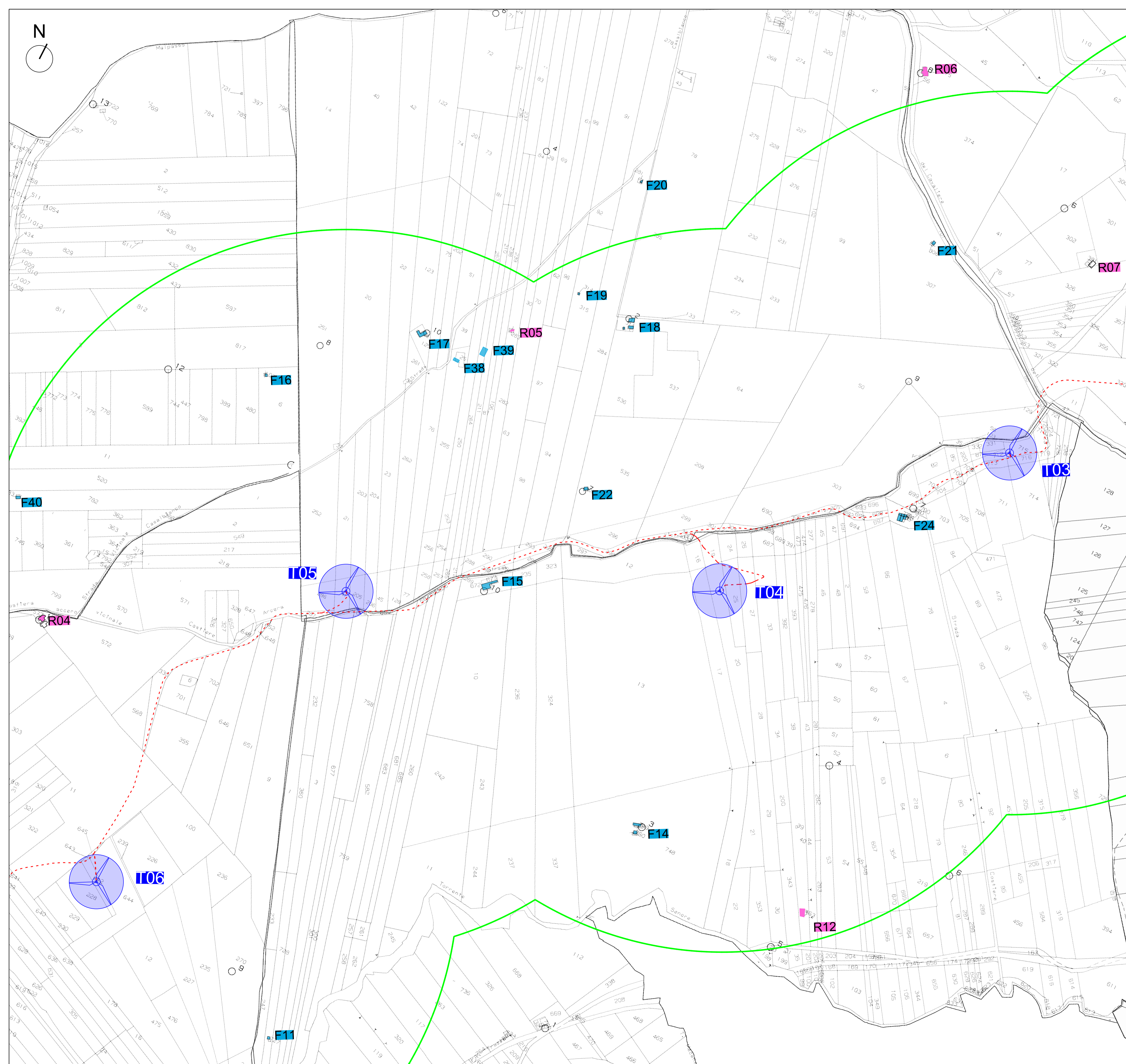
Scala 1:5.000
