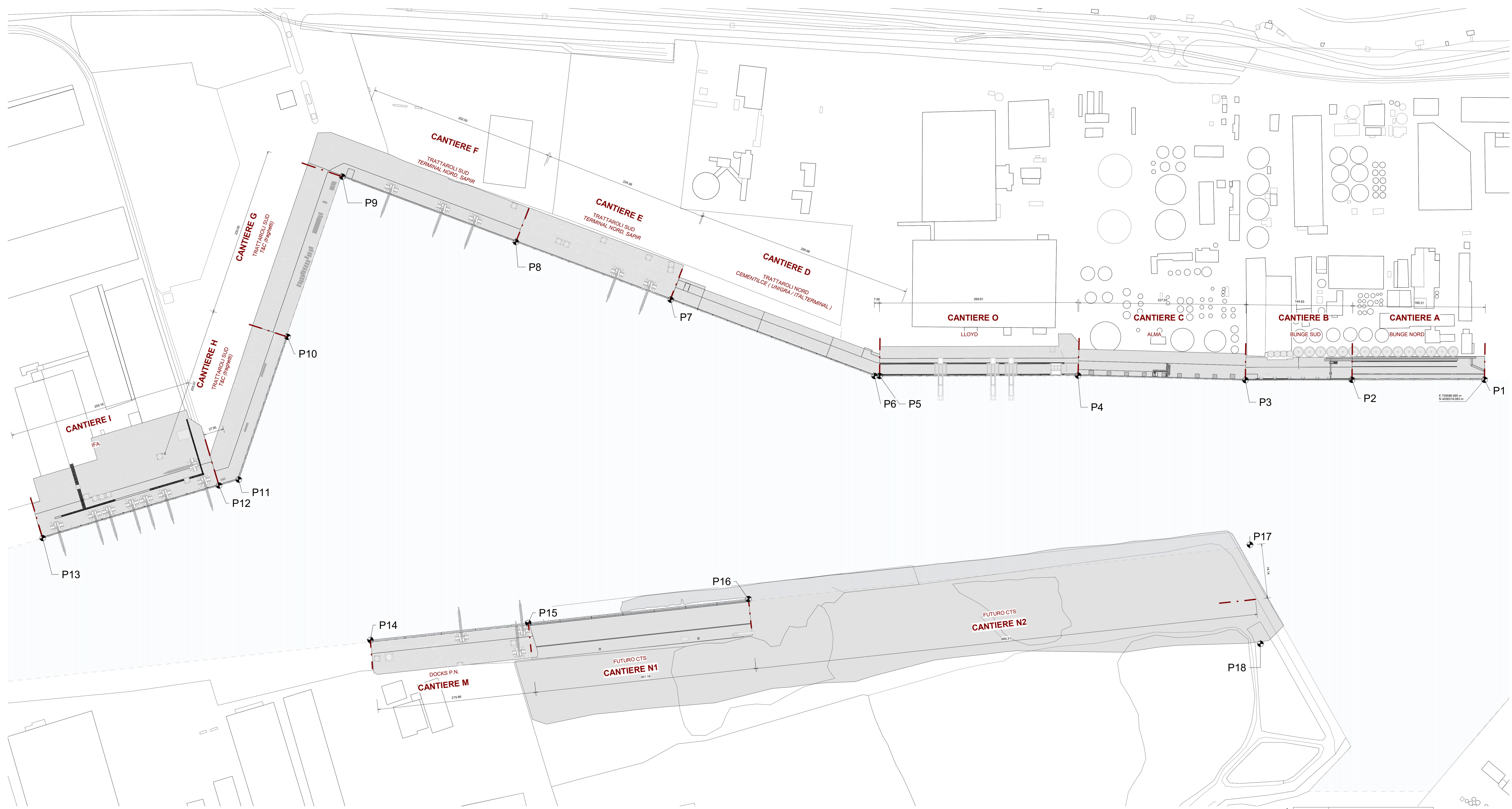
1 Planimetria generale Stato di fatto 1 : 2000
