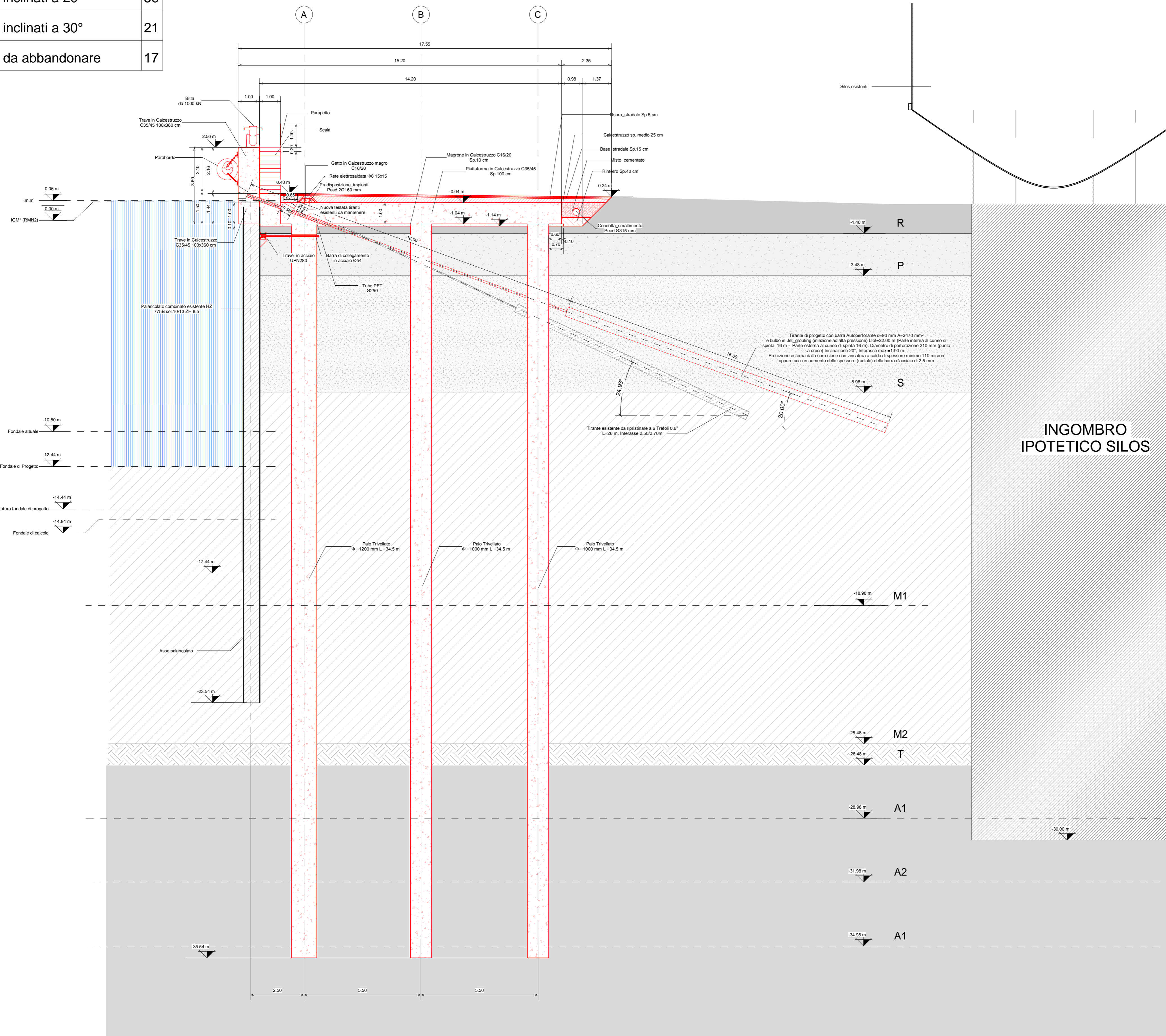
1 Sezione Tipologica 1 : 100
