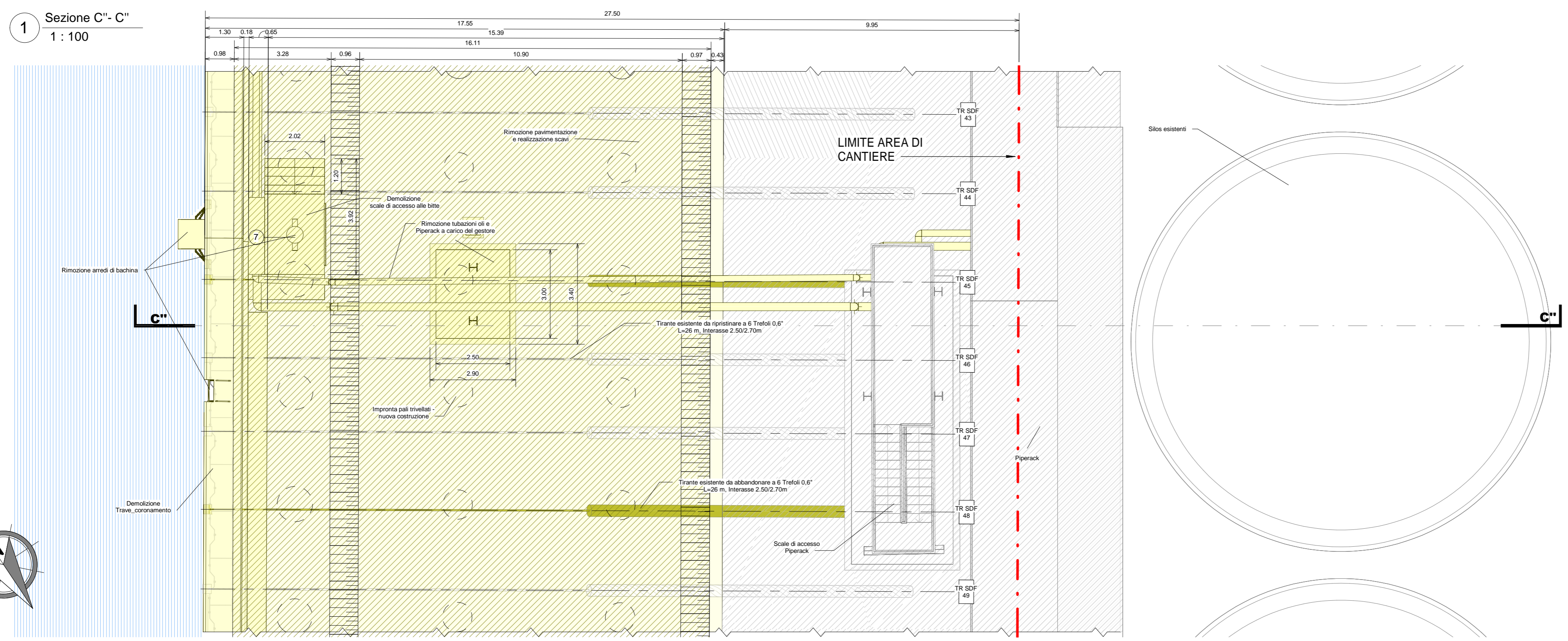
2 Pianta degli scavi e delle demolizioni sezioni tipo 1: 100
