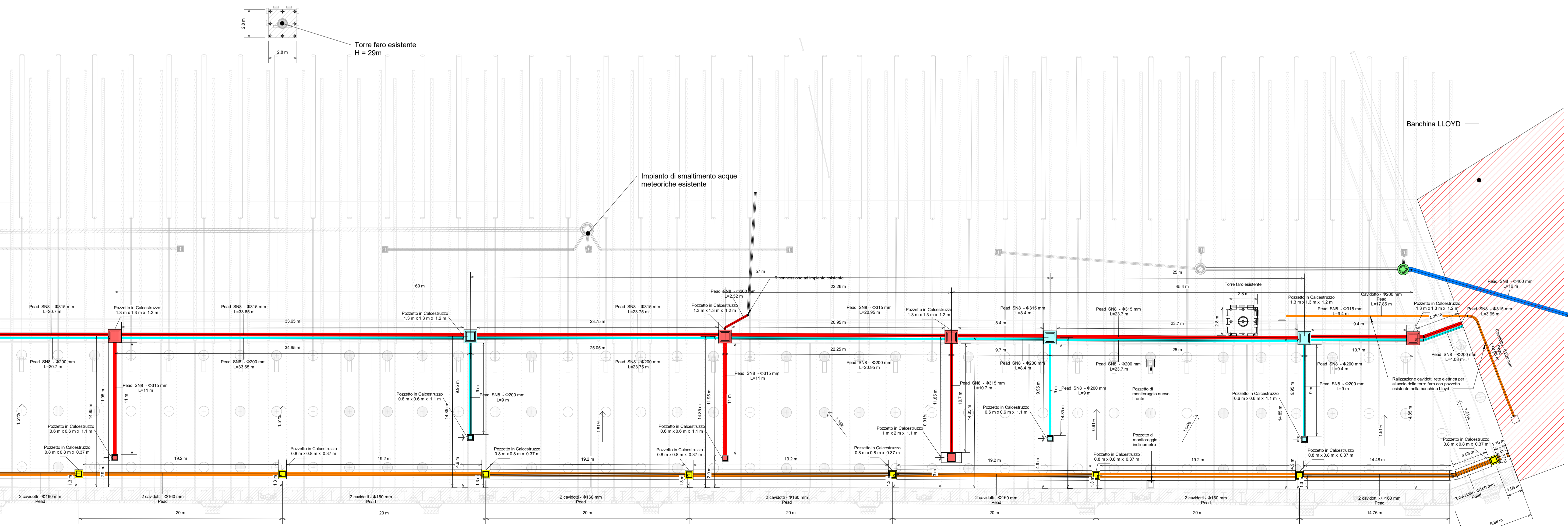
2 Planimetria impianti - Inquadramento 2
