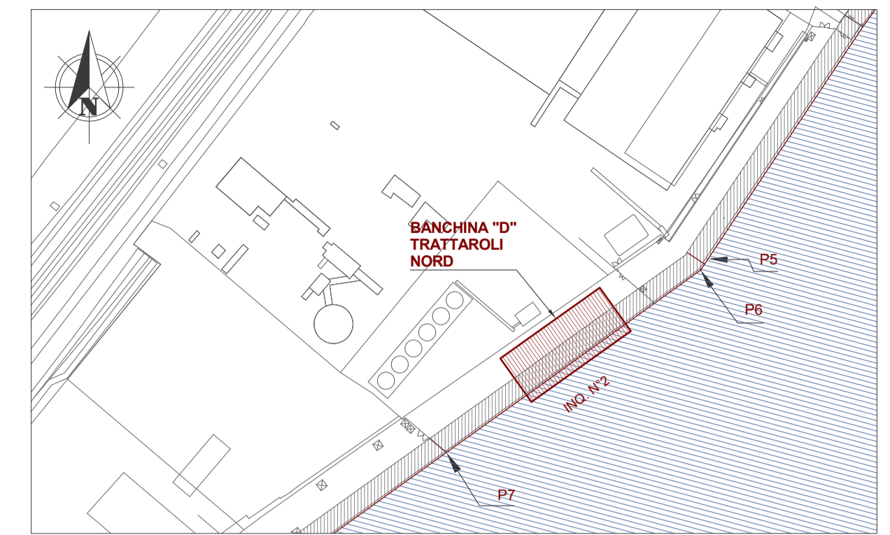
keyplan 1 : 5000
