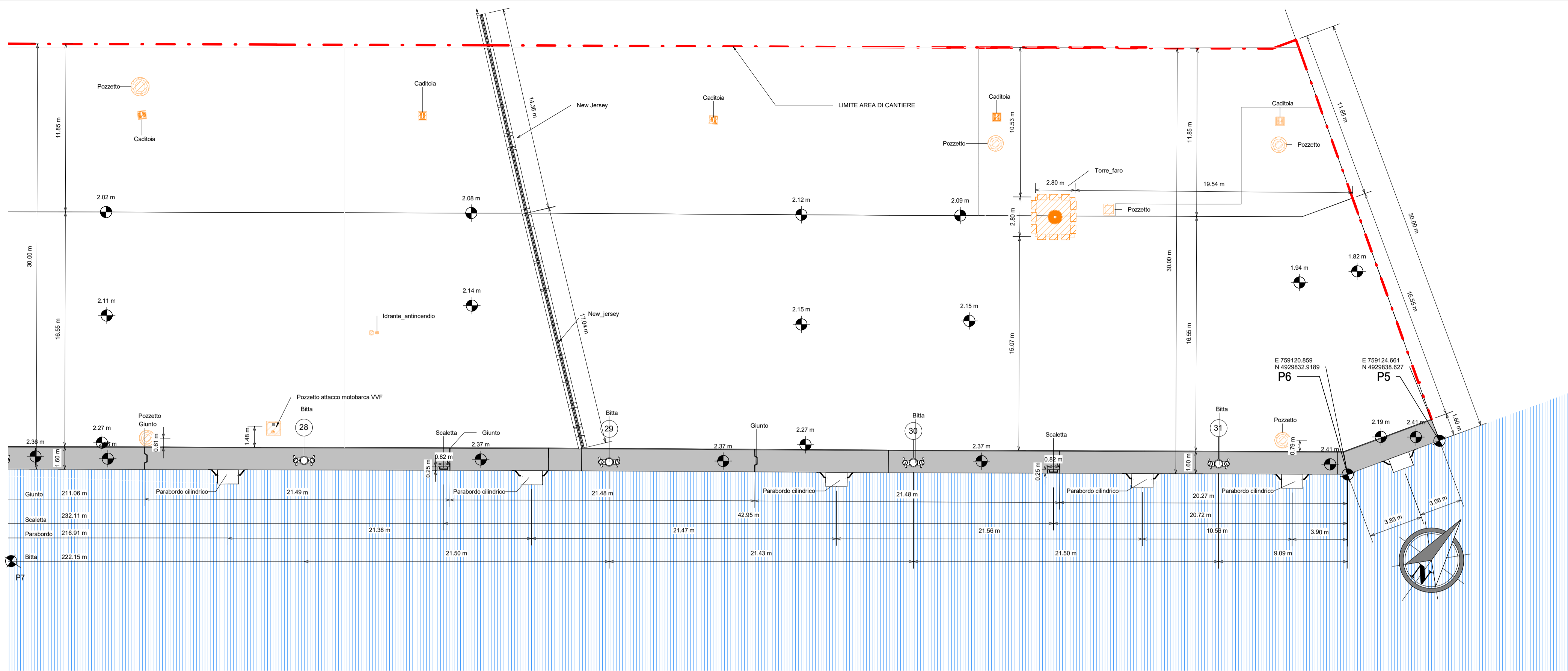
1 Planimetria generale SDF quota piazzale - Inq.3 1 : 200
